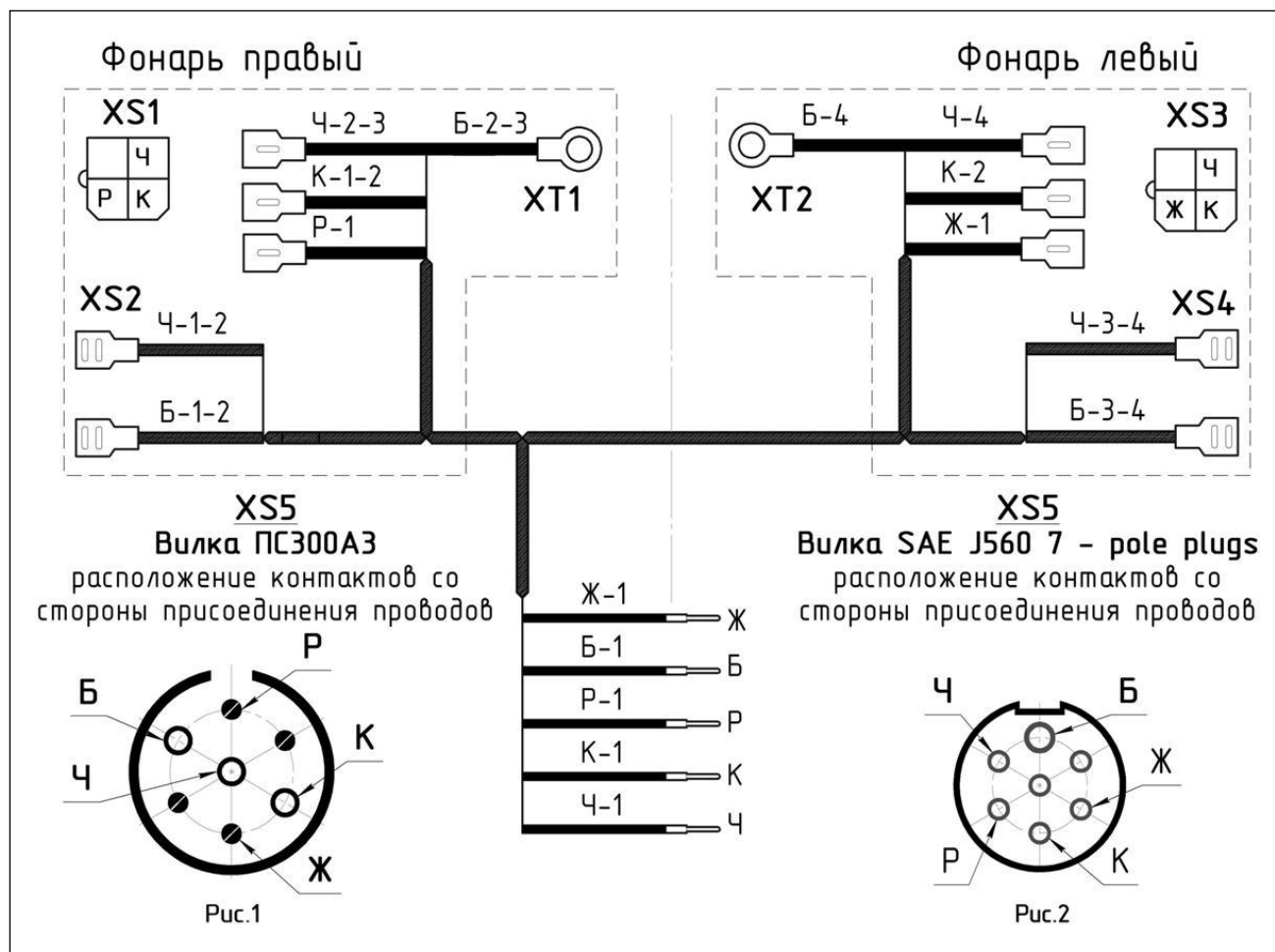
Рисунок Д.1 – Схема электрических коммуникаций культиваторной части
