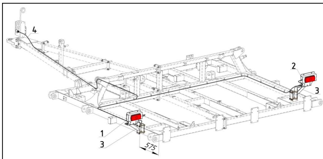
1 – Фонарь левый; 2 – Фонарь правый; 3 – Кронштейн; 4 – Жгут проводки
