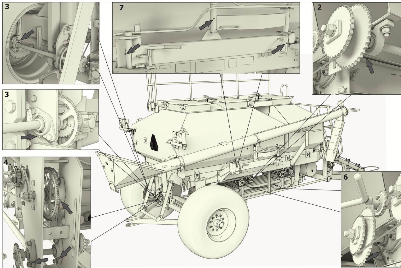
Рисунок 8.3 – Точки смазки бункера АТ-11
