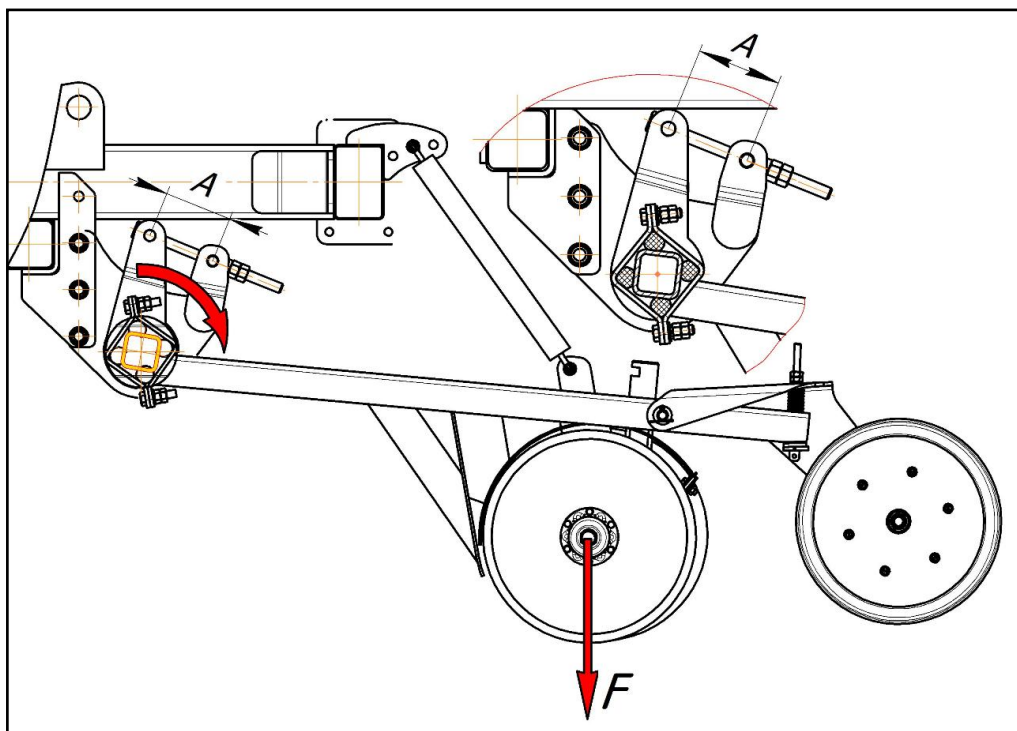
Рисунок 7.4.1 – Схема догрузки дисковых сошников СГ-122.31.800 (900)
