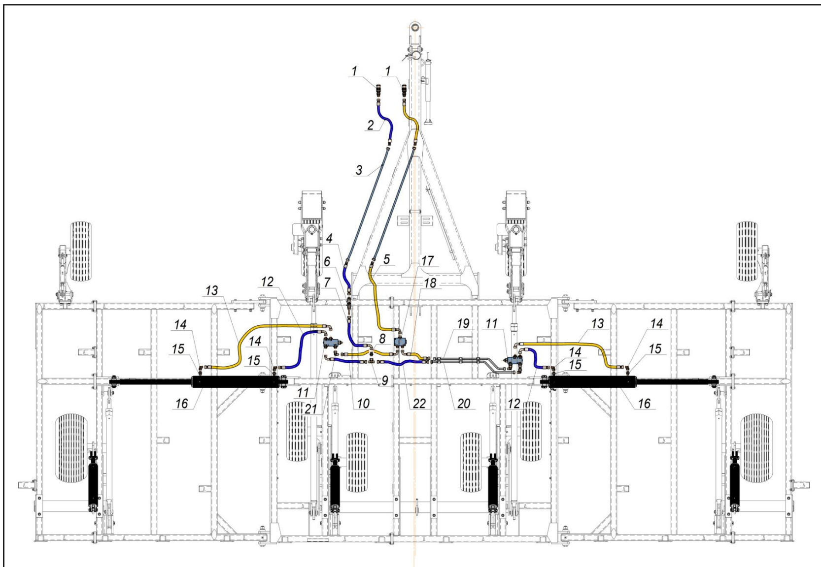
Рисунок Г.2 – Гидравлические соединения культиваторной части комплекса посевного SH-10200 (соединение гидроцилиндров подъёма крыльев)
