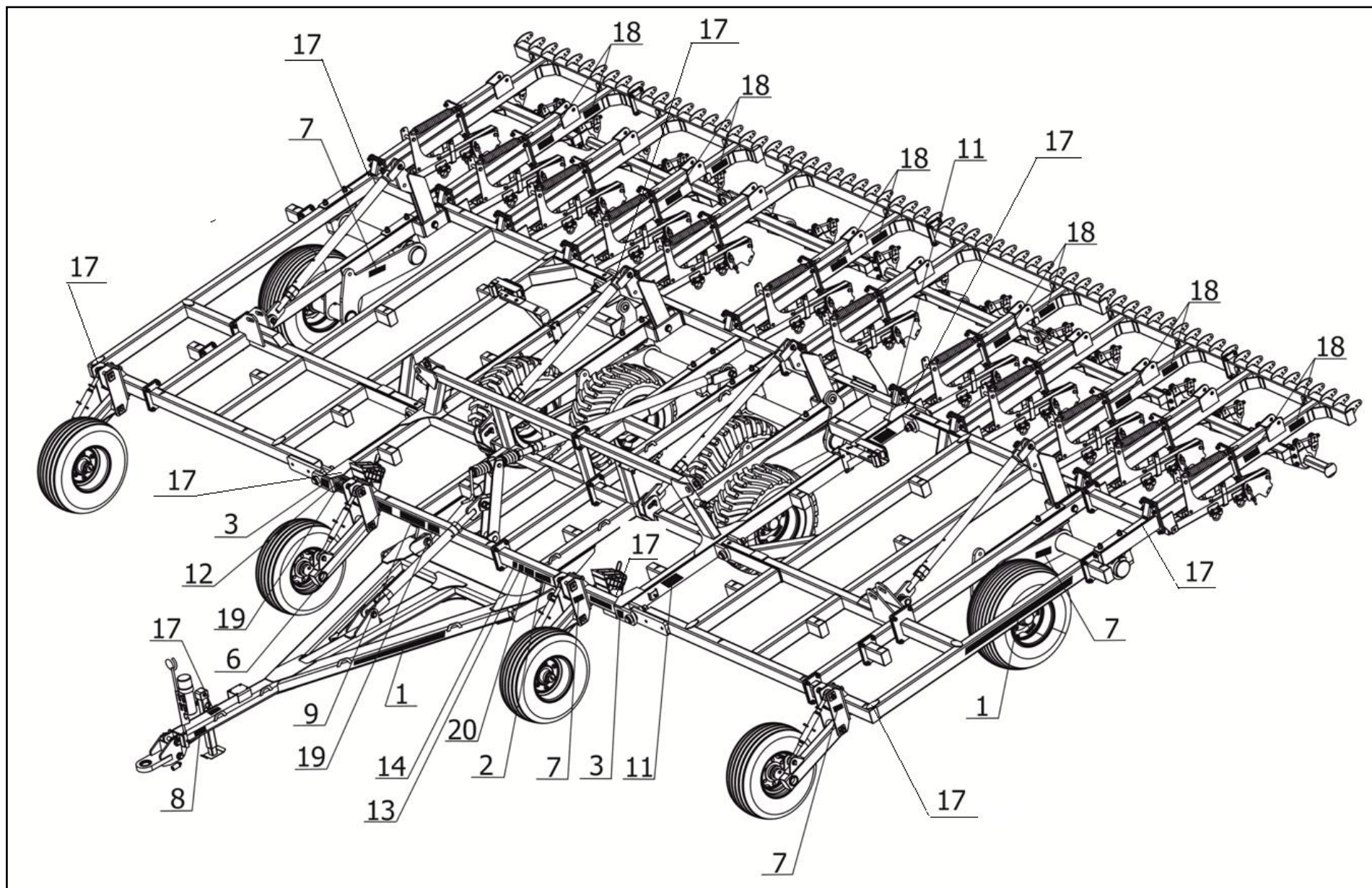
Рисунок 5.1 – Месторасположение табличек на культиваторной части (Лист 1 из 2)
