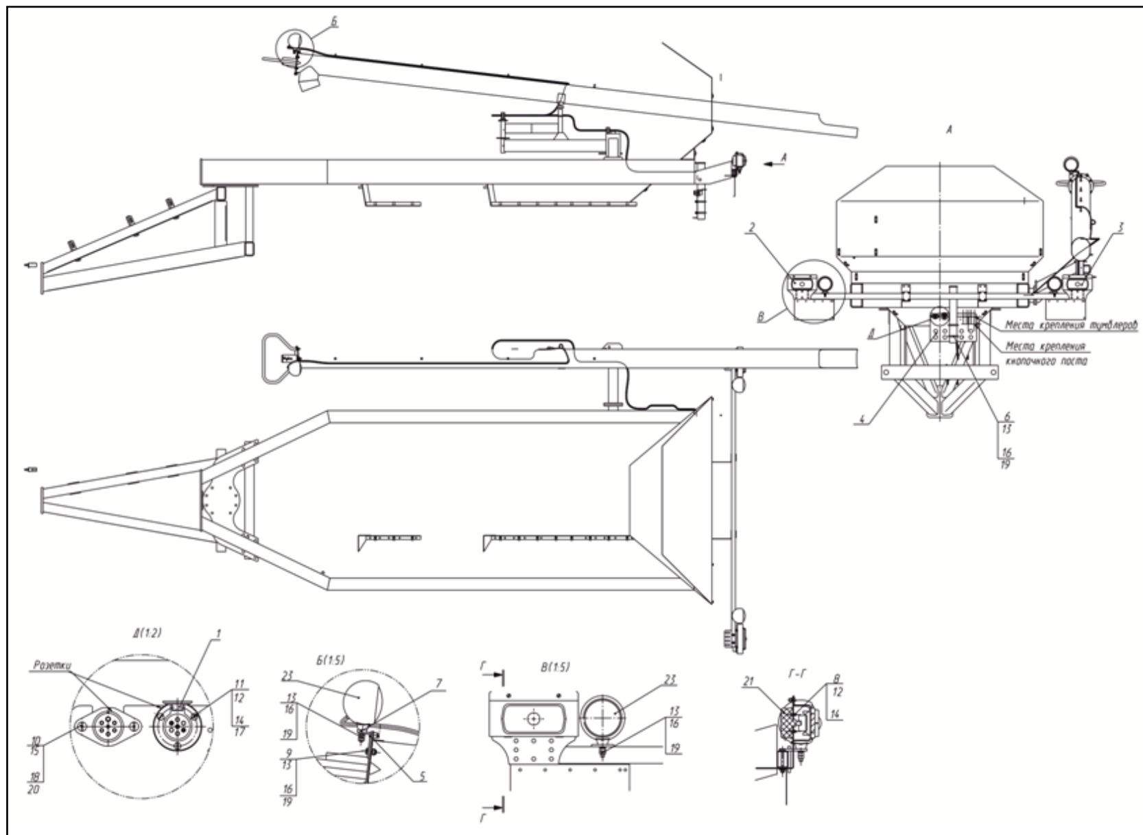
Рисунок В.1 – Схема коммуникаций электрических бункера АТ-11
