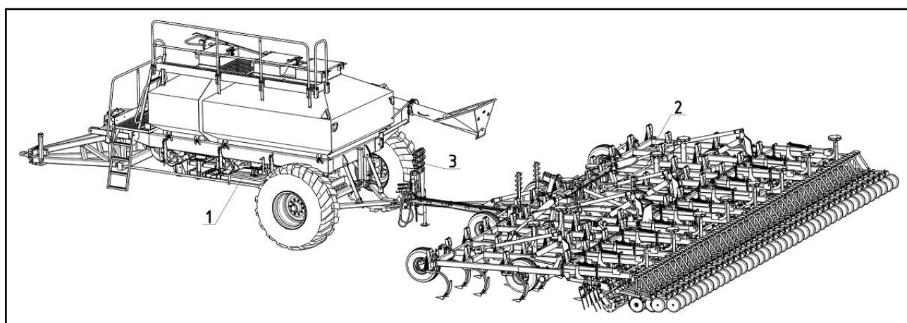
1 – Пневматический бункер; 2 – Культиваторная часть; 3 – Пневмораспределительная система Рисунок 3.1 Общий вид комплекса посевного гибридного типа SH-10200
