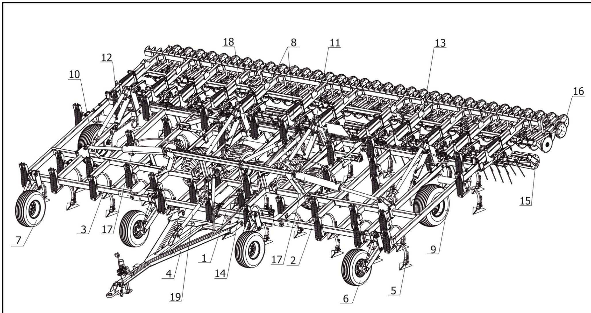
1 – Центральная рама; 2, 3 – Крылья; 4 – Сница; 5 – Рабочий орган; 6, 7 – Опорное колесо; 8 – Шасси; 9, 10 – Шасси крыла; 11 – Гидроцилиндр шасси; 12, 13 – Тяга регулировки глубины обработки; 14 – Регулятор горизонта; 15 – Шлейф; 16 – Посевной модуль; 17 – Гидроцилиндр; 18 – Кронштейн; 19 – Тяга Рисунок 3.5 – Общий вид культиваторной части комплекса
