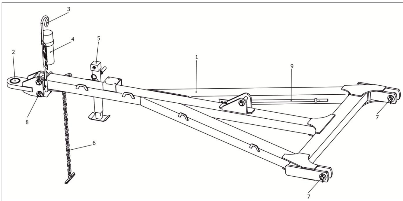
1 – Сница; 2 – Прицеп; 3 – Стойка-держатель; 4 – Тубус; 5 – Домкрат; 6 – Цепь; 7, 8 – Ось; 9 – Чистик
