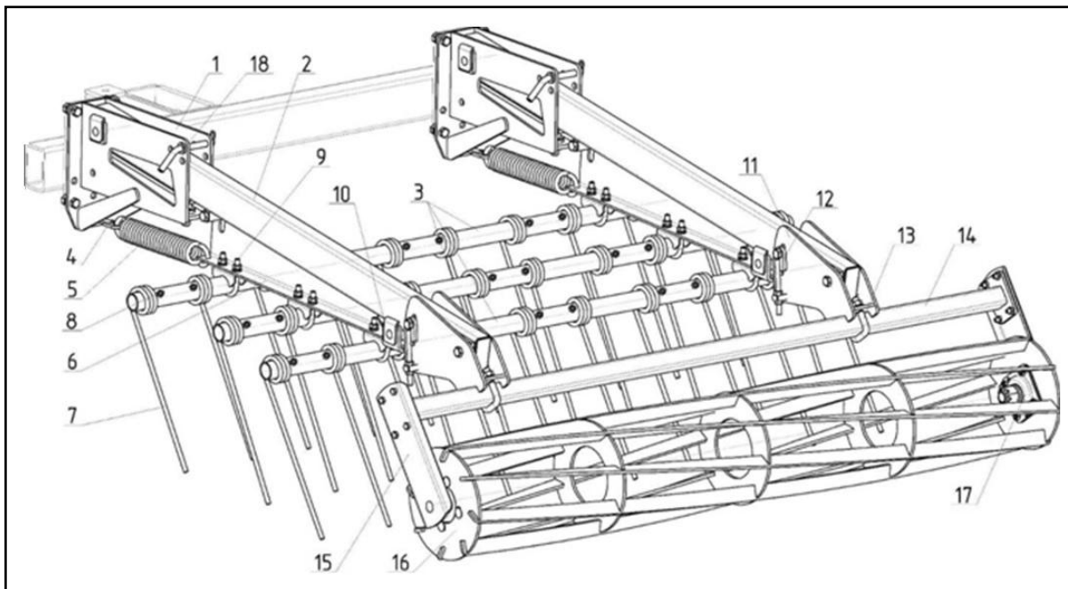
1 – Кронштейн; 2 – Поводок; 3 – Труба; 4 – Натяжитель; 5 – Пружина; 6 – Основание; 7 – Зуб пружинный; 8 – Болт; 9 – Хомут; 10 – Ось; 11 – Кронштейн; 12 – Натяжитель; 13 – Хомут; 14 – Перемычка; 15 – Боковина; 16 – Ротор; 17 – Подшипник; 18 – Штырь
