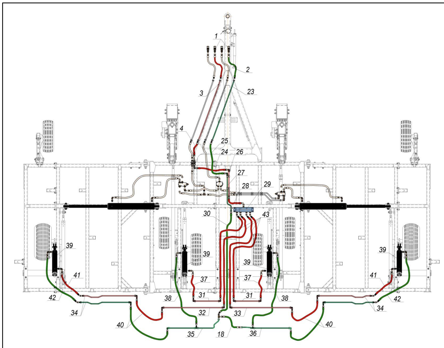
Рисунок Г.3 – Гидравлические соединения культиваторной части комплекса посевного SH-10200 (соединение гидроцилиндров шасси)
