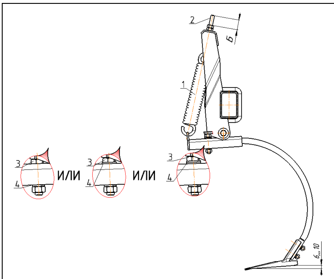
1 – Пружина; 2 – Натяжитель; 3 – Болт М16×70; 4 – Шайба 16 Рисунок 7.5.1 – Регулировка степени натяжения пружин
