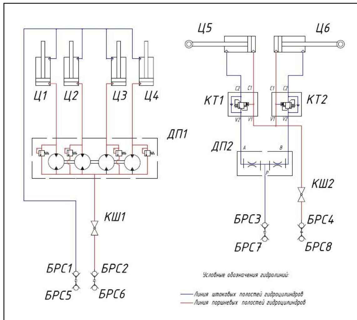
Рисунок Г.1 – Схема гидравлическая принципиальная культиваторной части комплекса посевного SH-10200
