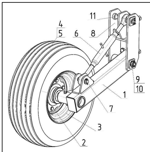
Рисунок 4.6 – Колесо опорное
