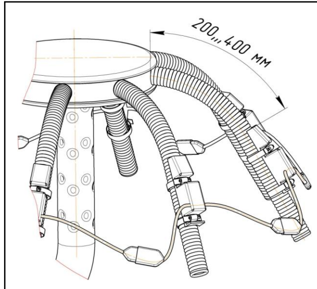
Рисунок 4.16 – Установка датчика контроля семян на семяпровод
