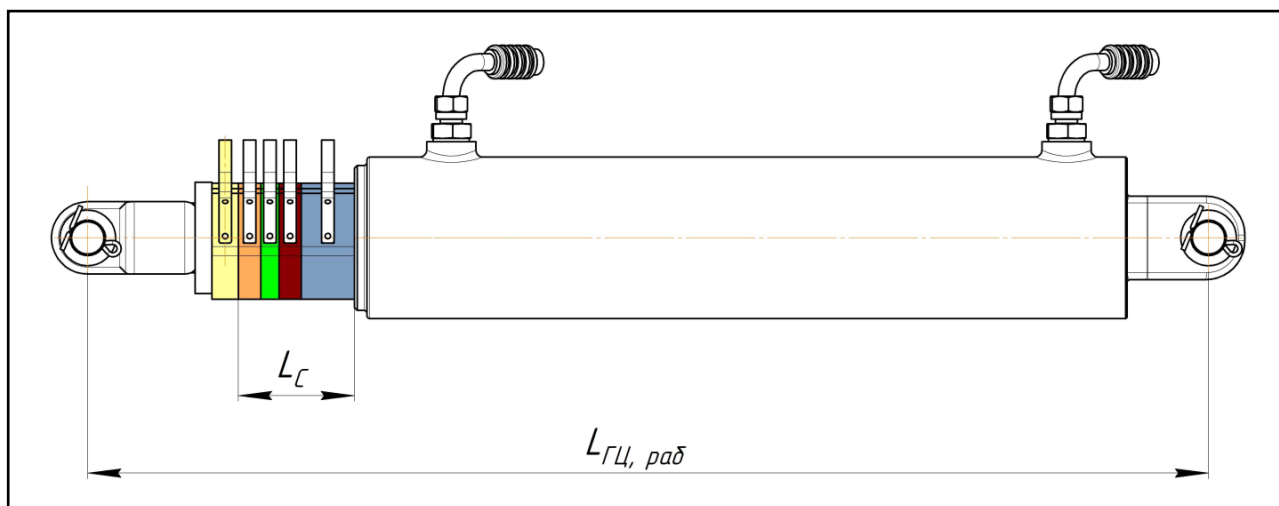
Рисунок 7.1.3 – Установка стоп-сегментов на шток гидроцилиндра шасси
