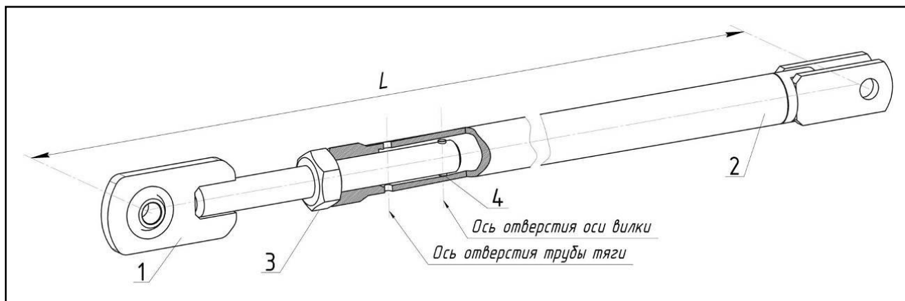
1 – Тяга; 2 – Вилка; 3 – Гайка; 4 – Штифт
