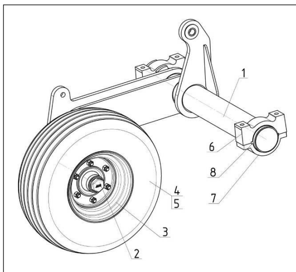
Рисунок 4.3 – Шасси
