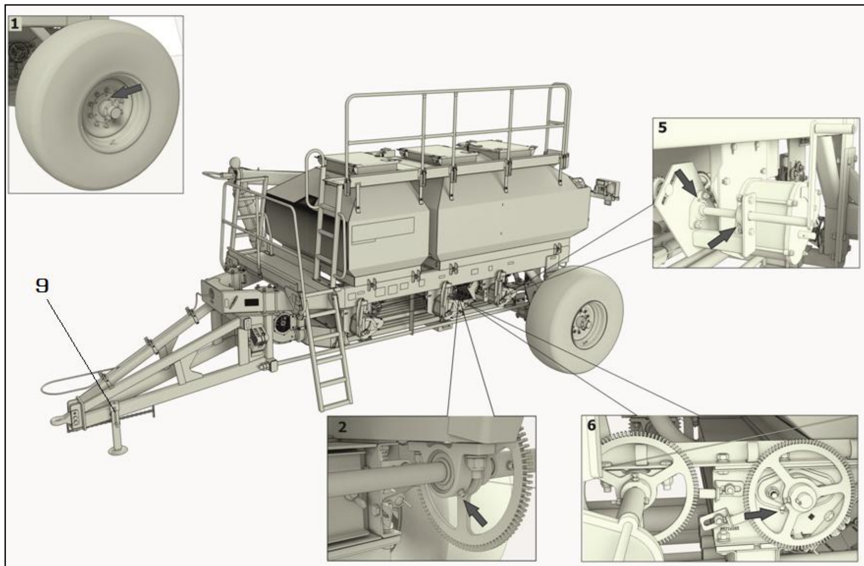
Рисунок 8.2 – Точки смазки бункера АТ-11
