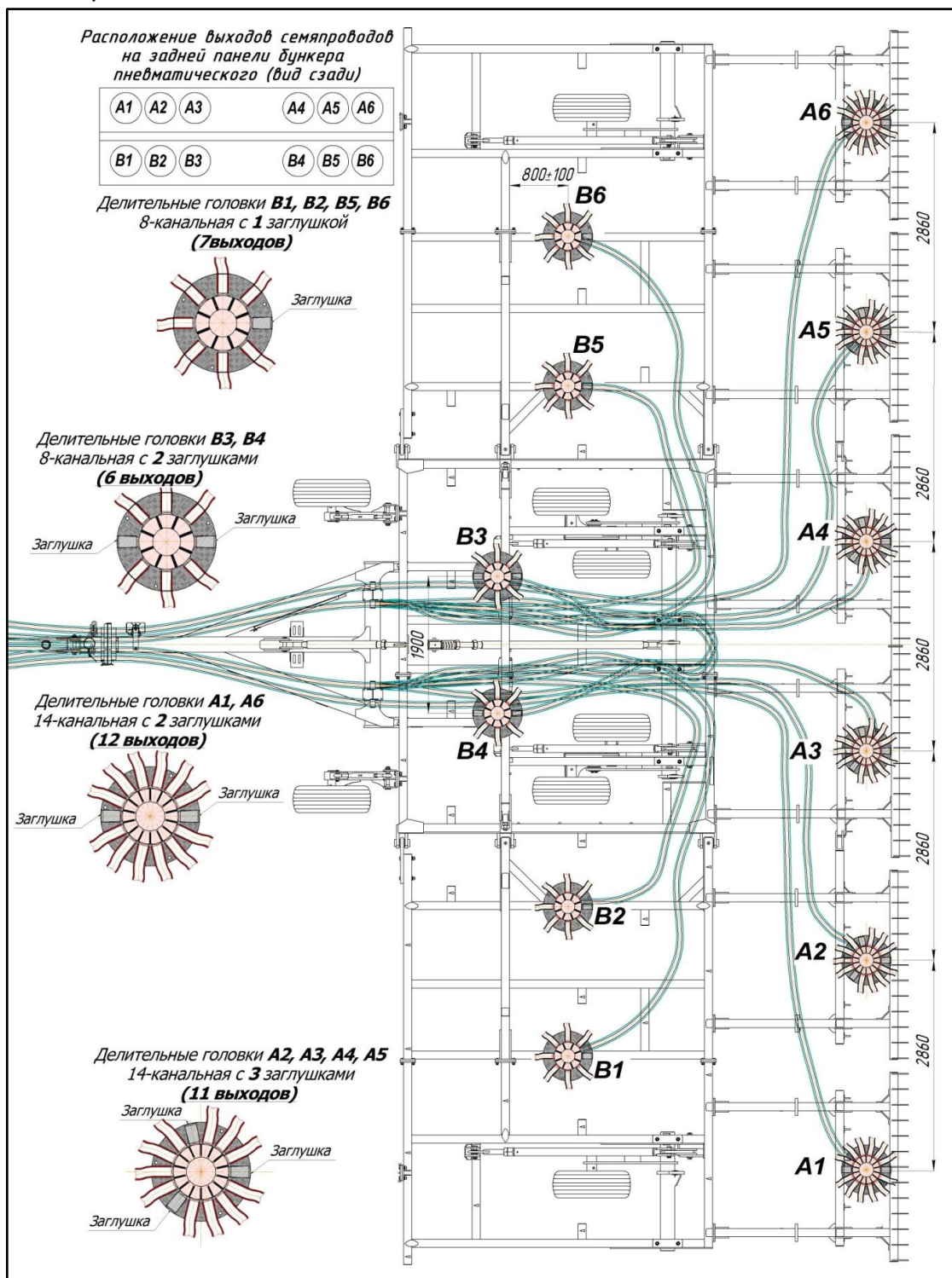
Рисунок 4.15 – Пневмораспределительная система комплекса посевного
