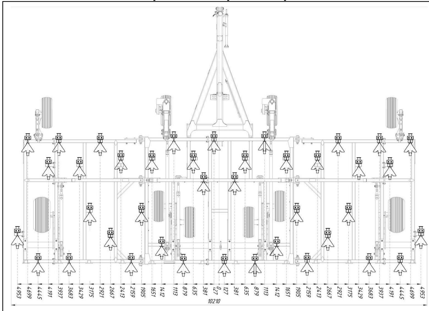
Рисунок Е.1 – Схема расстановки рабочих органов
