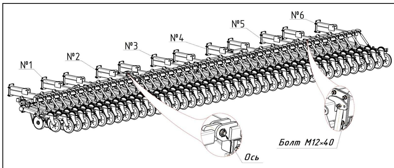
Рисунок 4.12 – Установка посевных модулей
