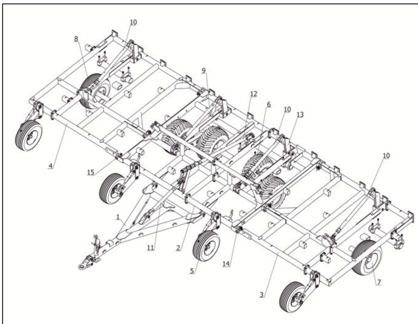
1 – Сница; 2 – Рама в сборе; 3 – Крыло левое; 4 – Крыло правое; 5 – Колесо опорное; 6 – Шасси; 7, 8 – Шасси крыла; 9, 10, 11 – Тяга; 12 – Регулятор горизонта; 13 – Кронштейн; 14, 15 – Пальцы Рисунок 4.1 – Рамная конструкция культиваторной части комплекса
