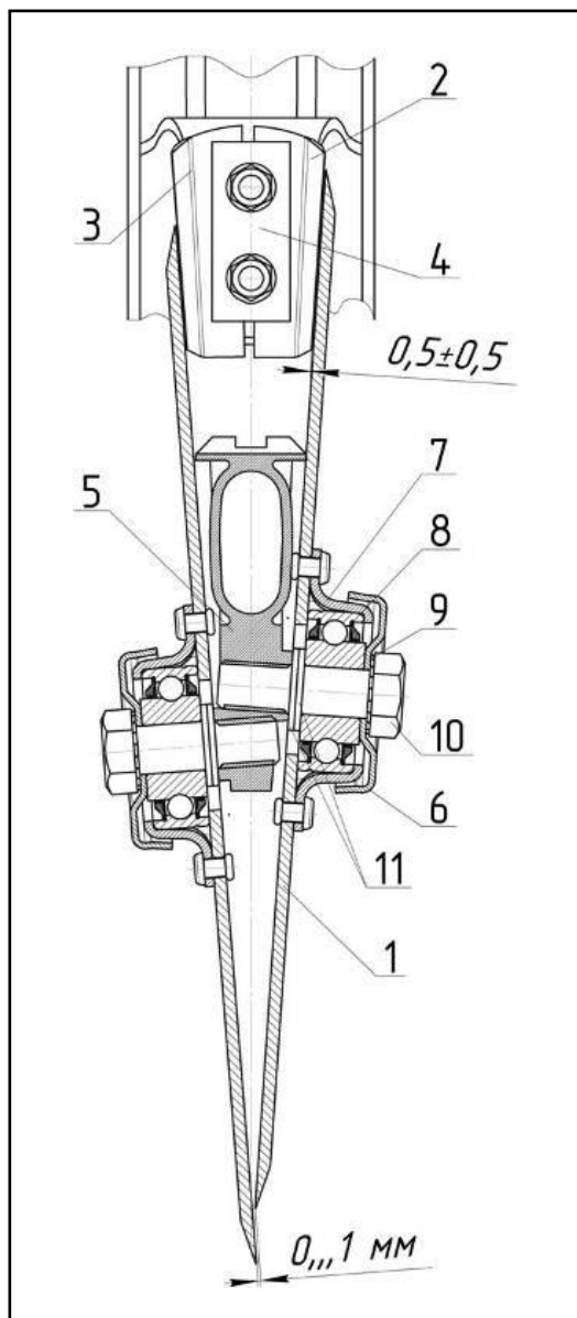
Рисунок 7.6 – Параметры дискового сошника
