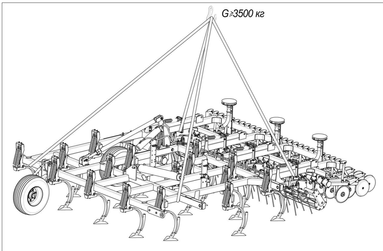
Рисунок 11.3 – Вид крыла правого культиватора при подготовке к транспортированию
