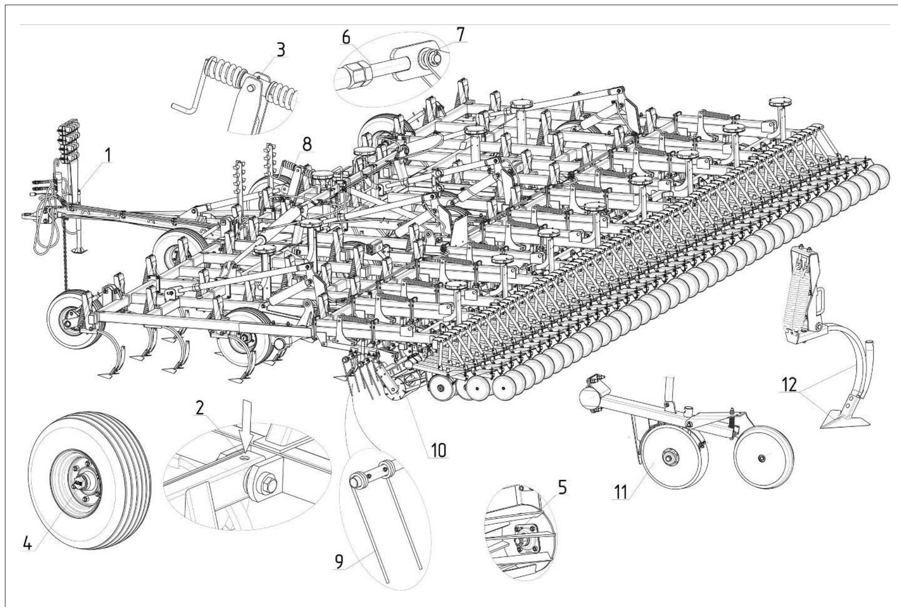
Рисунок 8.1 – Места смазки культиваторной части
