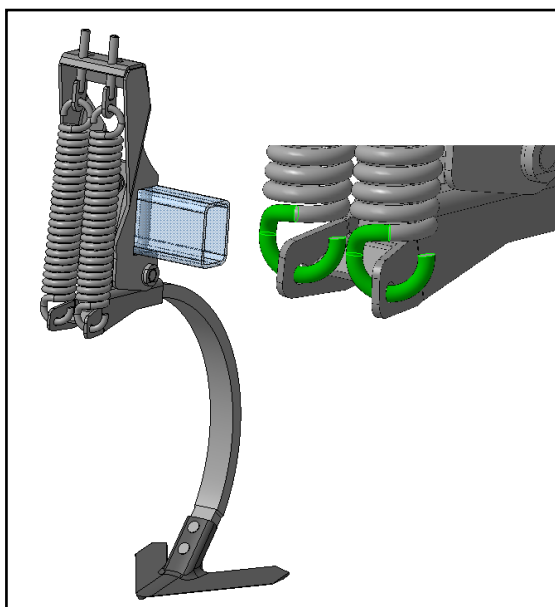
Рисунок 7.5.2 – Установка пружин и натяжителей подвески рабочего органа
