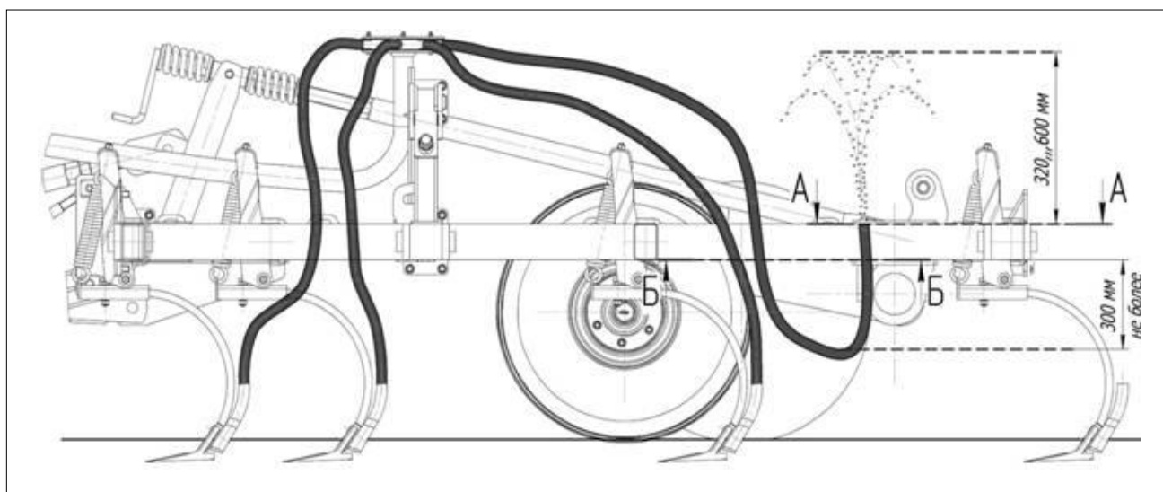
Рисунок 7.7 – Регулировка воздушного потока
