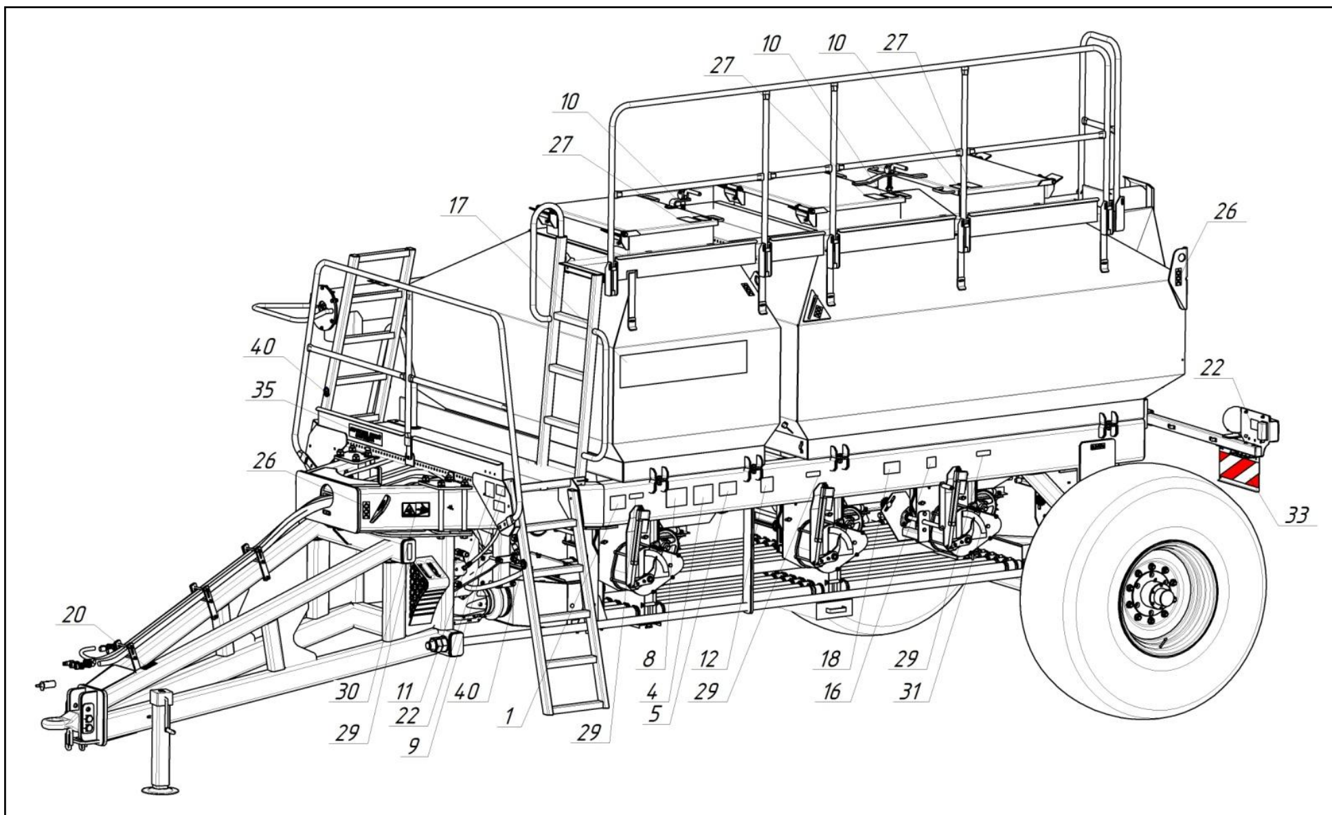
Рисунок 5.2 – Месторасположение табличек на бункере АТ-11 (Лист 1 из 4)
