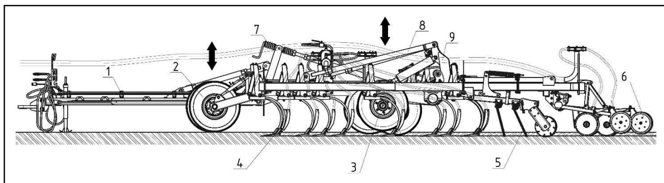
1 – Сница; 2 – Колесо опорное; 3 – Колесо шасси; 4 – Рабочий оран; 5 – Бороновальный модуль; 6 – Посевная секция; 7 – Регулятор горизонта; 8 – Тяга регулировки глубины обработки; 9 – Кронштейн
