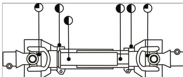
Рисунок 7.2 - Места смазки карданного вала
