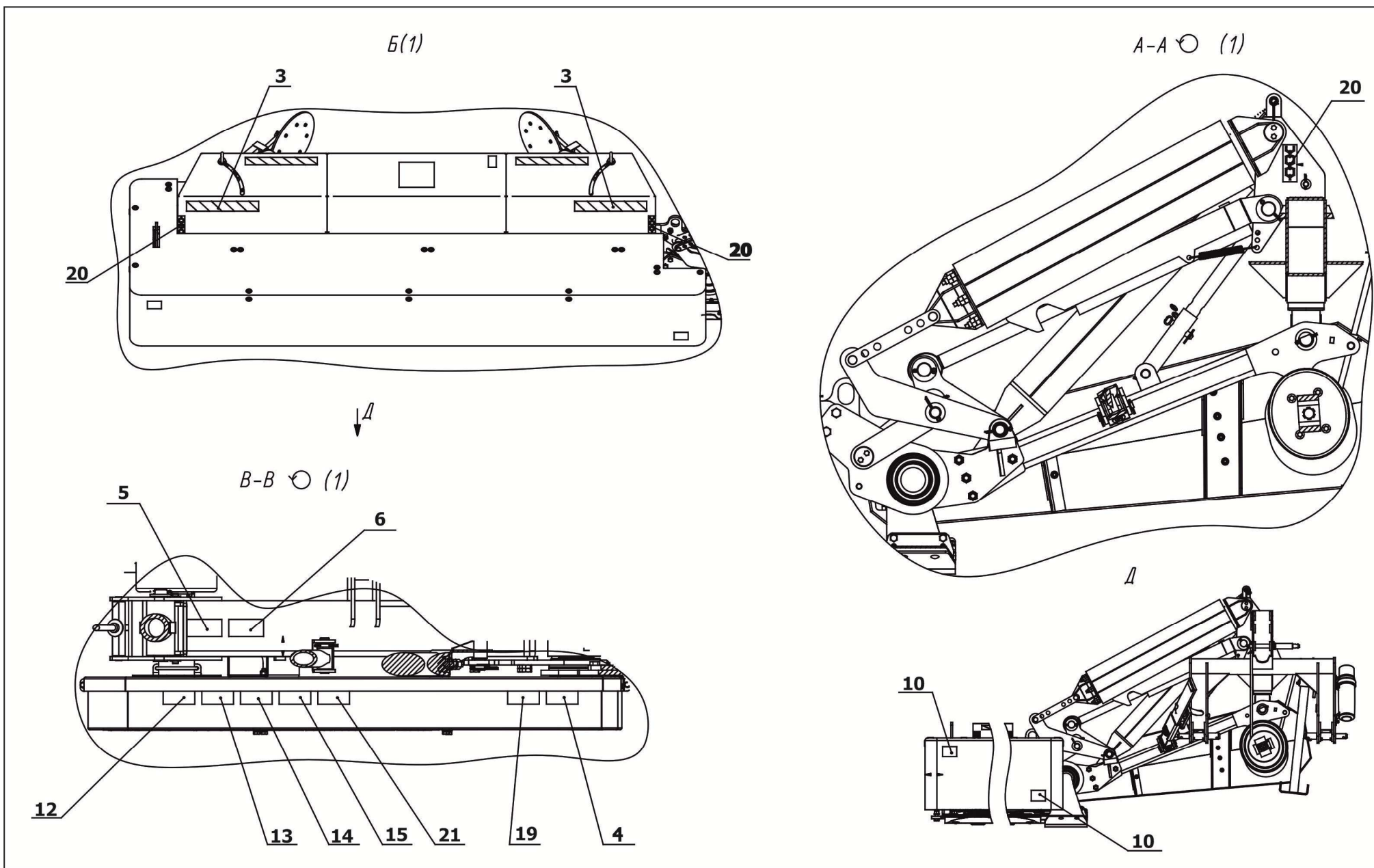
Рисунок 4.2 - Места расположения аппликаций и табличек на косилке
