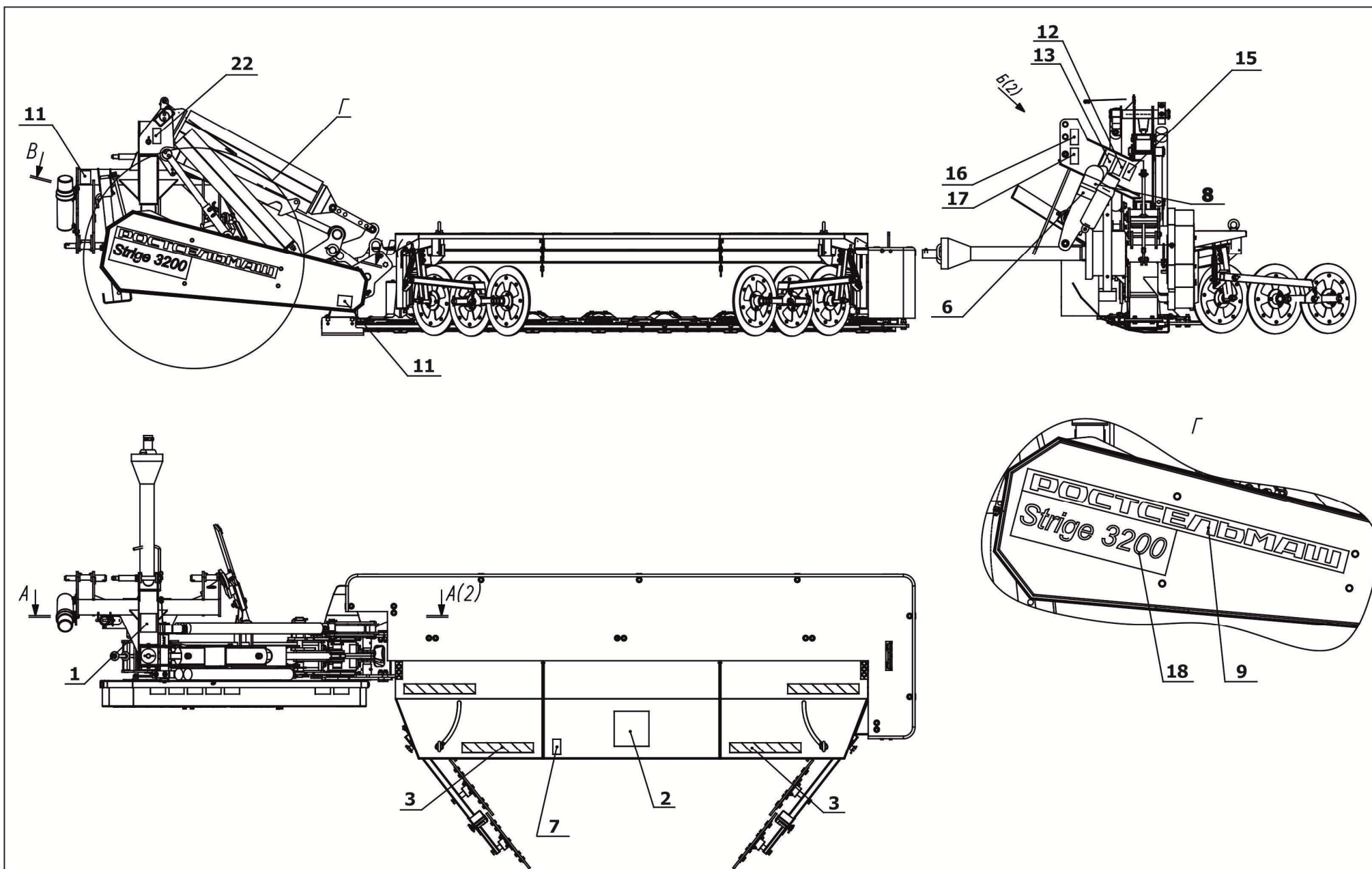
Рисунок 4.1 - Места расположения аппликаций и табличек на косилке
