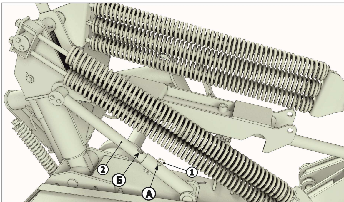
А – рабочее положение косилки; Б – транспортное положение косилки 1 – Фиксатор; 2 - Устройство телескопическое стопорное
