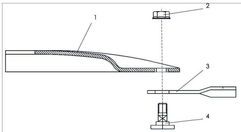
1 - Ротор; 2 - Гайка; 3 - Нож; 4 - Болт Рисунок 6.6 - Крепление скашивающего ножа к ротору
