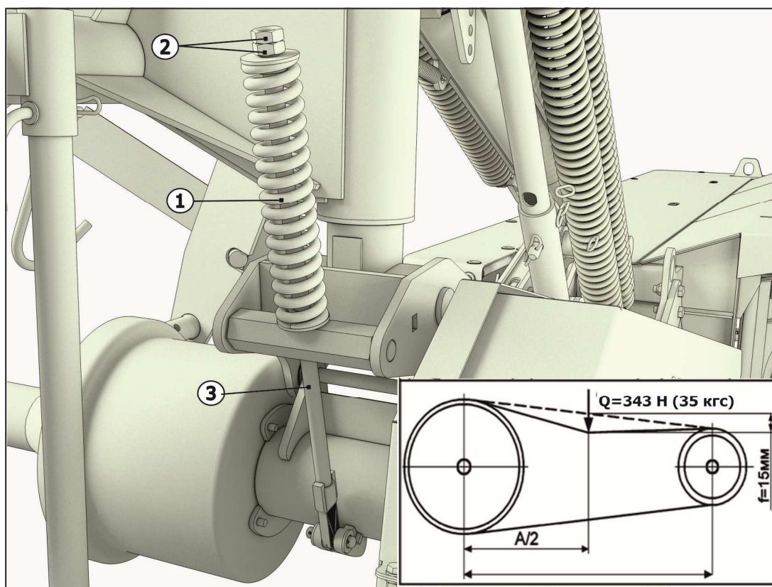
Рисунок 6.10 - Регулировка натяжения ременной передачи
