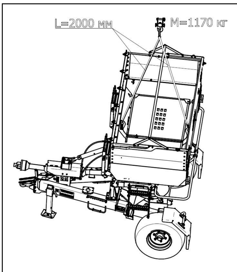
Рисунок 8.1 – Схема строповки
