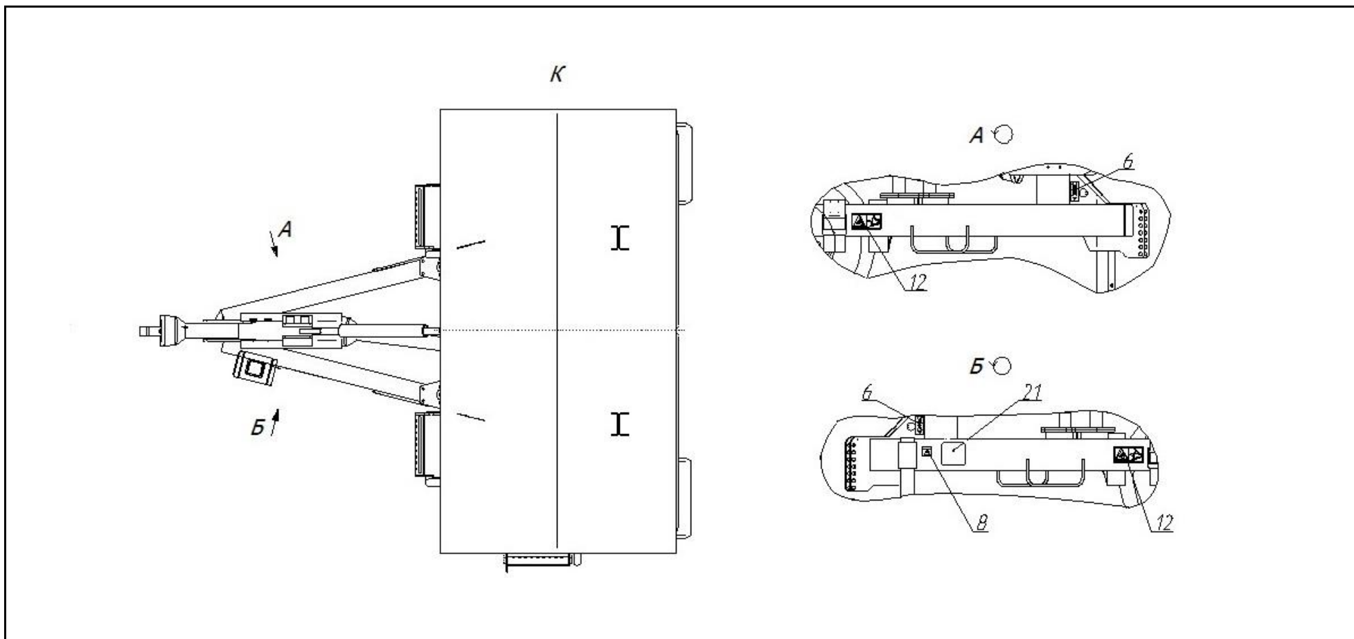
Рисунок 4.1 – (Лист 2 из 3)
