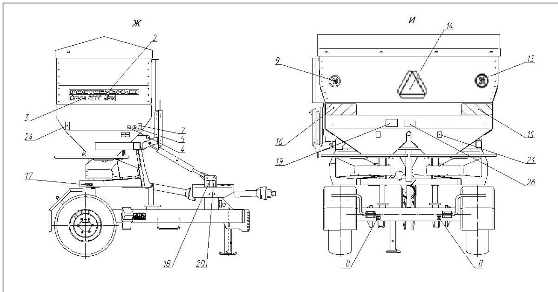
Рисунок 4.1 – (Лист 3 из 3)
