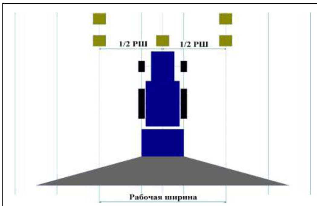
Рисунок 6.6 – Установка поддонов
