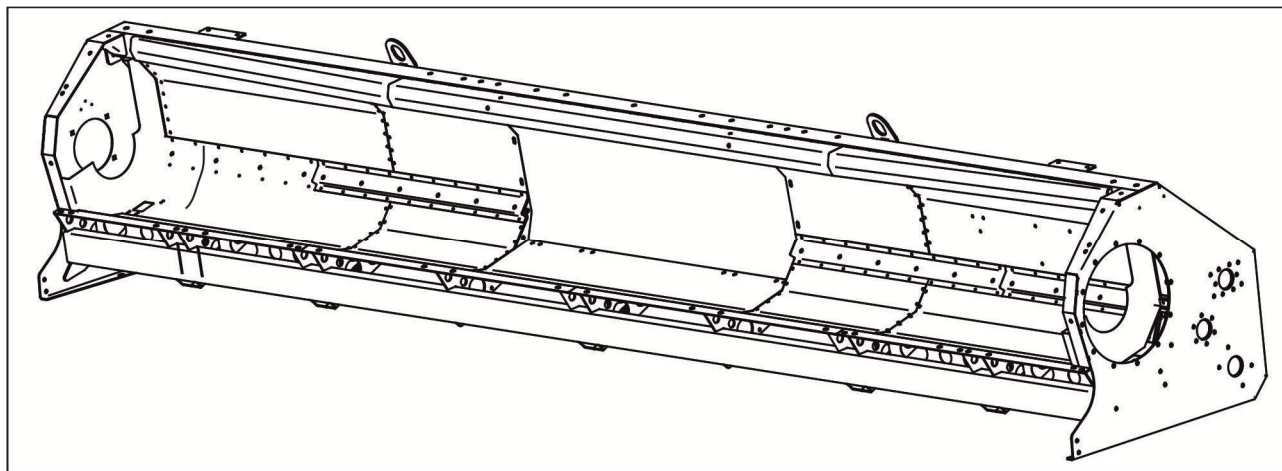
Рисунок 2.2 - Каркас
