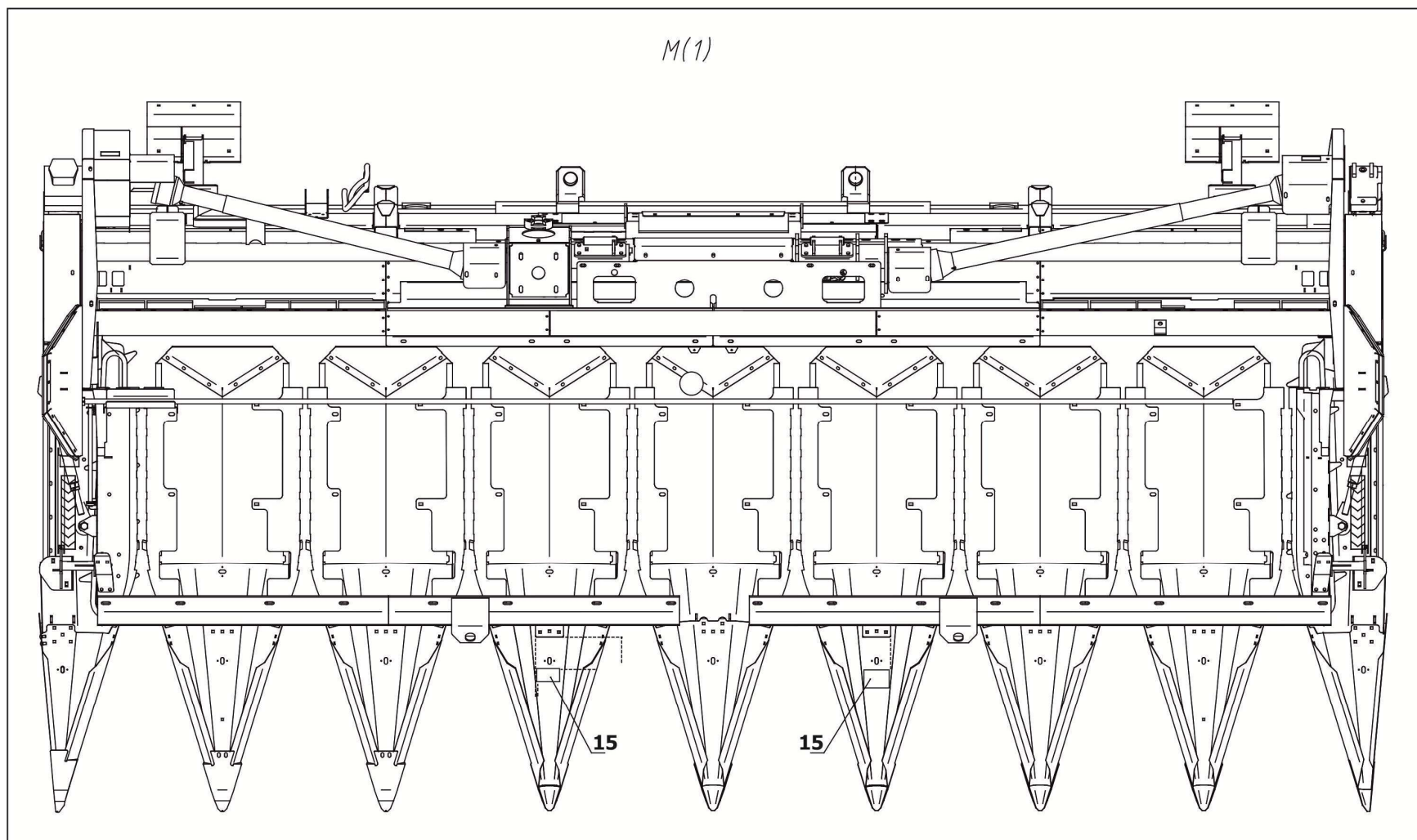
Рисунок 4.1 – Месторасположение табличек и аппликаций
