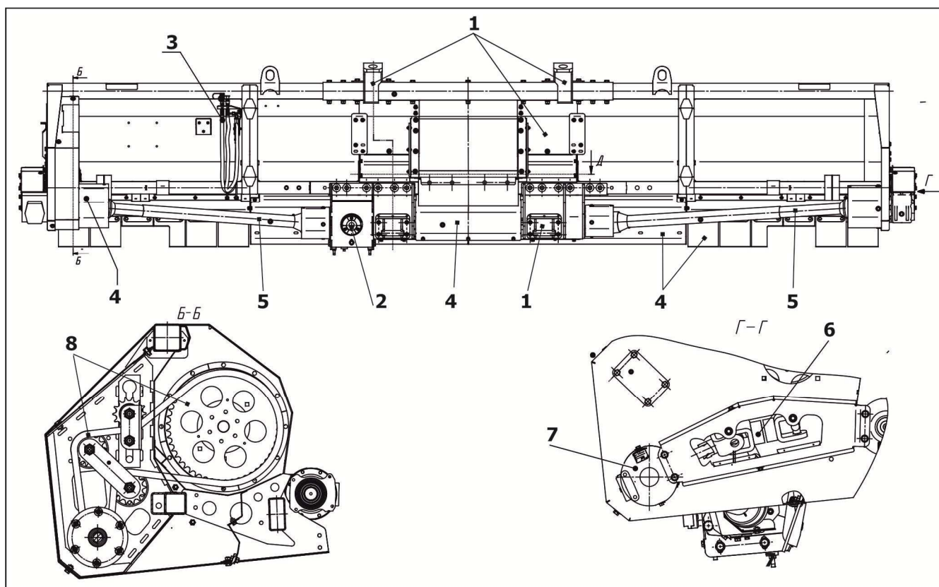
1 – Рамка; 2 – Редуктор; 3 – Гидрооборудование; 4 – Установка щитков; 5, 6 – Карданный вал; 7 – Редуктор правый; 8 – Привод шнека
