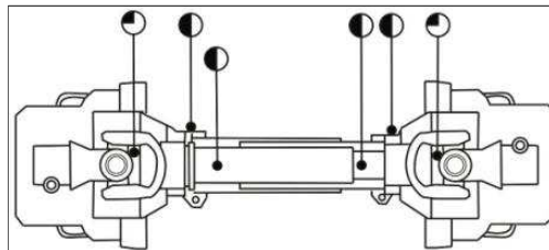
Рисунок 8.2 - Места смазки карданного вала
