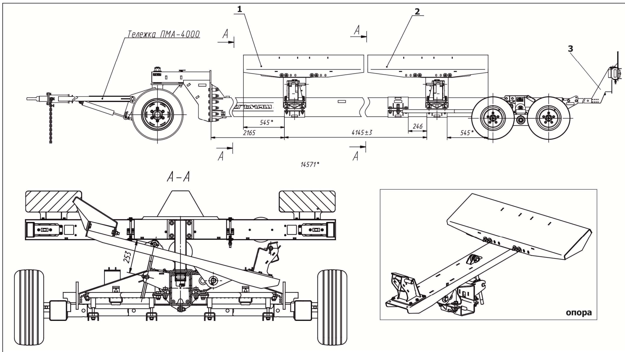
Рисунок 9.2 – Схема установки комплекта опор на тележку
