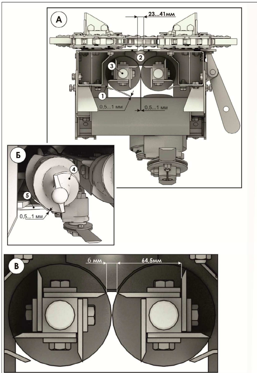
1 – Чистик; 2 – Отрывочная пластина; 3 – Протягивающий валец; 4 – Конусный шнек вальца; 5 – Чистик Рисунок 7.4 - Регулировки русла
