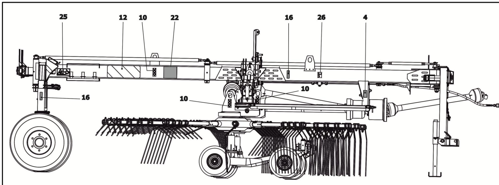
Рисунок 4.1 – Месторасположение табличек и аппликаций на граблях (Лист 1 из 4)
