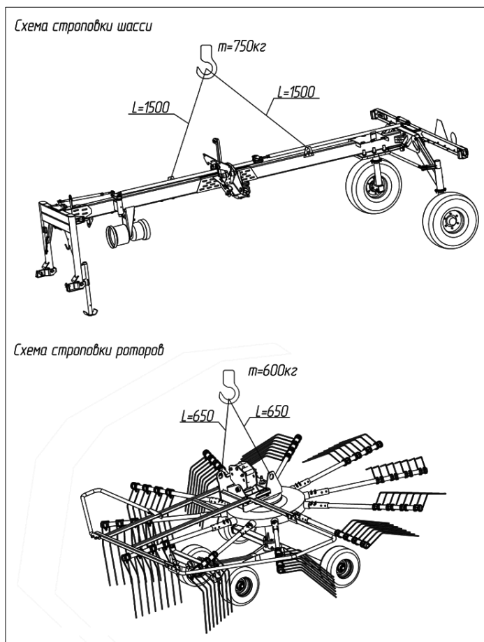
Рисунок 9.1 – Схема строповки
