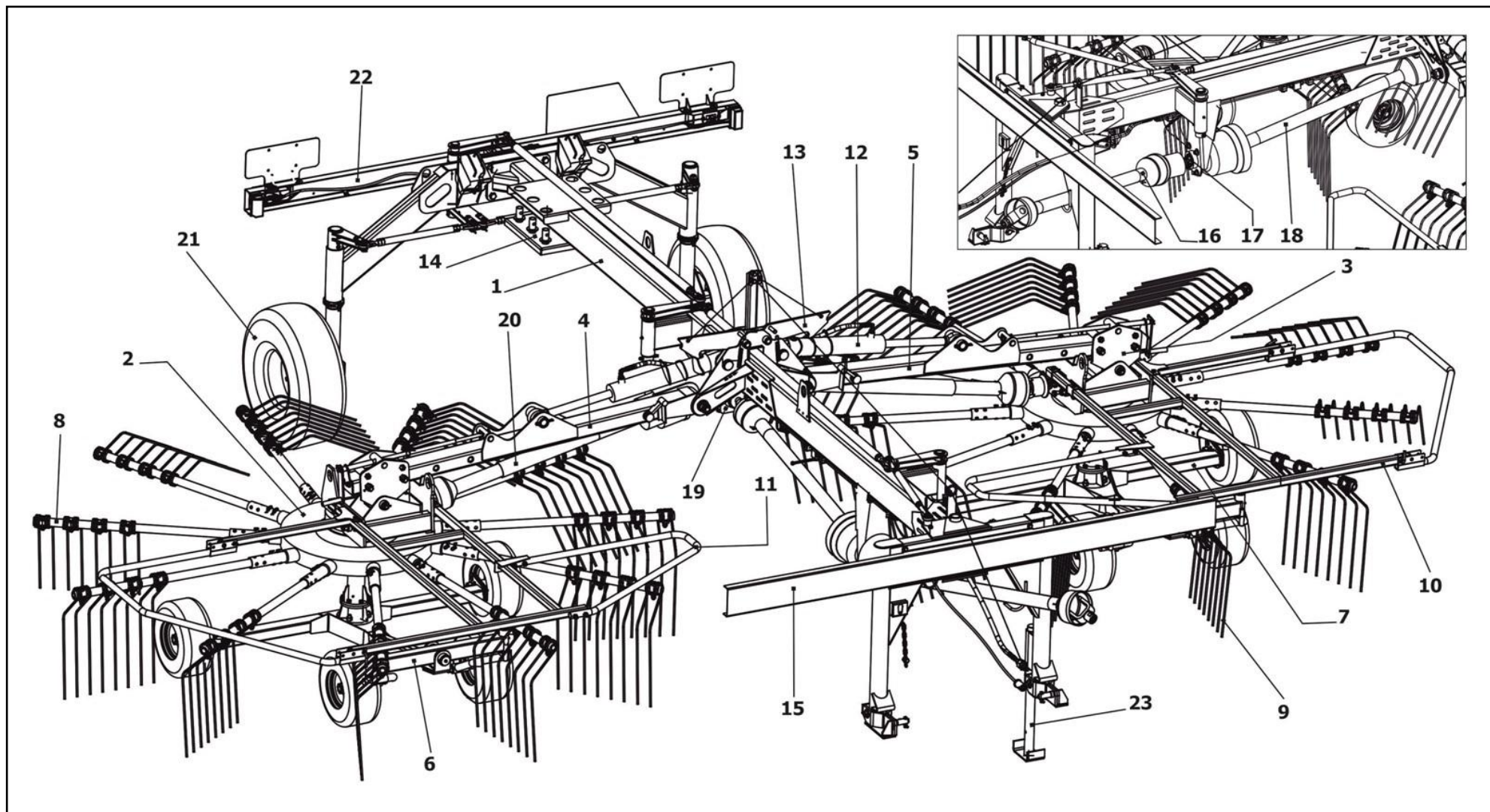
1 – Балка средняя; 2, 3 – Ротор; 4, 5 – Балка ротора; 6, 7 – Шасси тележки; 8, 9 – Граблина; 10, 11 – Ограждение; 12 – Гидроцилиндр; 13 – Зацеп; 14 – Кронштейн; 15 – Навеска; 16, 18, 20 – Вал карданный; 17 – Привод; 19 – Редуктор конический; 21 – Колесо; 22 – Балка задняя; 23 – Опора
