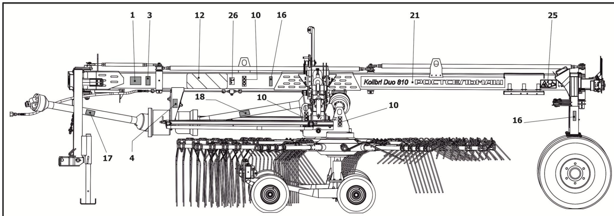
Рисунок 4.1 – (Лист 2 из 4)
