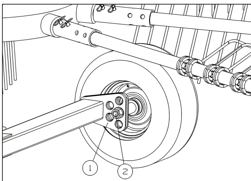
1 – Кронштейн; 2 – Колесо
