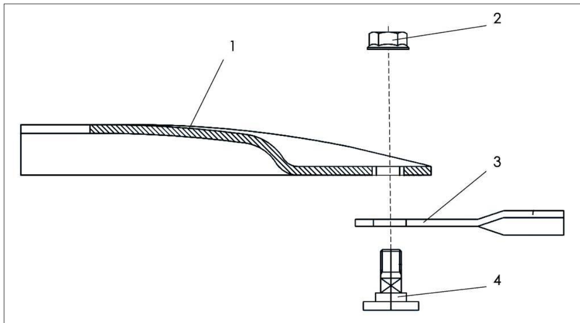
Рисунок 3.7 – Крепление скашивающего ножа к ротору
