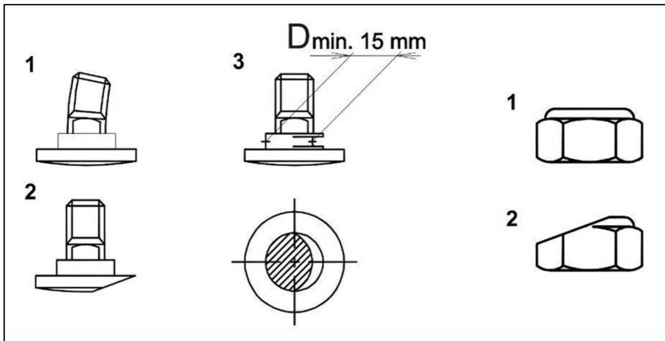
Рисунок 3.9 – Замена болтов и гаек крепления ножей
