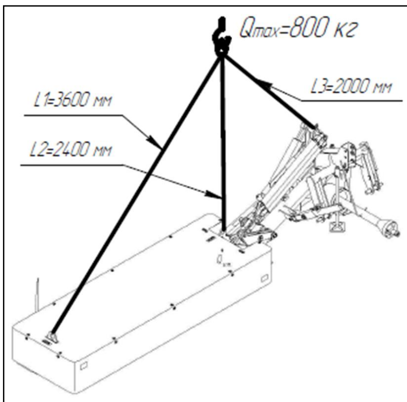
Рисунок 9.1 – Схема строповки
