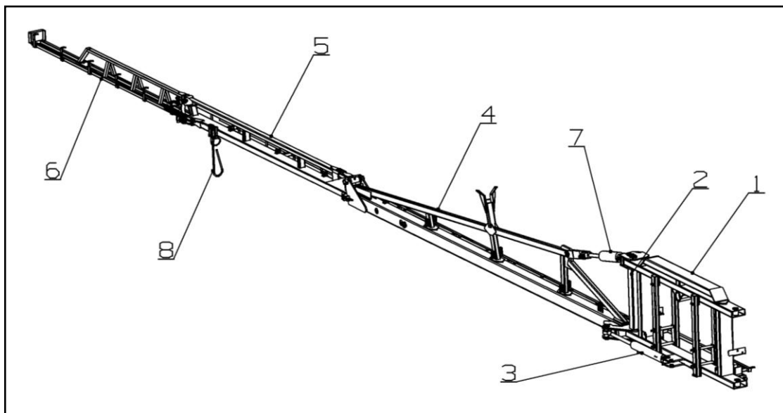
1 – Центральное звено; 2 – Шарнир 1-го звена; 3 – Гидроцилиндр раскладывания первого звена; 4 – 1-е звено; 5- 2-е звено; 6 – Противоударное звено; 7 – Гидроцилиндр вертикального положения крыла; 8 – Отбойник
