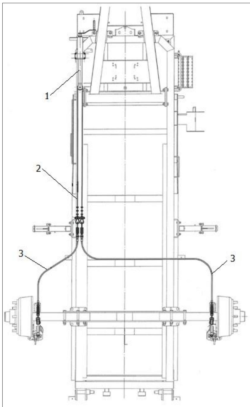
1 – Привод стояночного тормоза; 2 – Трос; 3 – Трос управления
