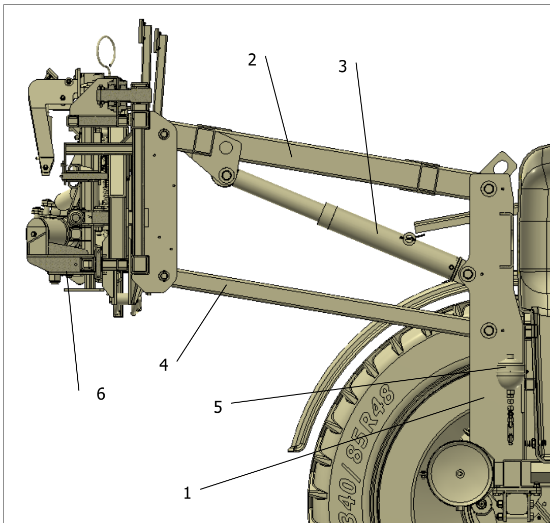
1 – Рама; 2 – Верхний рычаг; 3 – Гидроцилиндры подъема; 4 – Нижний рычаг; 5 – Пневмогидроаккумулятор; 6 – Штанга
