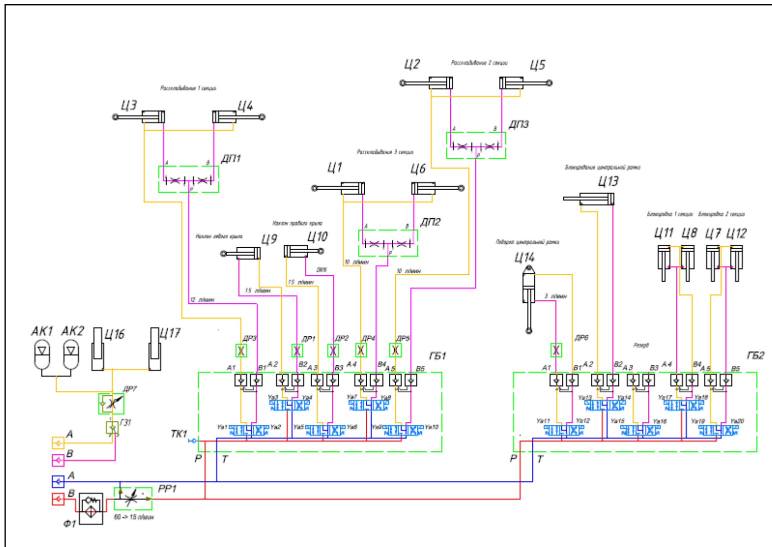
Рисунок Б.1 – Схема гидравлическая управления штангой семизвеной
