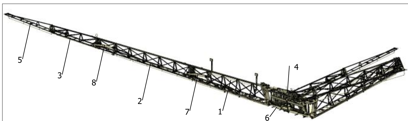
1 – Первое звено; 2 – Второе звено; 3 – Третье звено; 4 – Центральное звено; 5 – Противоударное звено; 6 – Гидроцилиндр раскладывания 1-го звена; 7 – Гидроцилиндр раскладывания 2-го звена; 8 – Гидроцилиндр раскладывания 3-го звена.
