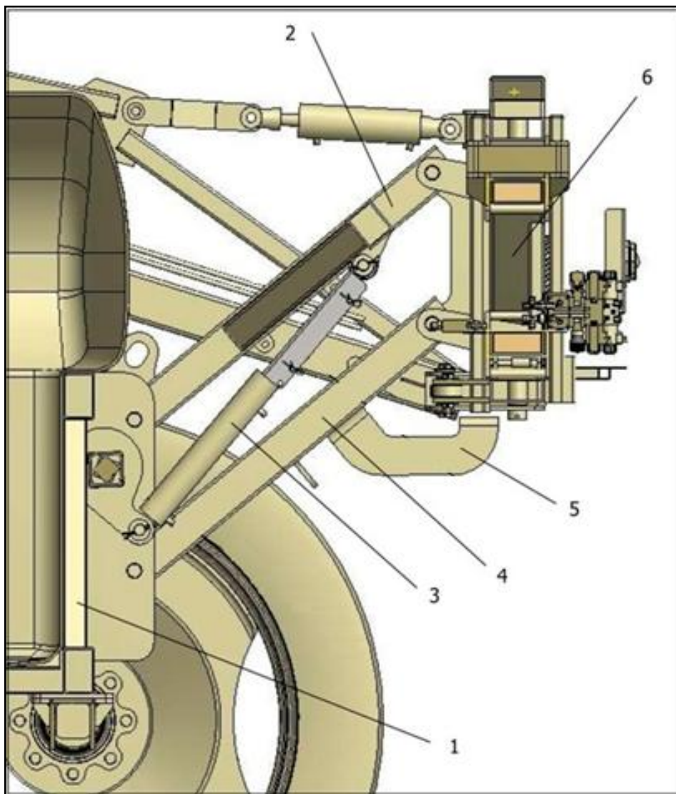
1 – Рама; 2 – Верхний рычаг; 3 – Гидроцилиндры подъема; 4 – Нижний рычаг; 5 – Фиксатор штанги в верхнем положении от раскочки; 6 – Штанга Рисунок 3.3.1 – Механизм подъема штанги (пятизвенной)
