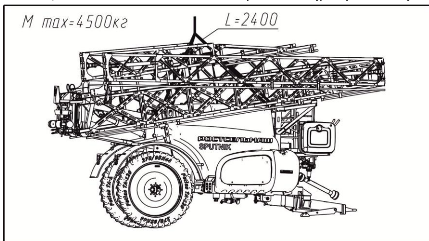
Рисунок 8.1 – Схема строповки
