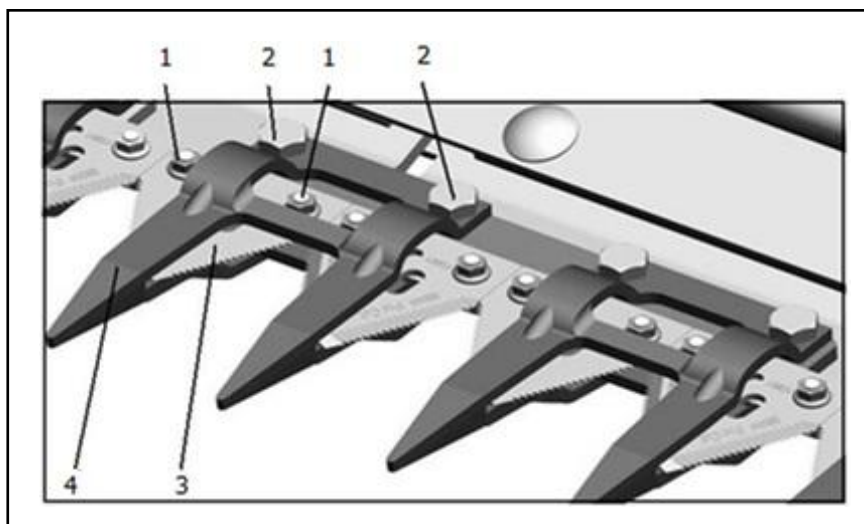
1, 2 – Болтокрепеж; 3 – Сегмент ножа; 4 – Палец
