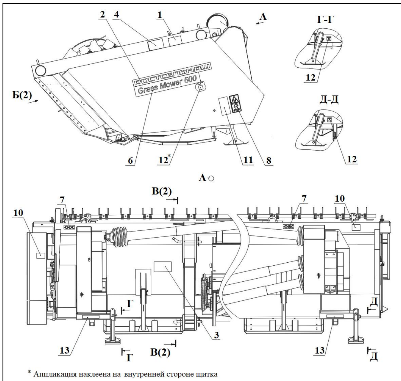
Рисунок 4.1 – Месторасположение табличек (Лист 1 из 2)
