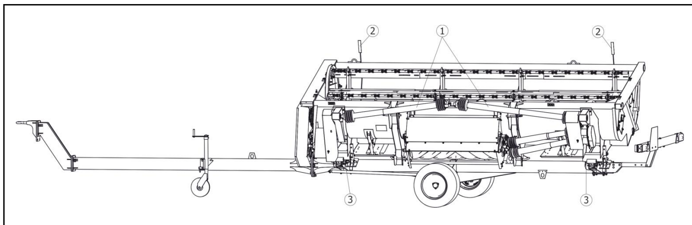
1 – Карданный вал; 2 – Маркер; 3 – Шплинт
