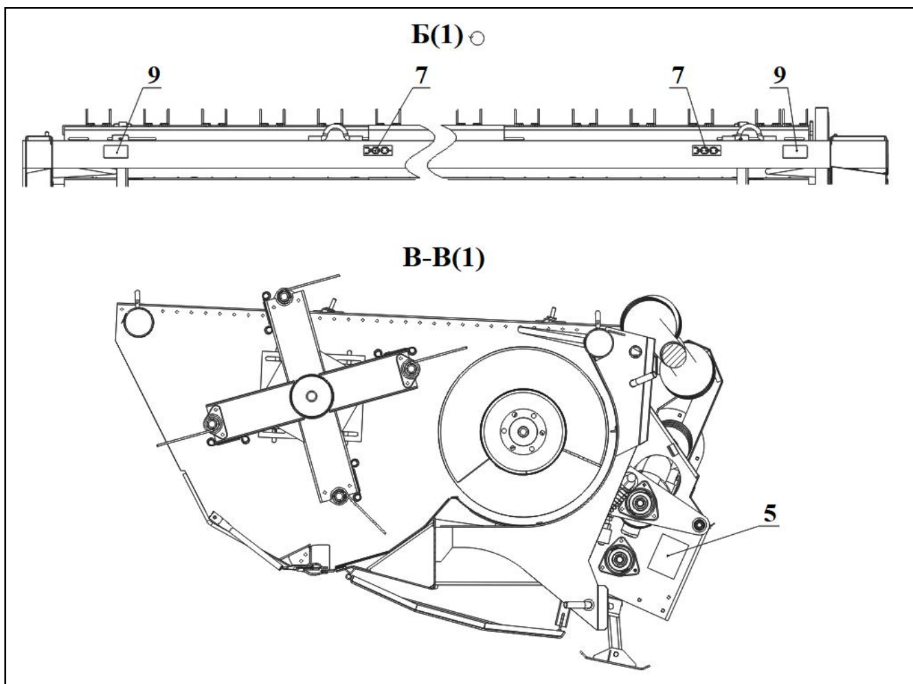
Рисунок 4.1 – Месторасположение табличек (Лист 2 из 2)
