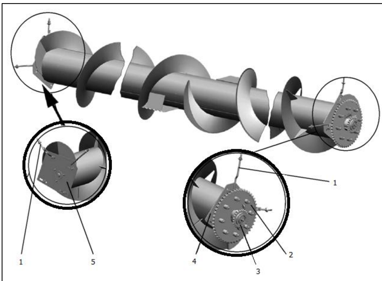
1 – Тяга; 2 – Звездочка с предохранительной фрикционной муфтой; 3 – Звездочка с обгонной муфтой; 4, 5 – Плита шнека
