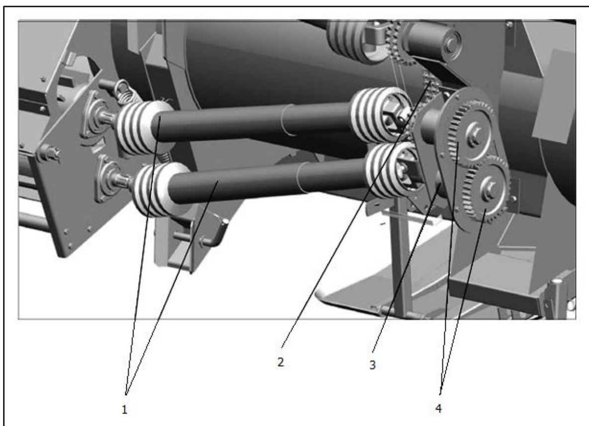
1 – Карданный вал; 2 – Цепь; 3 – Раздаточная гитара; 4 – Шестерня
