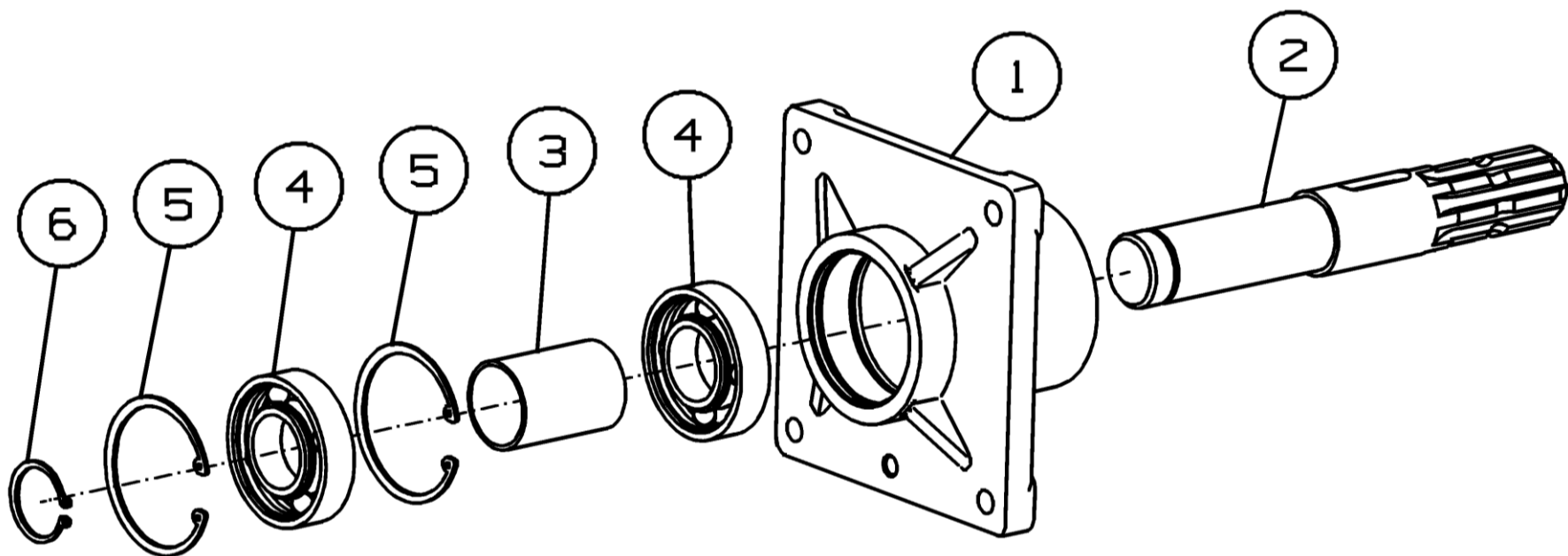
Рисунок 14 - Вал РСМ - 100.72.01.710
