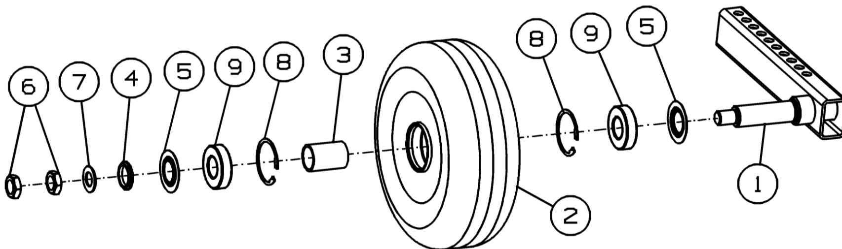
Рисунок 22 - Колесо PCM - 100.72.02.430M
