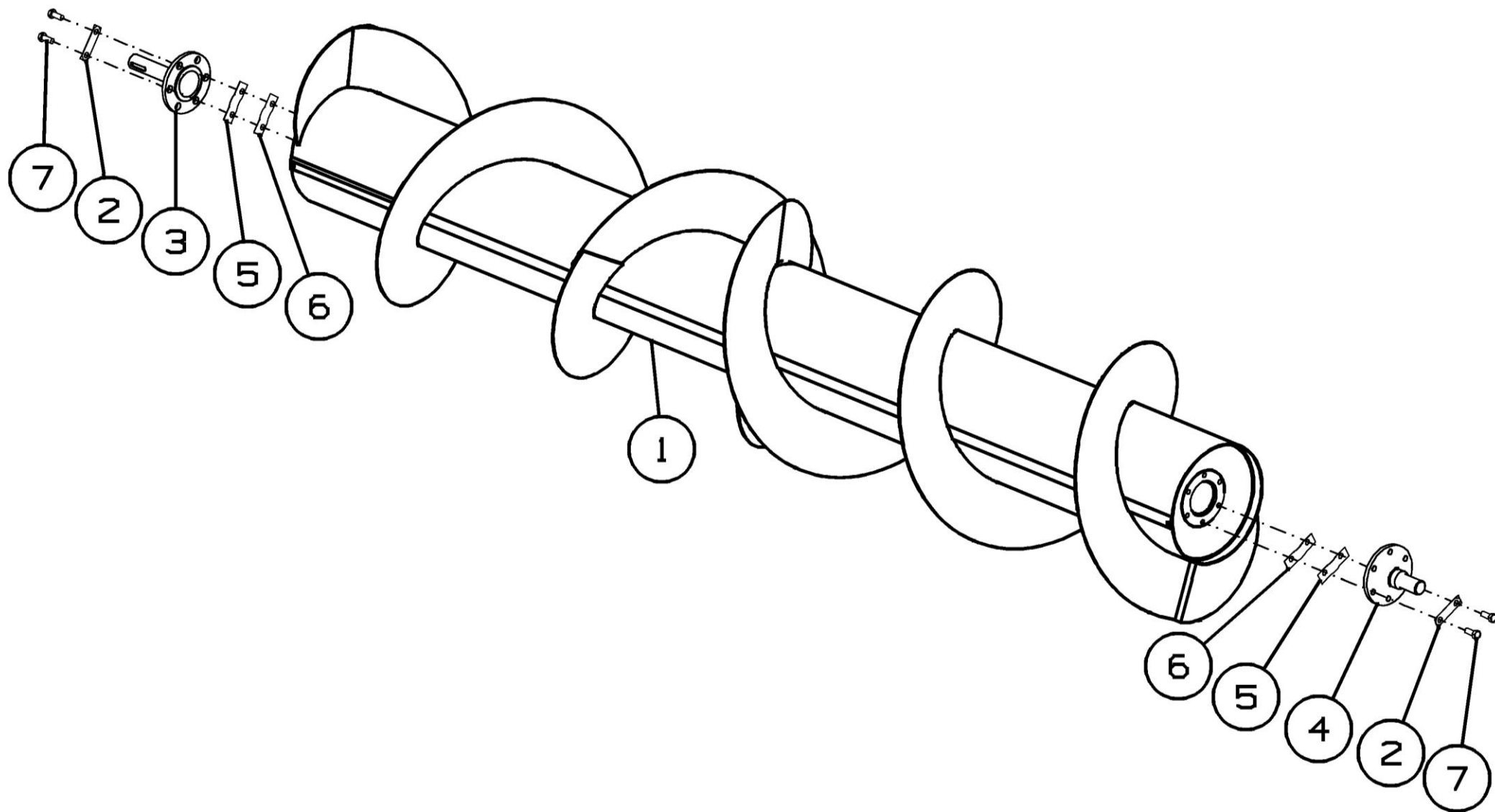
Рисунок 6 - Шнек МСМ - 100.72.01.020А
