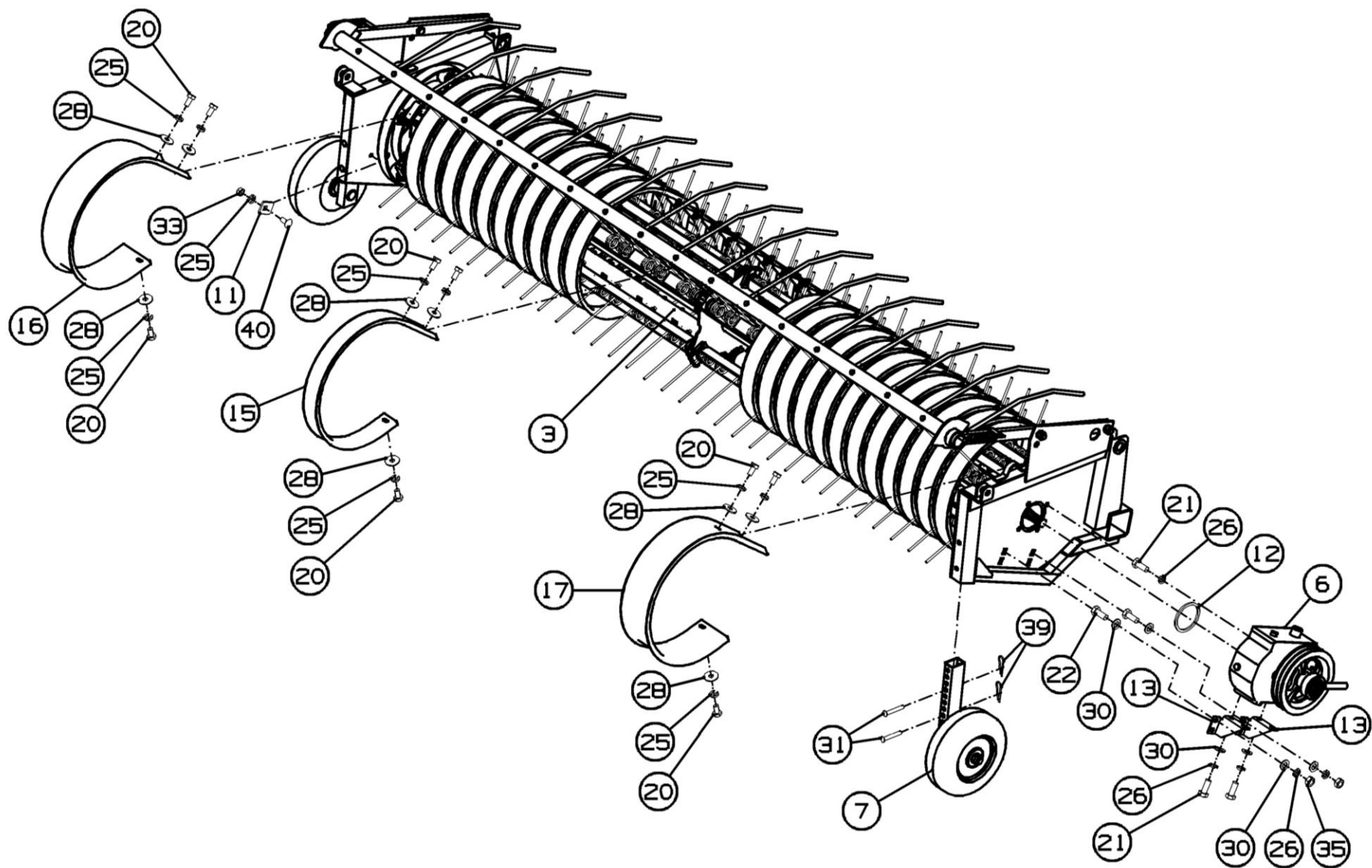
Рисунок 16 - Подборщик РСМ - 100.72.02.000Д
