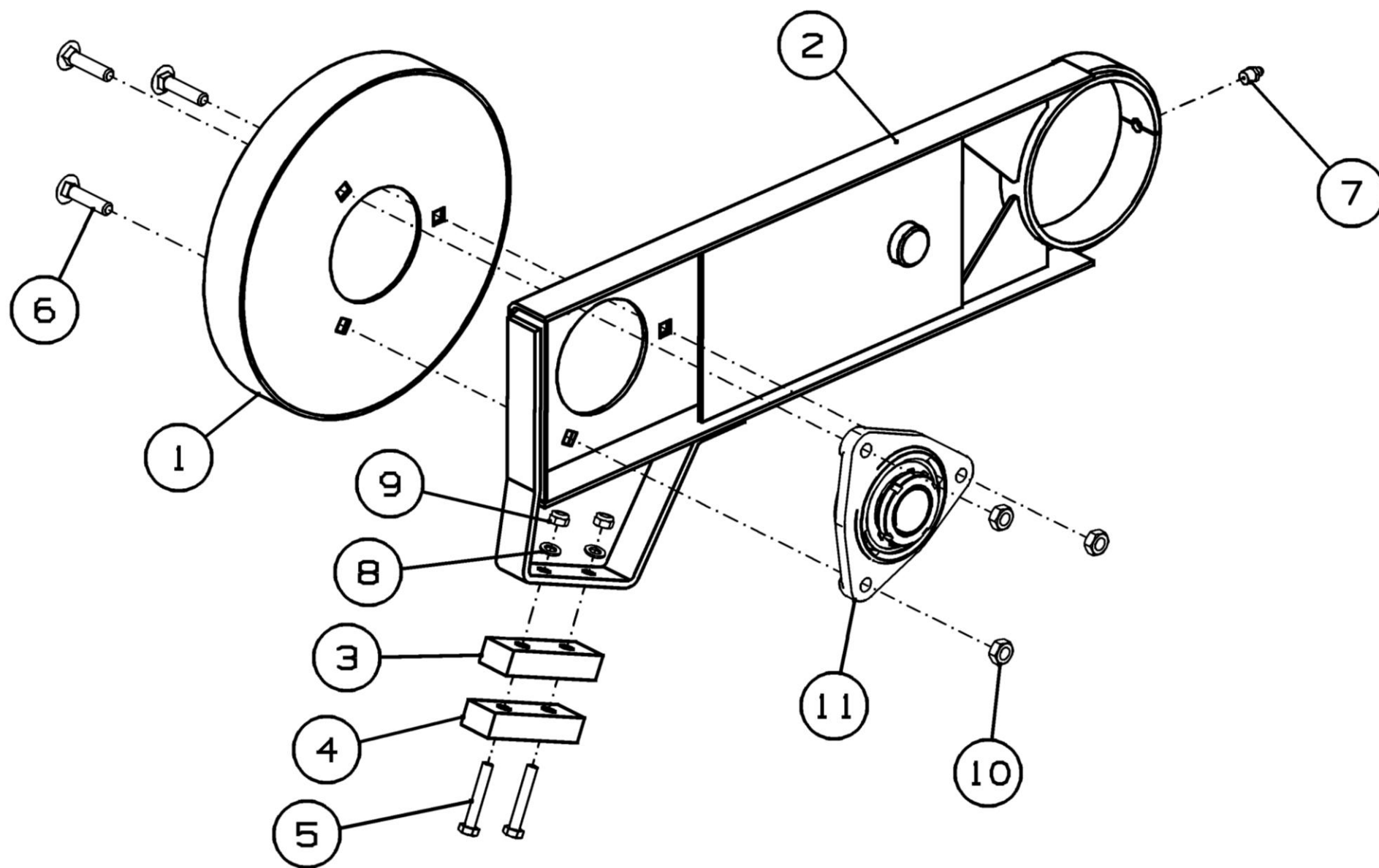
Рисунок 8 - Рычаг МСМ - 100.72.01.780
