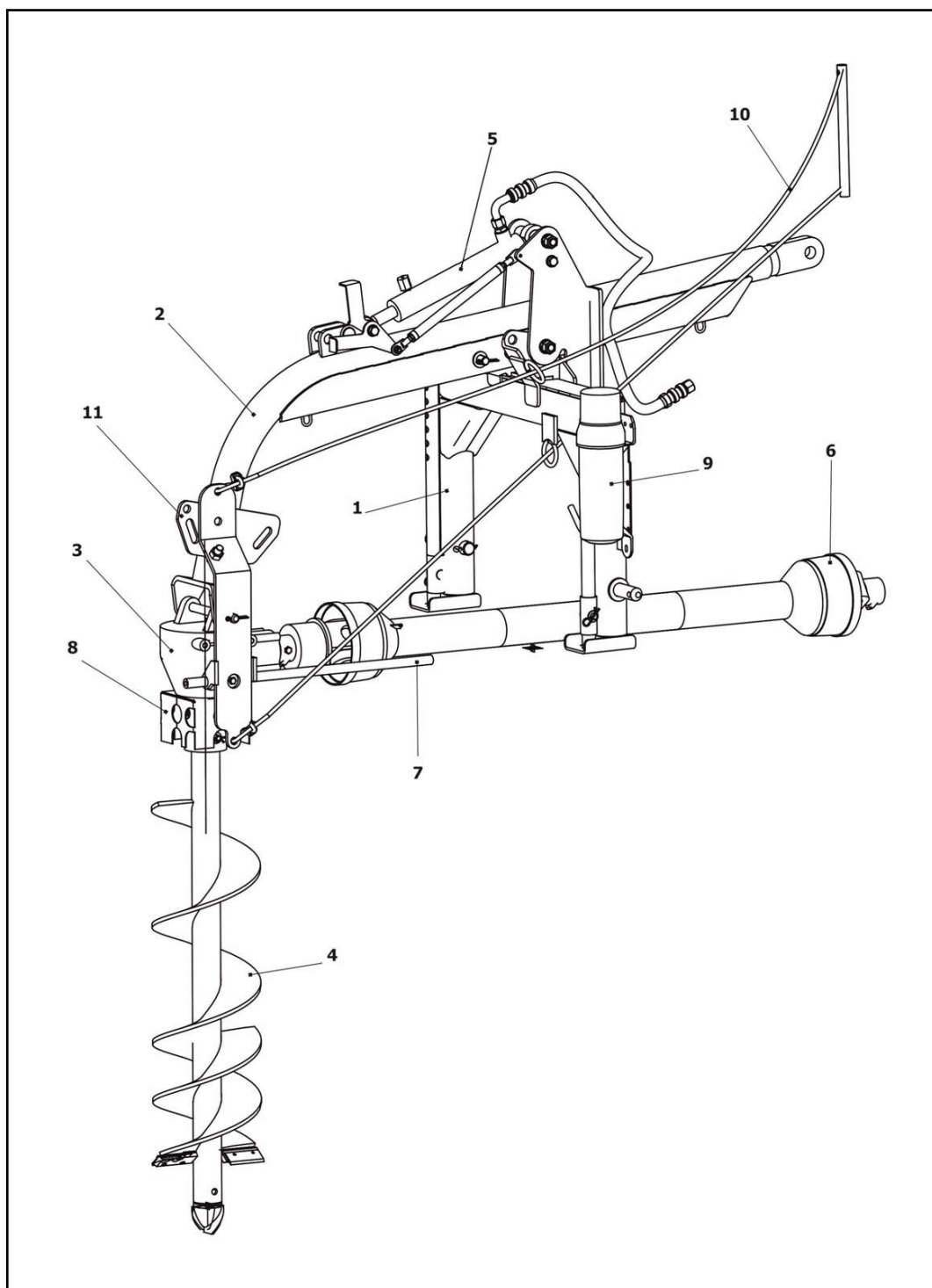
1 – Навеска; 2 – Штанга; 3 – Редуктор; 4 – Шнек; 5 – Гидрозаглубитель; 6 – Карданный вал; 7 – Ручка; 8 – Кожух; 9 – Тубус; 10 – Канат; 11 – Фиксатор
