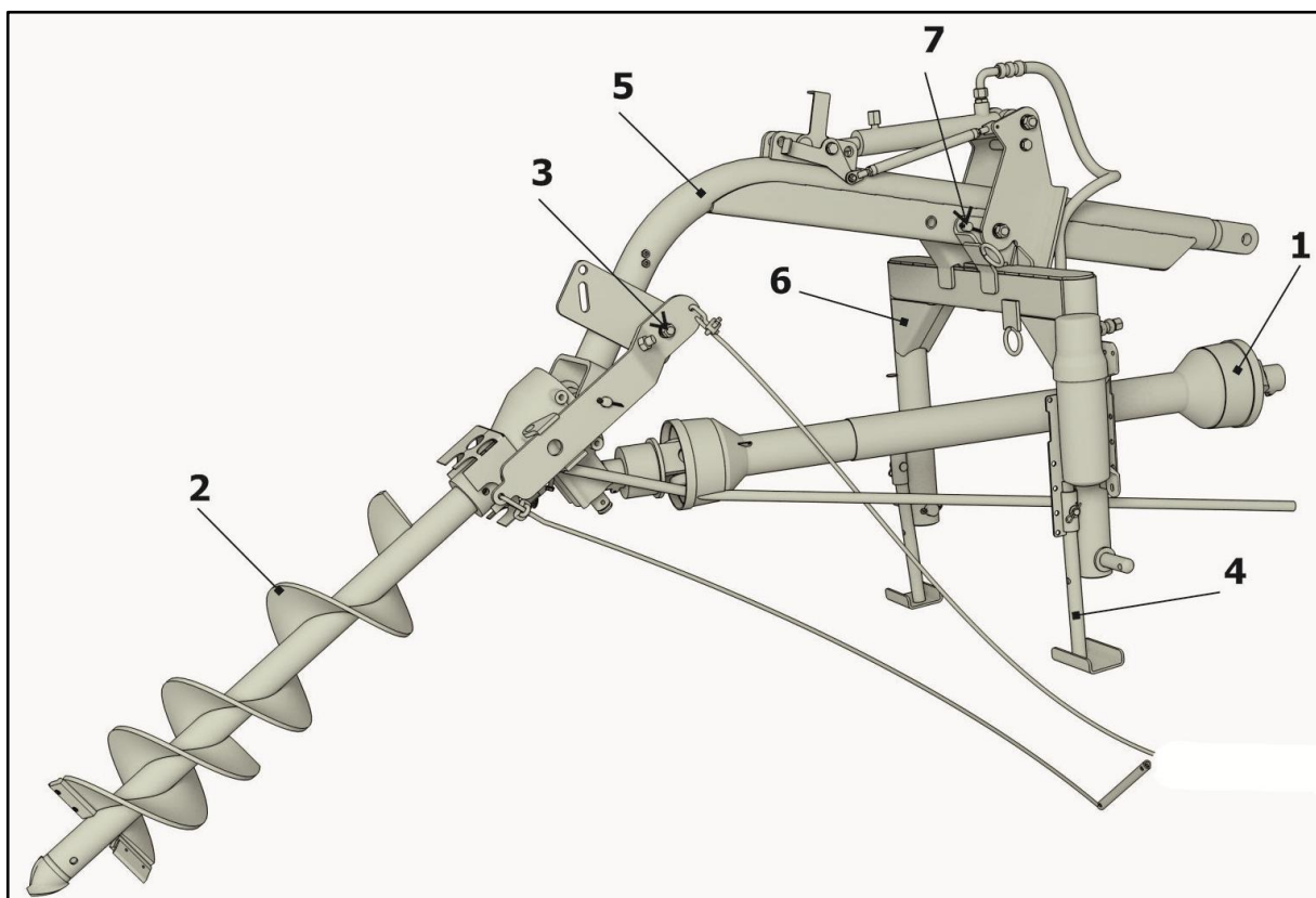
1 – Карданный вал; 2 – Шнек; 3 – Болтокрепеж; 4 – Опора; 5 – Штанга; 6 – Навеска; 7 – Ось Рисунок 6.1 – Подготовка бура к хранению
