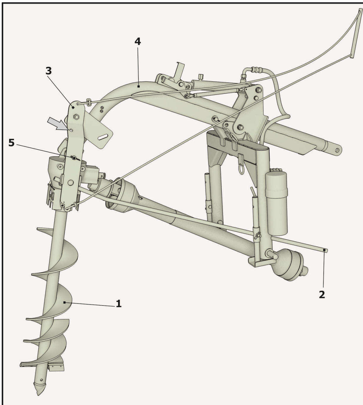
1 – Шнек; 2 – Ручка; 3 – Фиксатор; 4 – Штанга; 5 – Болтокрепеж Рисунок 5.4 – Транспортное положение бура
