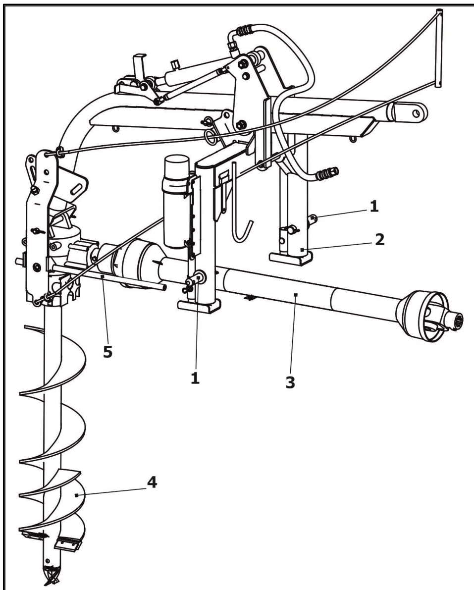
1 – Ось; 2 – Навеска; 3 – Карданный вал; 4 – Шнек; 5 – Ручка
