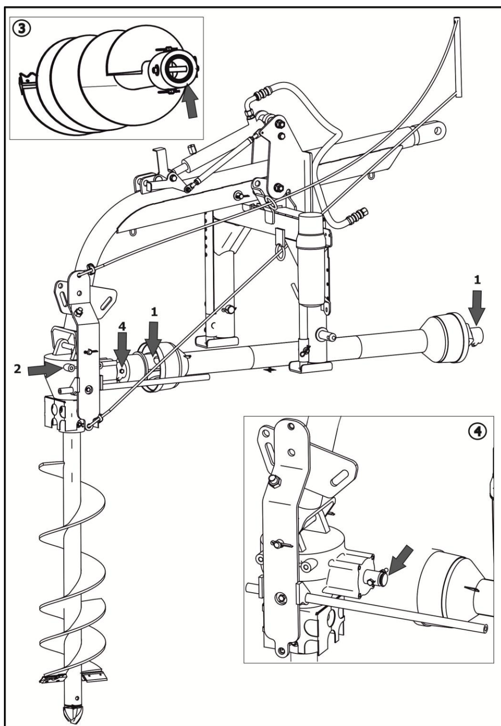
Рисунок 6.3 – Точки смазки бура БШ-230
