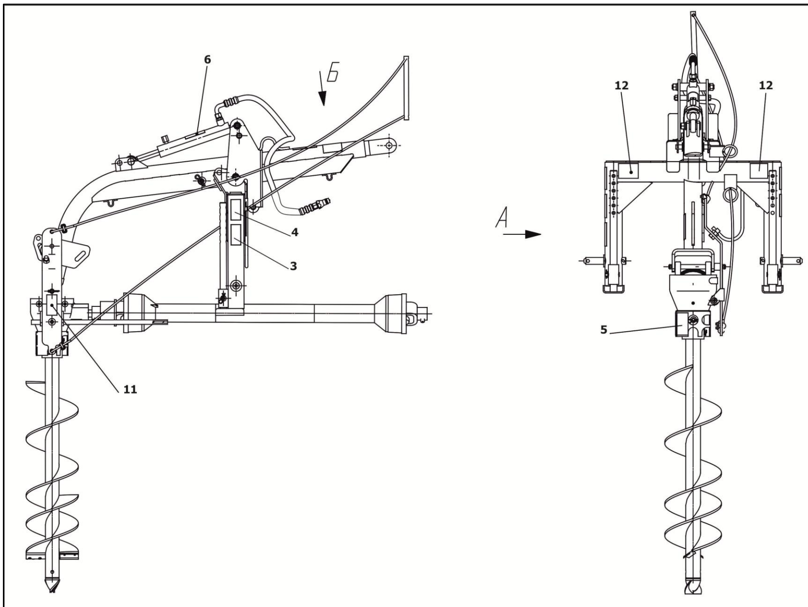
Рисунок 4.1 – Месторасположение табличек и аппликаций (Лист 1 из 2)
