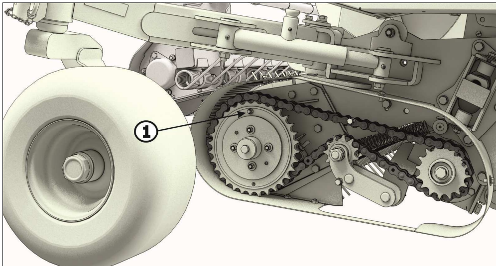
1-срезной болт
