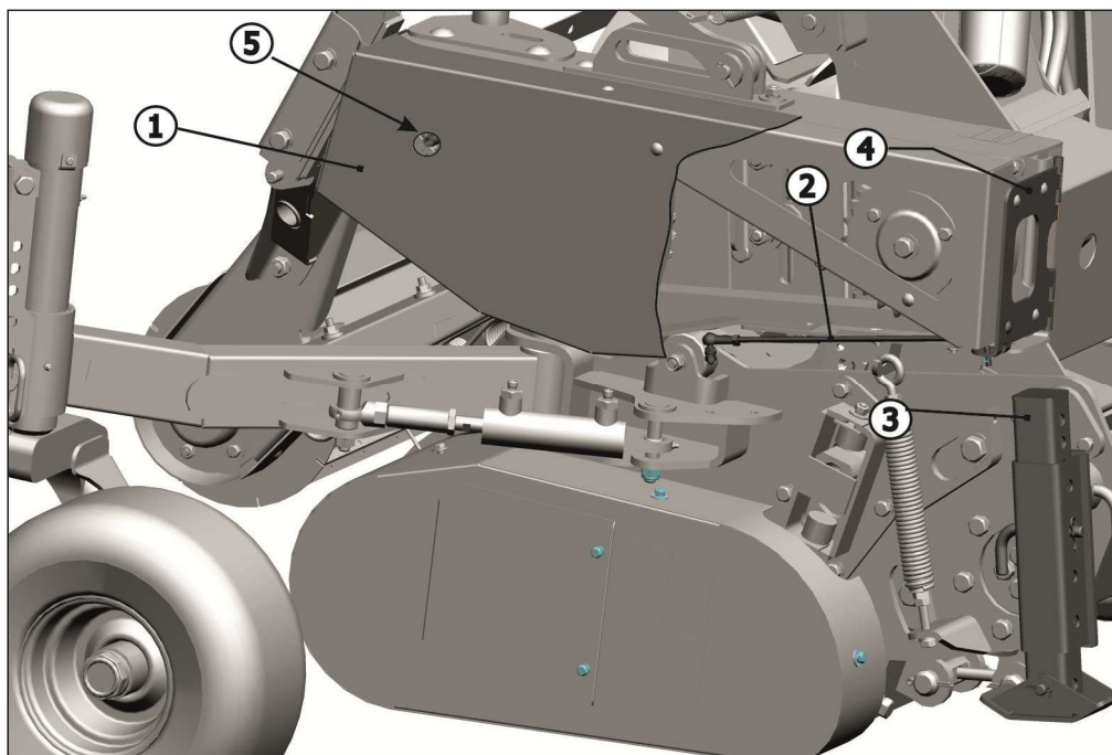
1 - щиток; 2-тяги; 3 - опора; 4 - петли; 5 - замок
