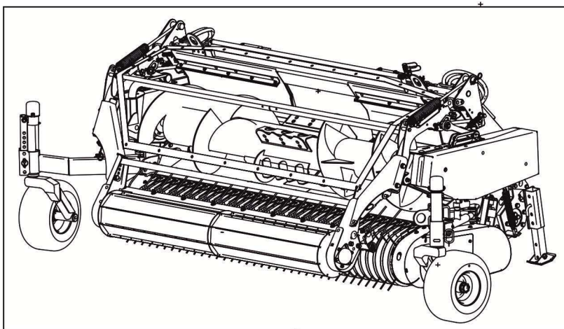
Рисунок 1.1 – Подборщик кормоуборочный ПК-432 "For Up 400"
