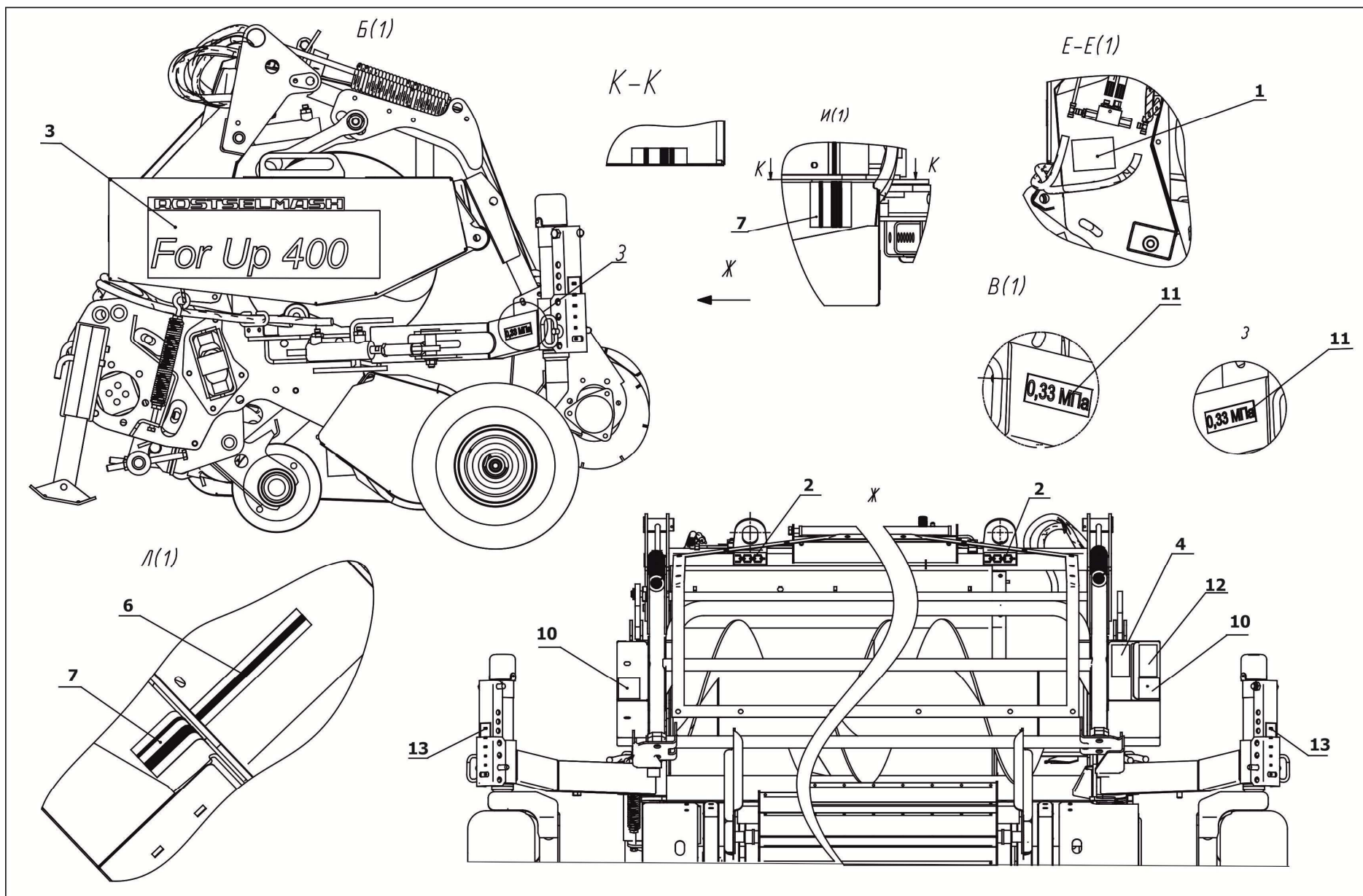
Рисунок 4.1 – Месторасположение аппликаций и табличек на подборщике
