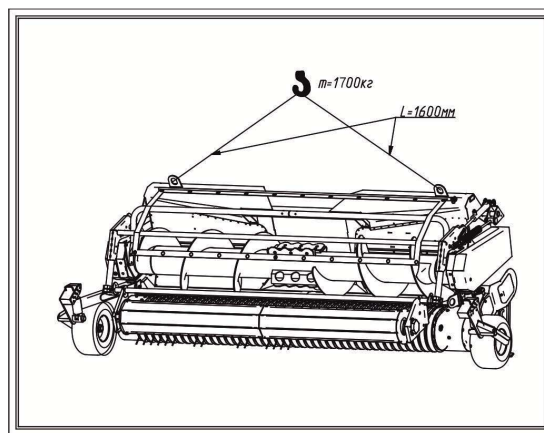
Рисунок 8.1 – Табличка «Схема строповки»
