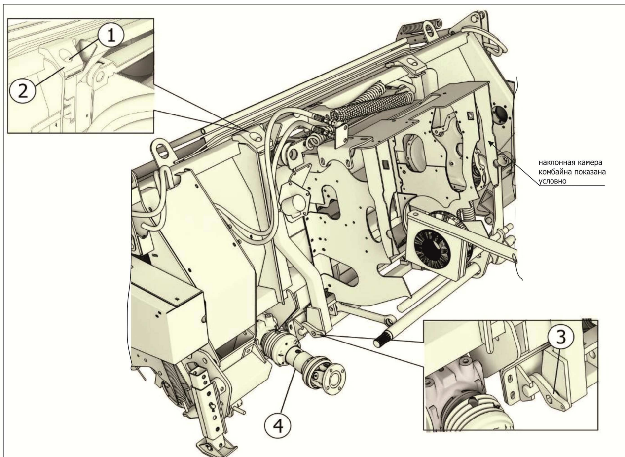
1—верхний фиксатор; 2—ловитель; 3—крюк; 4—вал карданный Рисунок 5.4 – Навеска подборщика на комбайн марок РСМ-200
