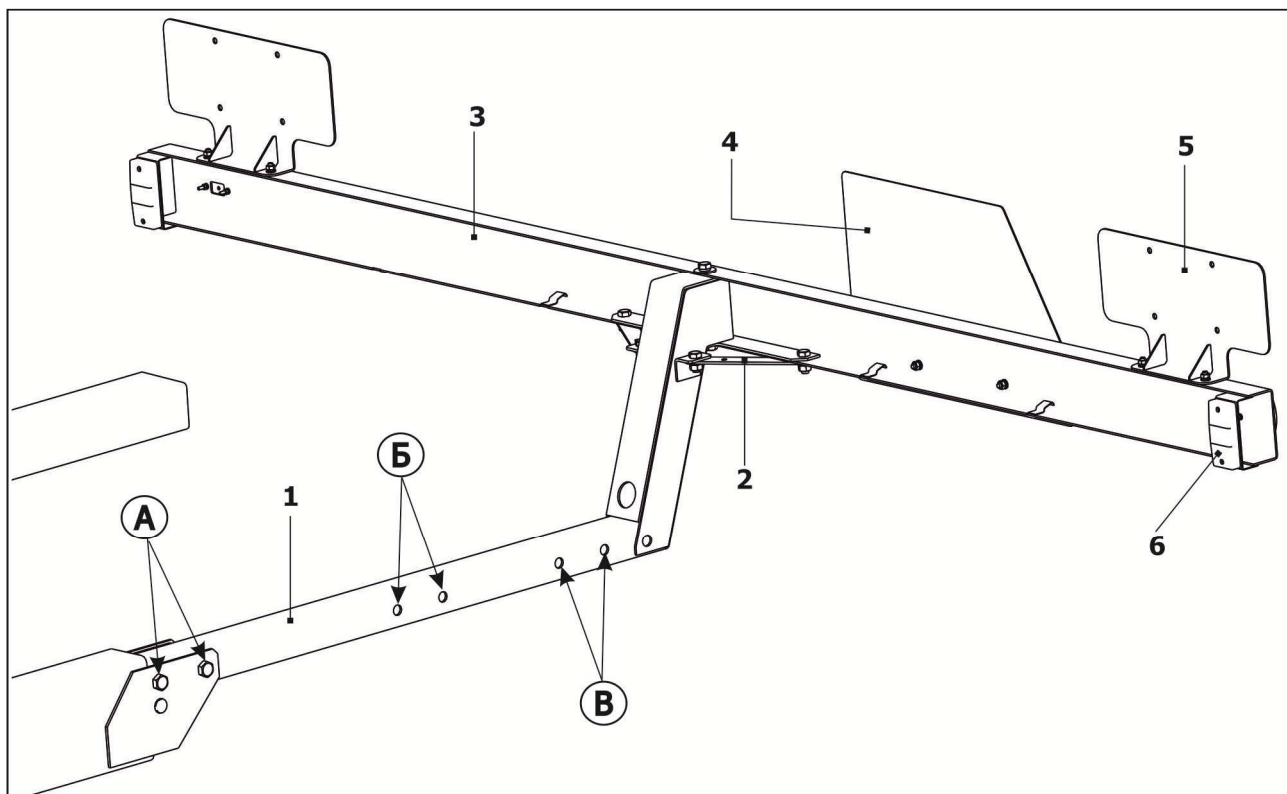
1 - балка; 2 - пластина; 3 - панель; 4 - знак; 5 - экран; 6 - передний фонарь А - отверстия для крепления жатки с шириной захвата 7 - 9 м; Б - отверстия для крепления жатки с шириной захвата 6 м; В - отверстия для крепления жатки с шириной захвата 5 м Рисунок 2.8 – Кронштейн для крепления фонарей
