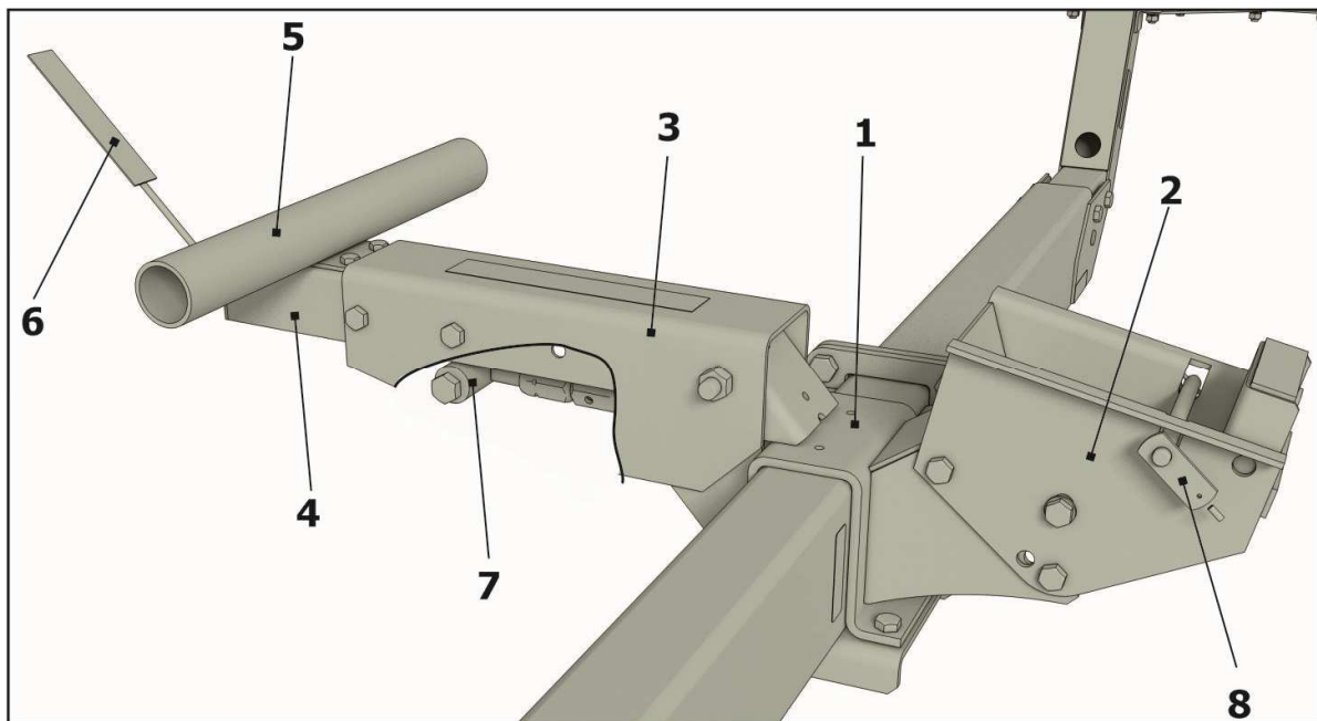
Рисунок 2.12 – Опора ППА-700.12.000
