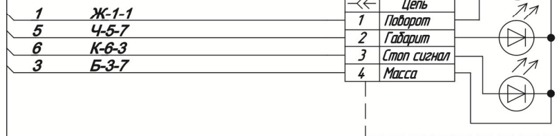
Фонарь задний левый
