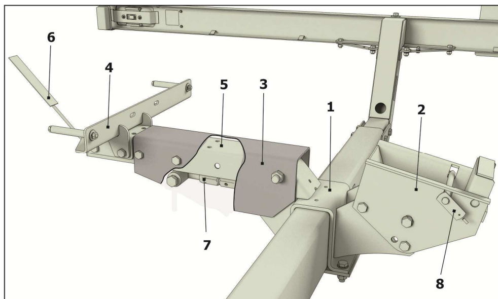
1 - основание; 2, 3, 4 - кронштейн; 5 - ложемент; 6 - ориентир; 7 - гайка стяжная; 8 - фиксатор Рисунок 2.14 – Опора ППА-700.12.000А
