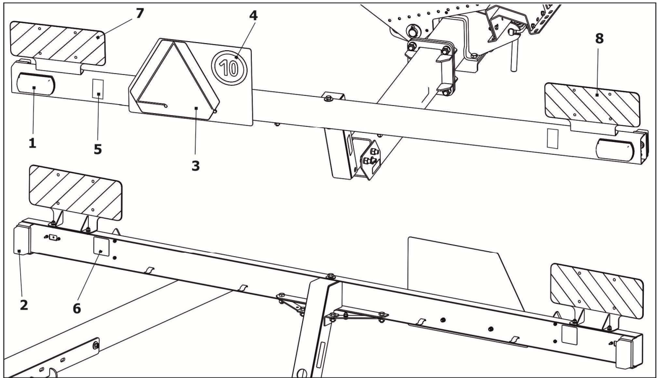
1 - фонарь задний; 2 - передний фонарь; 3 - аппликация «Тихоходное транспортное средство»; 4 - аппликация «Знак ограничения скорости»; 5 - аппликация «Световозвращатель красный»; 6 - аппликация «Световозвращатель белый»; 7, 8 - габарит Рисунок 2.9 – Средства сигнализации приспособления
