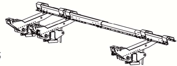
1, 2, 3 - опора; 4 - желоб опорный; 6 - желоб внутренний; 8 - надставка Рисунок 5.7 - Схема установки опор и желобов на ППА-700-05 (жатка 081.27 с ш/з 9 м пружинное копирование)
