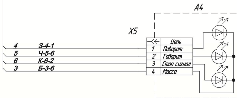
Фонарь задний правый
