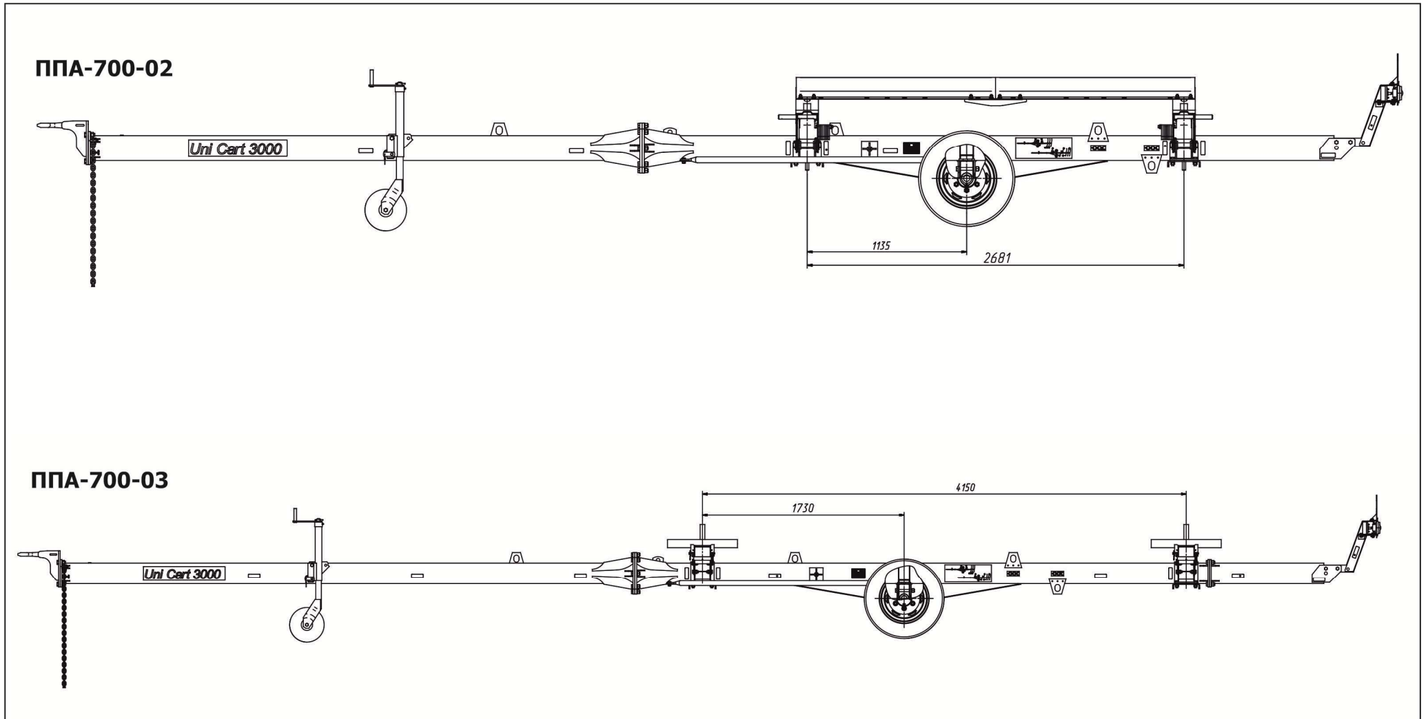
Рисунок 5.4 – Схема установка опор на приспособления ППА-700-02 и ППА-700-03
