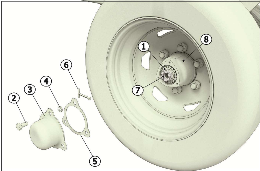
Рисунок 6.1 – Регулировка осевого зазора в подшипниках ступицы колеса
