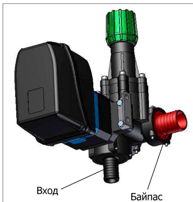
Рисунок 3.12 – Главный клапан
