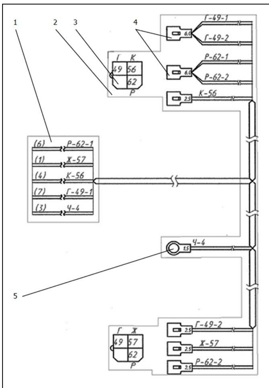
Рисунок 3.20 — Схема жгута задних фонарей
