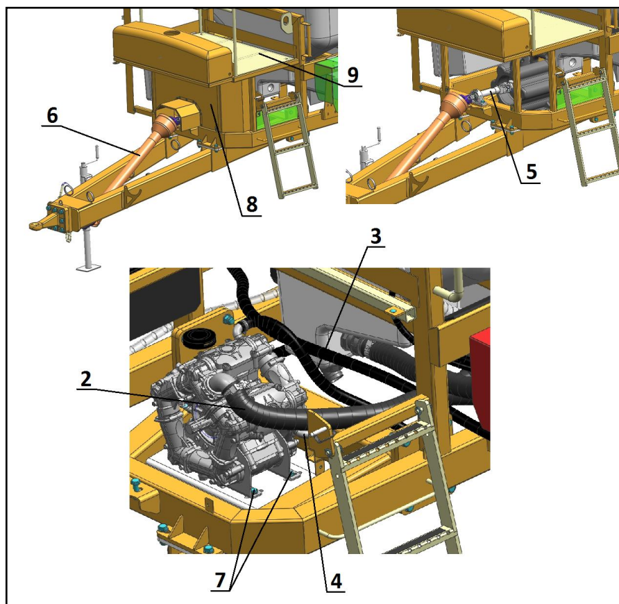
1 – Насос; 2, 3, 4 – Шланги системы распыления; 5 – Вал промежуточный; 6 – Карданный вал; 7 – Болтокрепёж насоса; 8 – Щиток центральный; 9 – Настил Рисунок 7.3 – Демонтаж насоса
