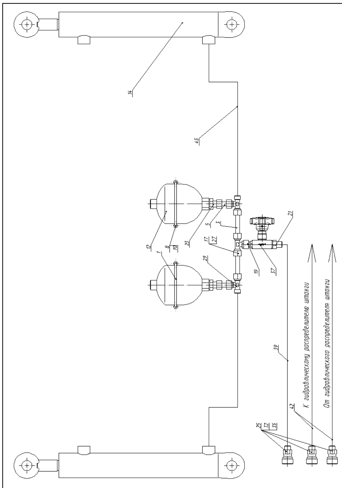
Рисунок Б.1 – Схема гидравлическая шасси
