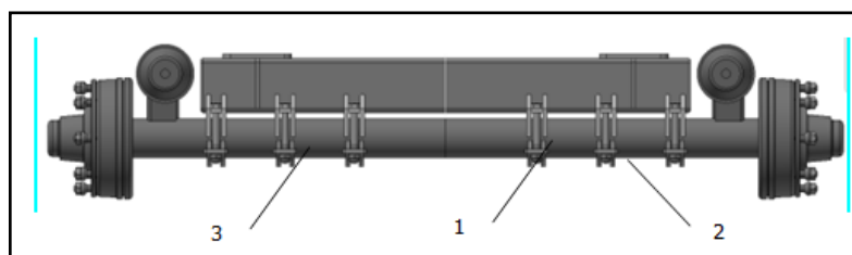
1 – Стягивающий болт; 2 – Хомут; 3 – Полуось. Рисунок 5.3 – Мост (колеса условно сняты)
