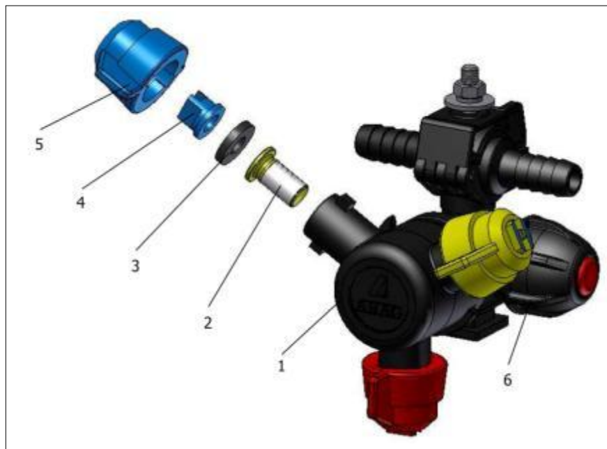
1 – Соплодержатель; 2 – Фильтр; 3 – Прокладка; 4 – Форсунка; 5 – Колпачок; 6 – Отсечной клапан Рисунок 3.11 – Соплодержатель
