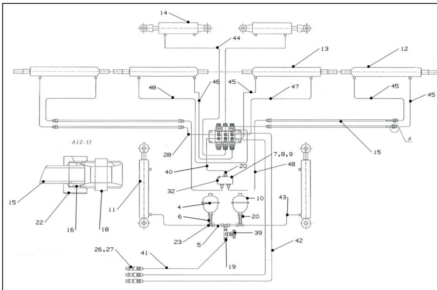
Рисунок В.1 – Схема гидравлическая управления штангой пятизвенной (Лист 1 из 3)
