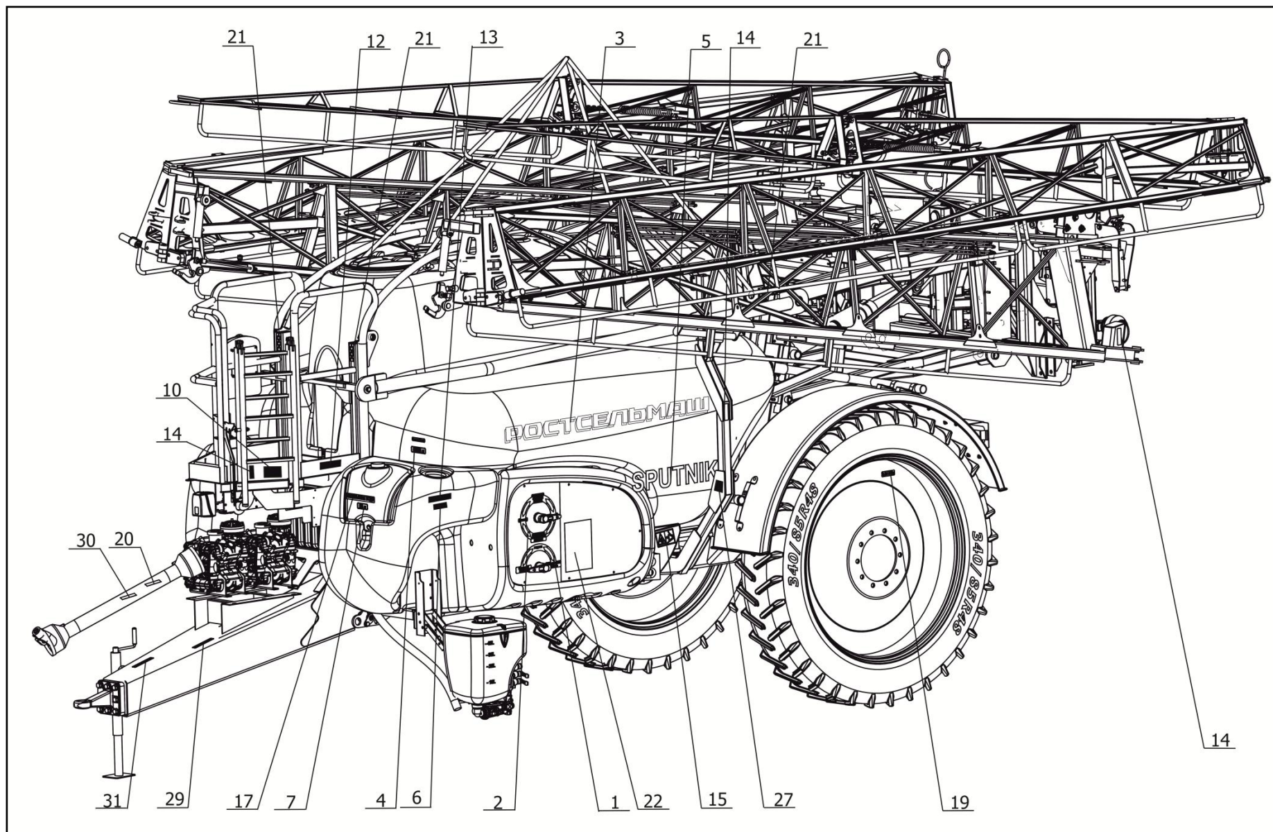
Рисунок 4.1 – Месторасположение аппликаций и табличек (Лист 1 из 3)
