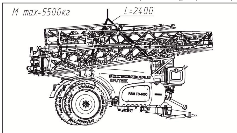
Рисунок 8.1 – Схема строповки
