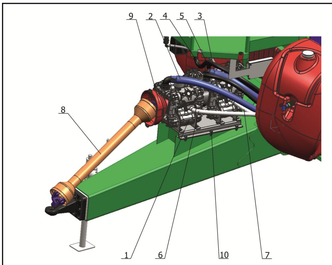
1 – Насос; 2, 3, 4, 5, 6, 7 – Шланги системы распыления; 8 – Вал карданный; 9 – Кожух шлицевого хвостовика насоса; 10 – Болтокрепёж насоса
