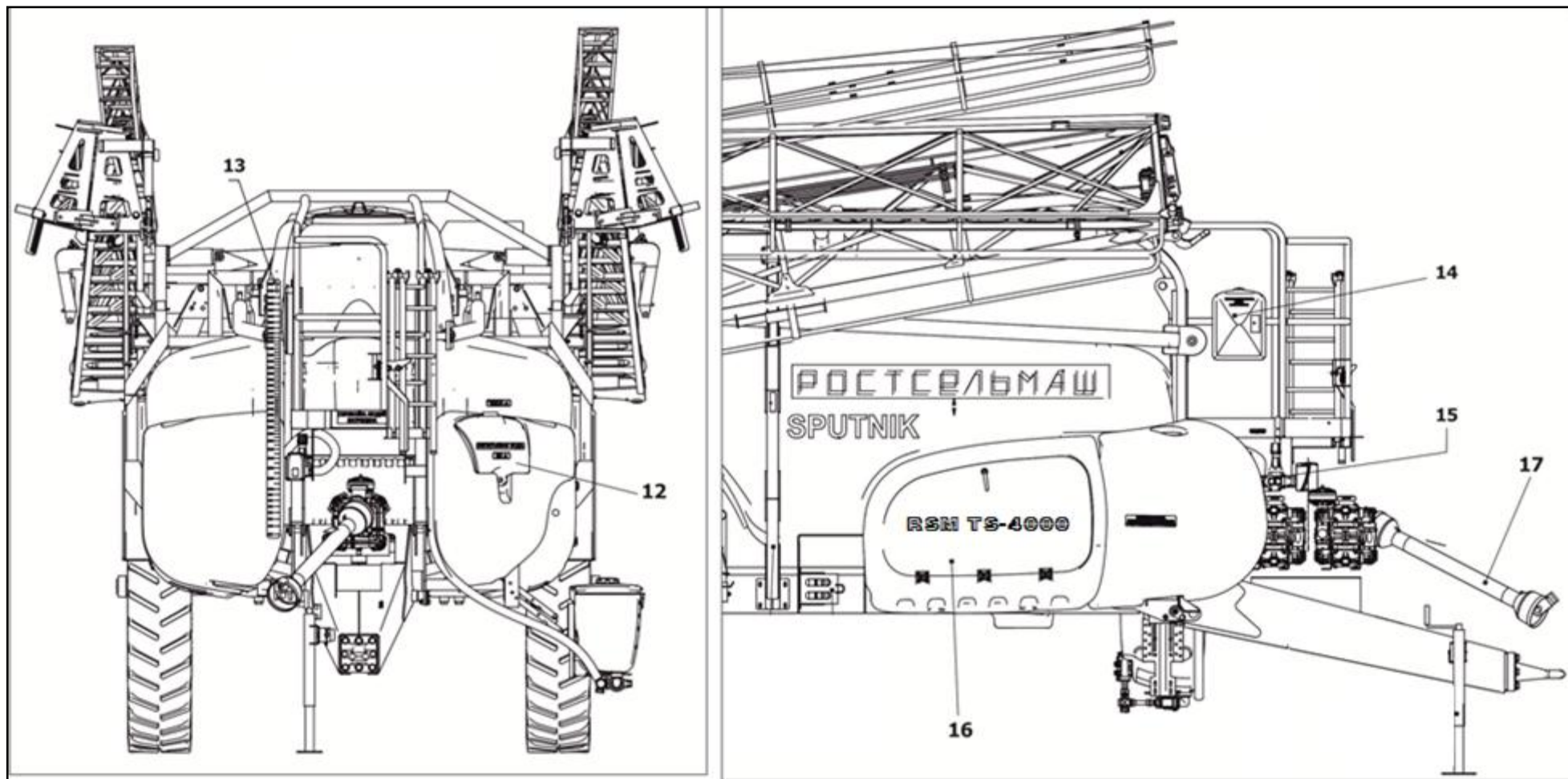
Рисунок 3.1.1 – Общий вид опрыскивателя
