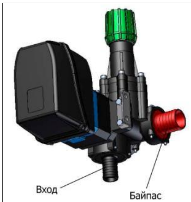
Рисунок 3.10 – Главный клапан
