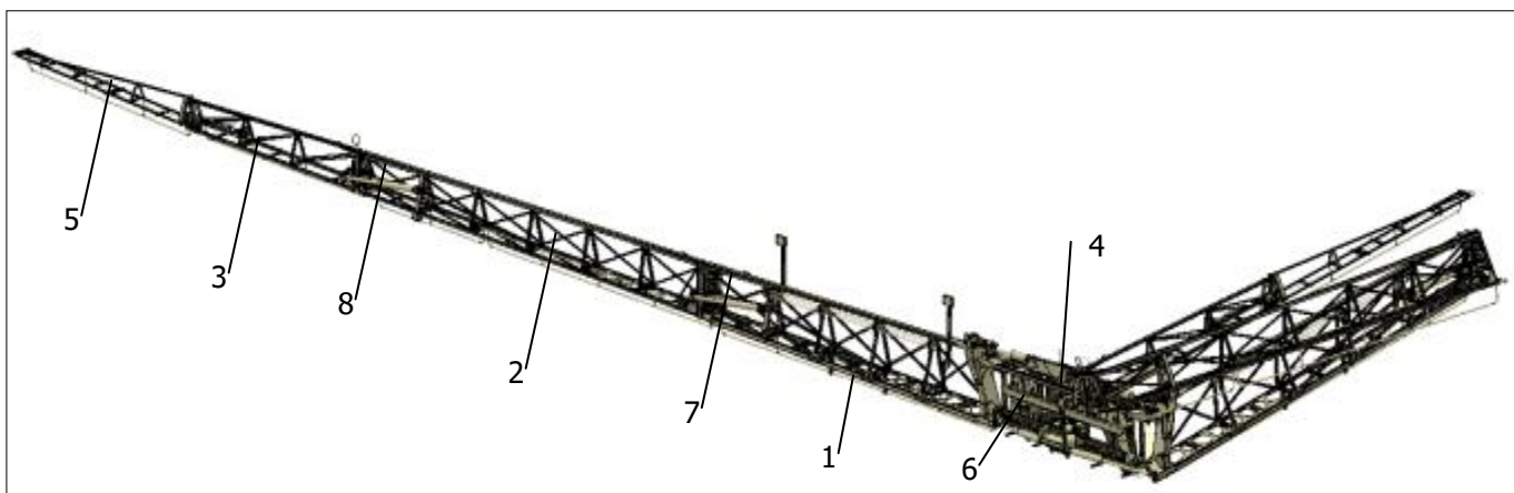
Рисунок 3.2 – Центральное звено семизвенной штанги
