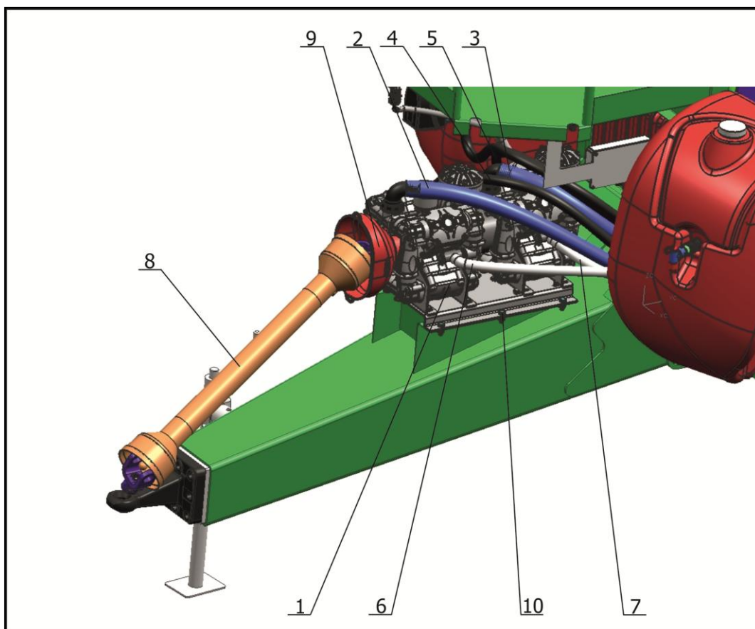
1 – Насос; 2, 3, 4, 5, 6, 7 – Шланги системы распыления; 8 – Вал карданный; 9 – Кожух шлицевого хвостовика насоса; 10 – Болтокрепёж насоса
