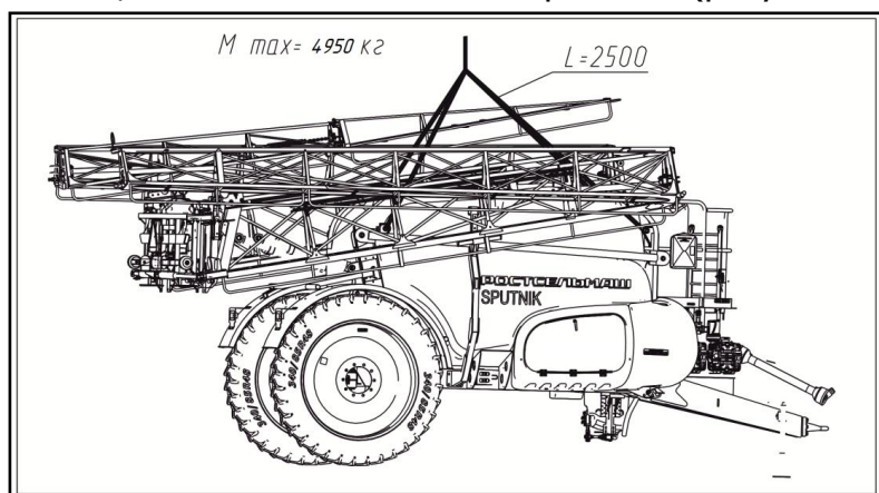
Рисунок 8.1 – Схема строповки
