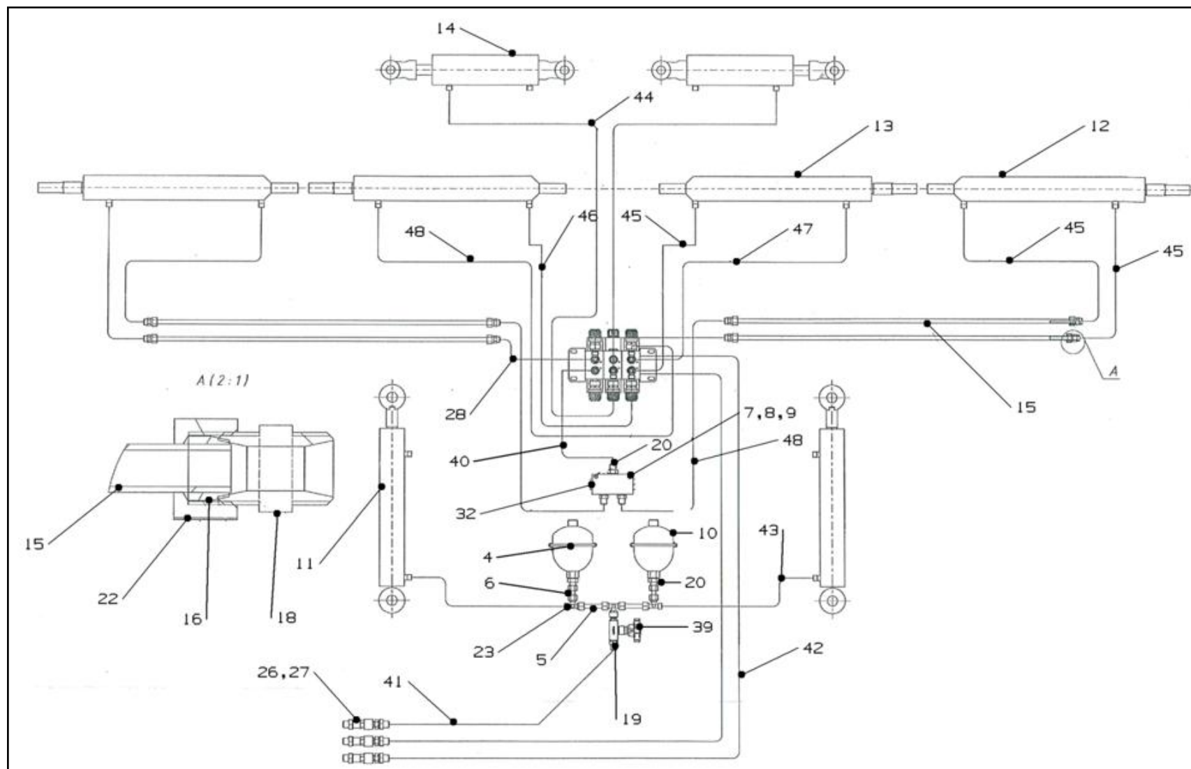
Рисунок В.1 – Схема гидравлическая управления штангой пятизвенной (Лист 1 из 3)
