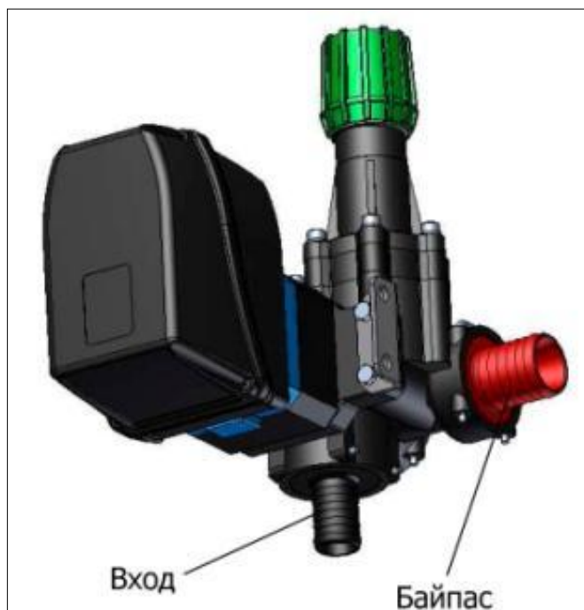
Рисунок 3.10 – Главный клапан
