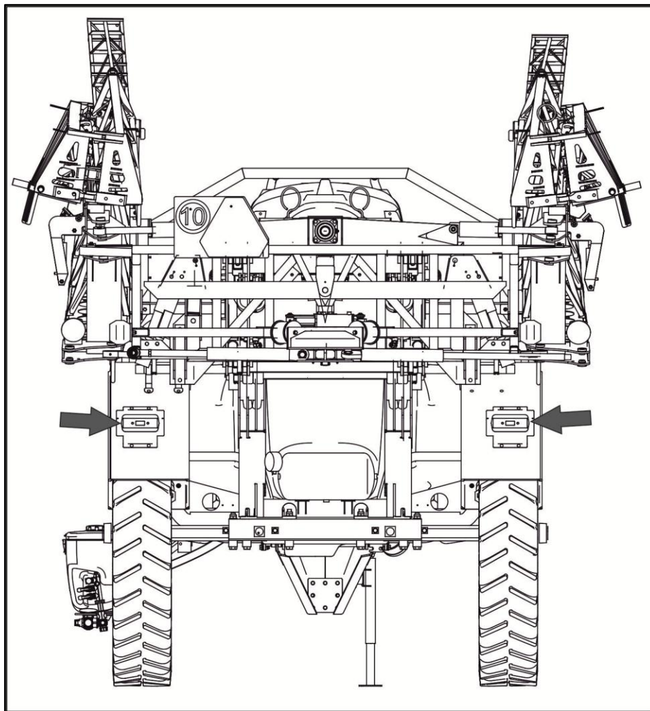
Рисунок 3.15 – Задние фонари
