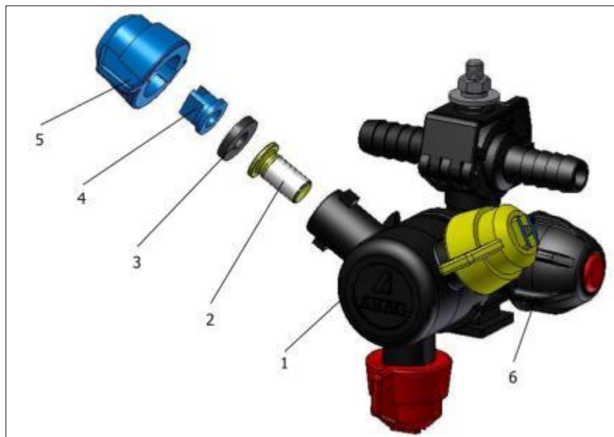
1 – Соплодержатель; 2 – Фильтр; 3 – Прокладка; 4 – Форсунка; 5 – Колпачок; 6 – Отсечной клапан Рисунок 3.11 – Соплодержатель
