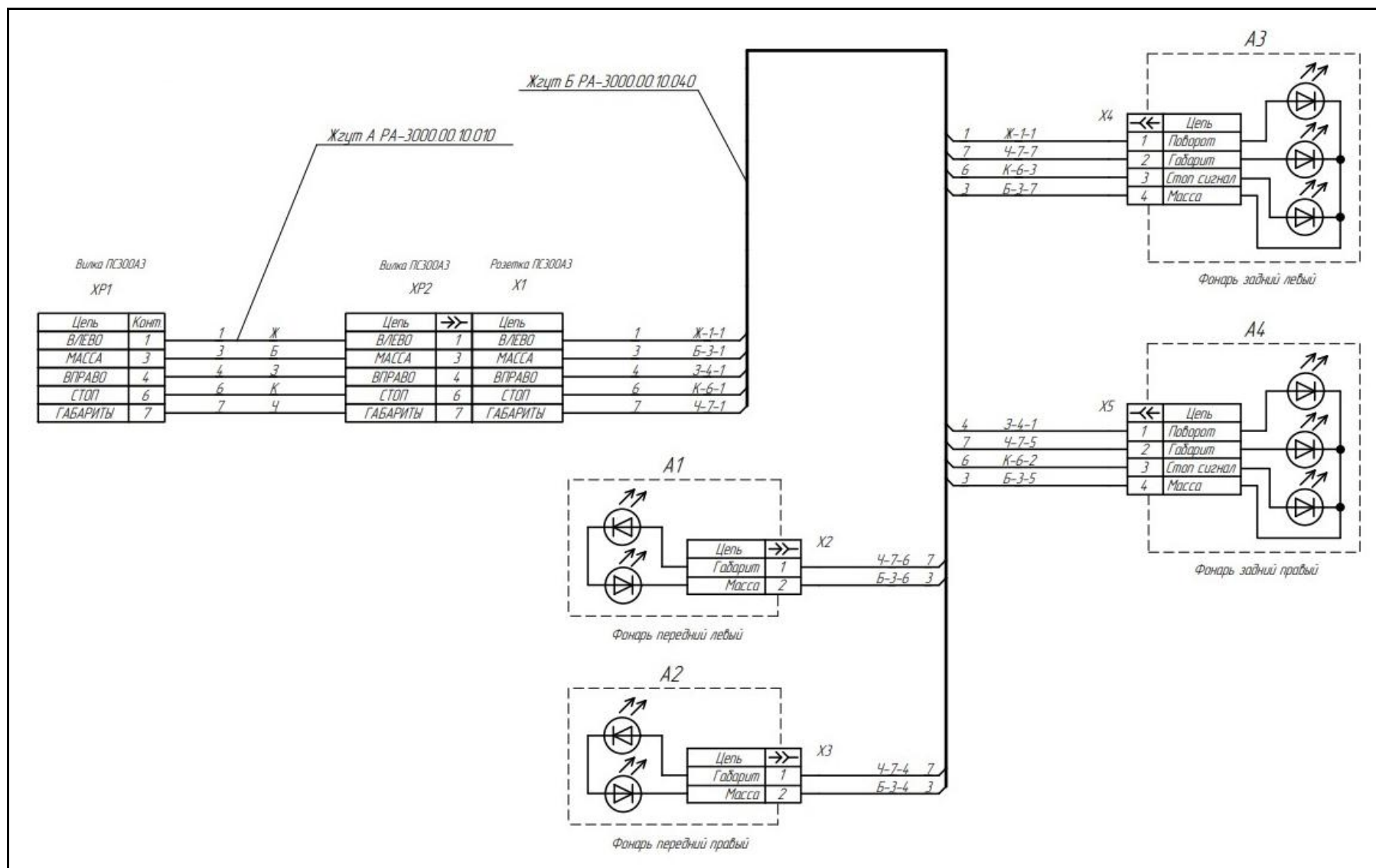
Рисунок Б.1 – Схема электрическая принципиальная
