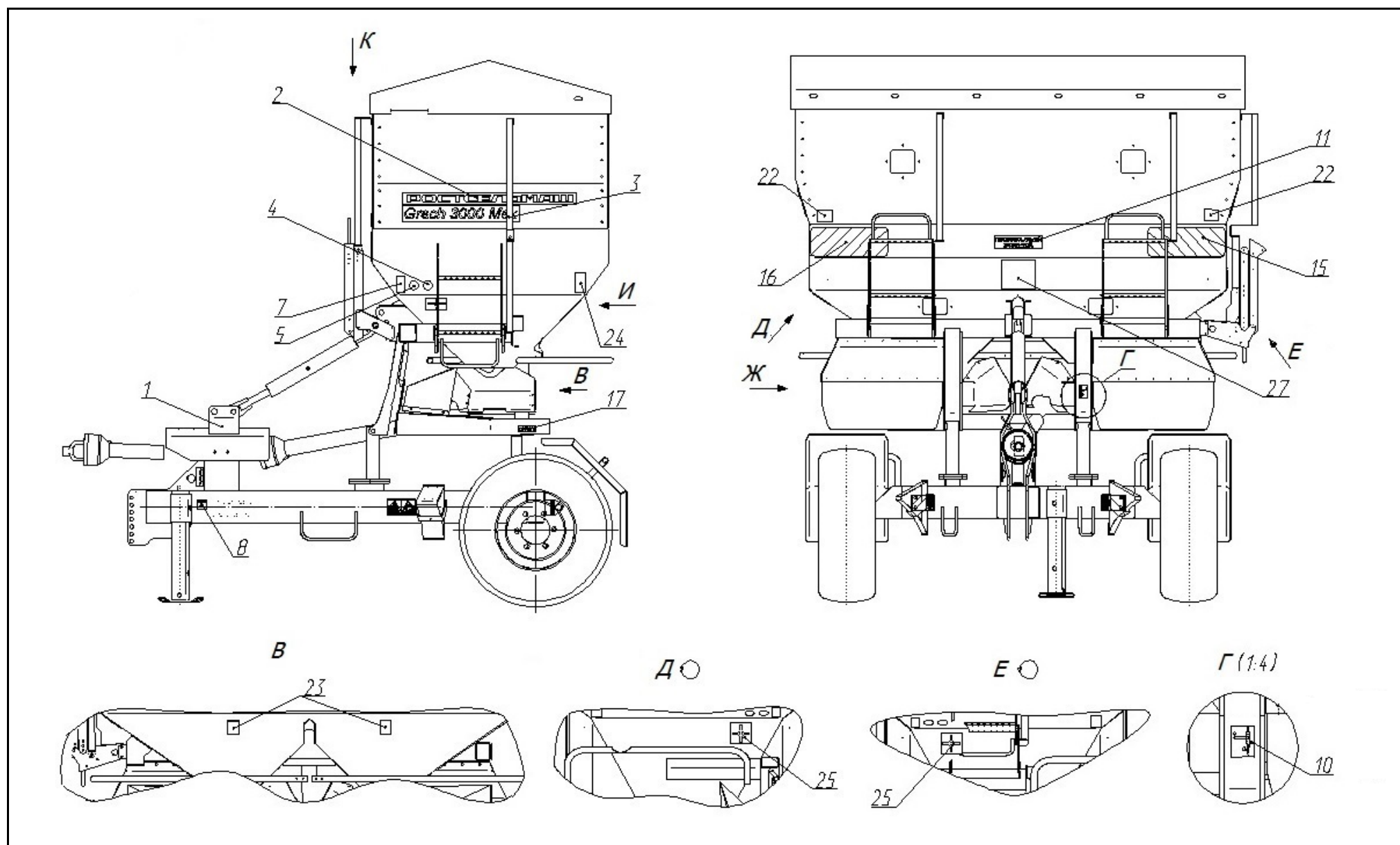
Рисунок 4.1 – Месторасположение табличек и аппликаций (Лист 1 из 3)
