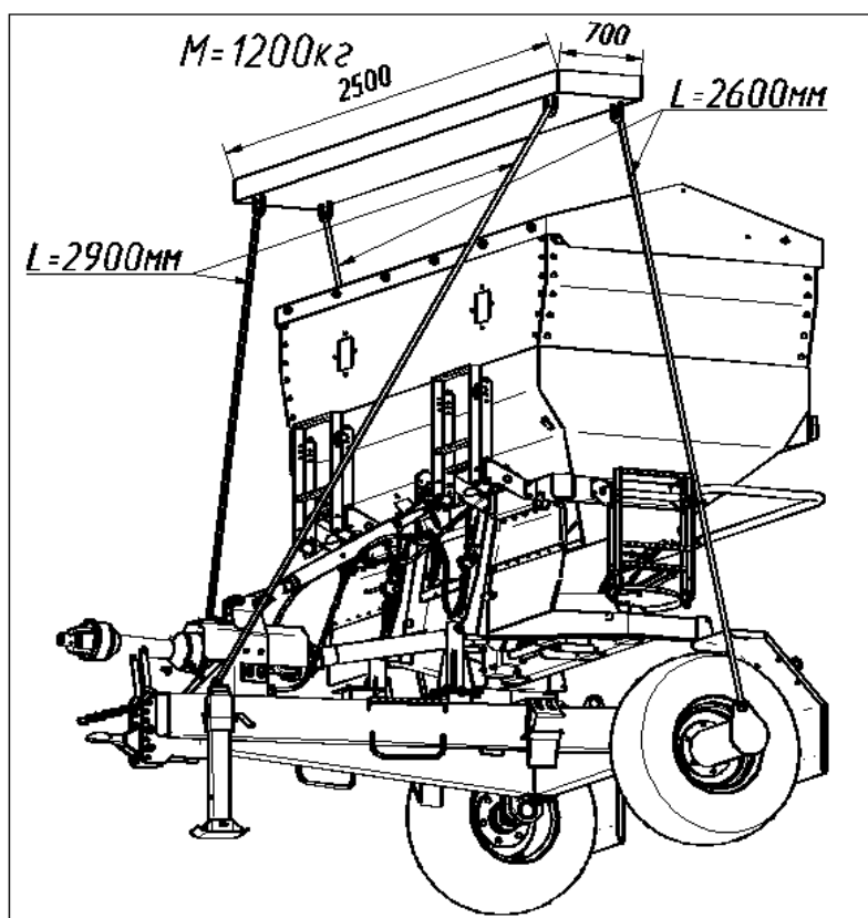
Рисунок 8.1 – Схема строповки
