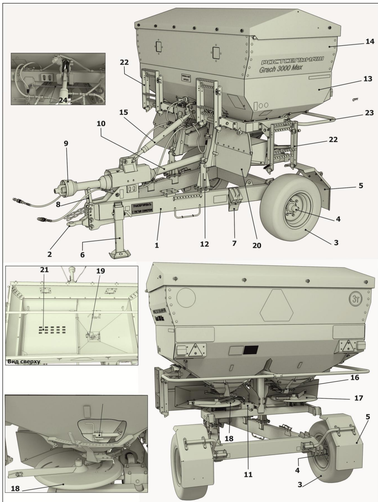
1 – Рама; 2 – Сница; 3 – Колесо; 4 – Ступица; 5 – Крылья; 6 – Домкрат; 7 – Упор противооткатный; 8 – Упор; 9 – Карданный вал с обгонной муфтой; 10 – Карданный вал; 11 – Редуктор; 12 – Стойка; 13 – Бункер; 14 – Надставка; 15 – Тяга; 16 – Механизм регулировки высева; 17, 18 – Диск разбрасывающий; 19 – Ворошилка; 20 – Брызговик; 21 – Решетка; 22 – Лестница; 23 – Ограждение; 24 – Чистик
