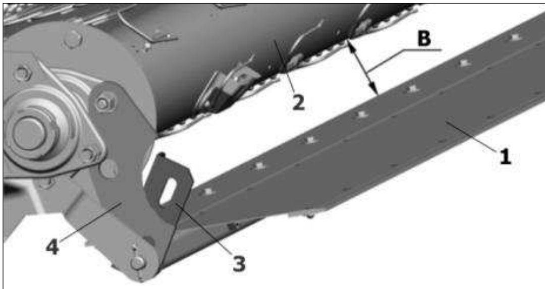
1 – Стеблесъемник; 2 – Вал задний; 3 – Угольник; 4 – Коромысло Рисунок 5.5 – Регулировка зазора между рабочей кромкой стеблесъемника и задним валом транспортера
