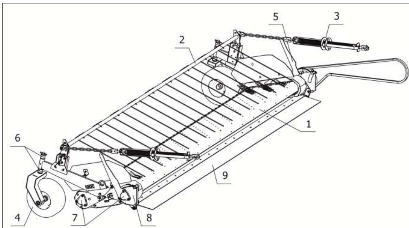
Рисунок 3.4 – Подборщик транспортный
