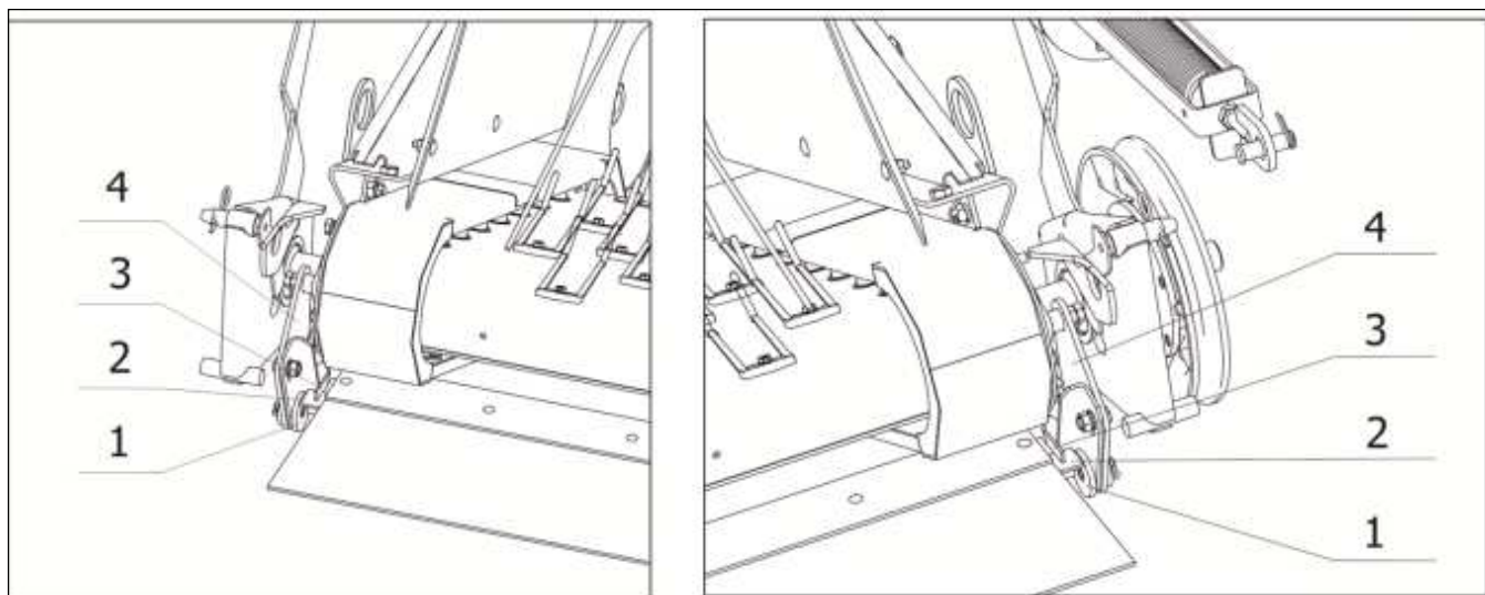
а) б) 1 – Цапфа; 2 – Упор; 3 – Уголок опорный; 4 - Коромысло Рисунок 5.7
