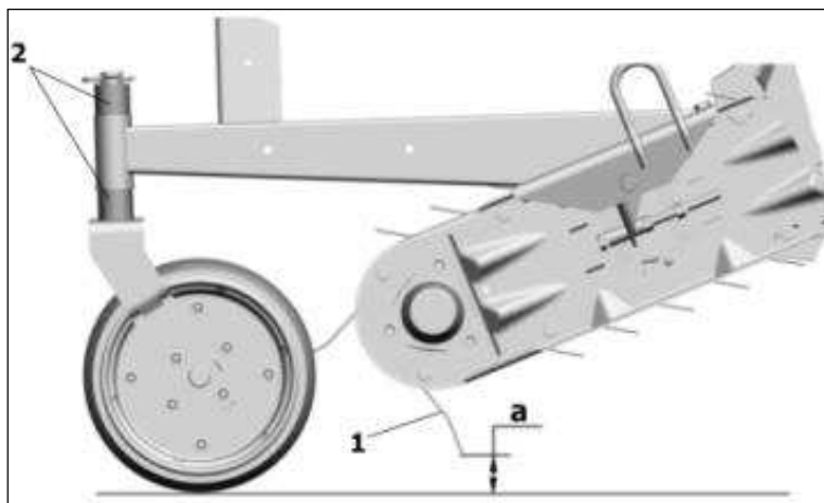
Рисунок 5.3 – Регулировка зазора между концами подбирающих пальцев и уровнем почвы
