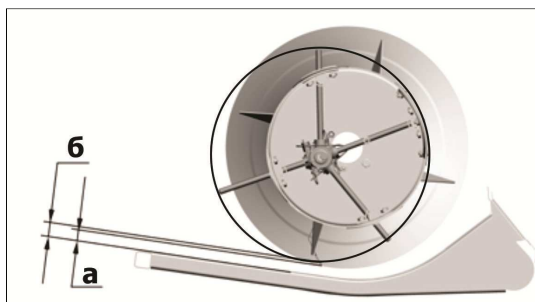
Рисунок 5.2 – Расположение шнека и его пальчикового механизма при работе платформы-подборщика
