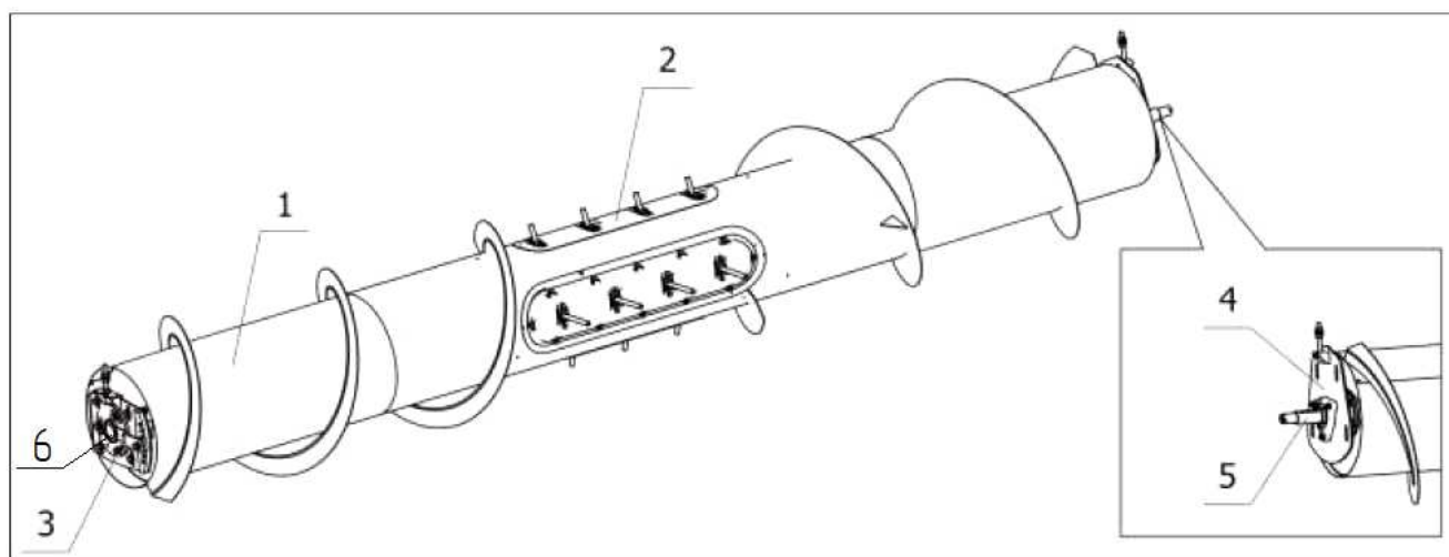
1 – Труба шнека; 2 – Пальчиковый механизм; 3 – Плита левая ЖСУ-900.01.01.120; 4 – Плита правая ПП-342R.01.00.010; 5 – Цапфа; 6 – Ось шнека правая
