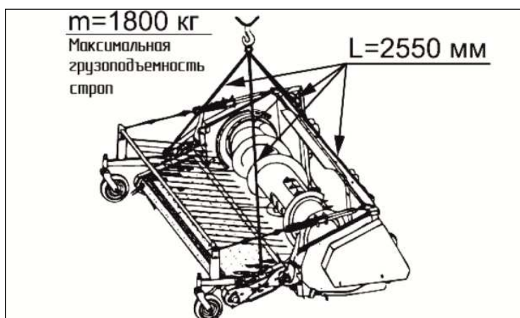
Рисунок 9.1 – Табличка «Схема строповки»
