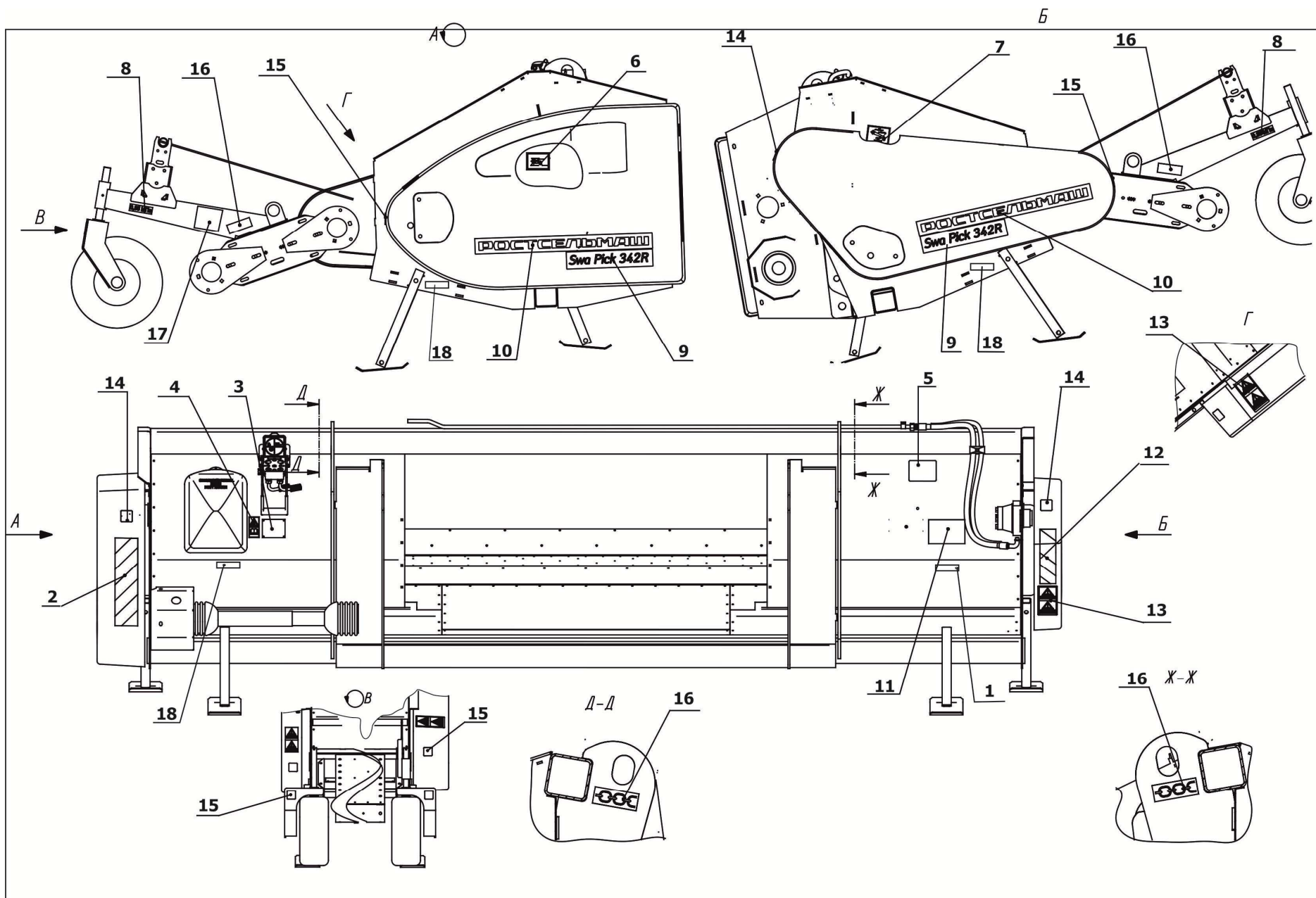
Рисунок 4.1 – Месторасположение табличек на платформе-подборщике
