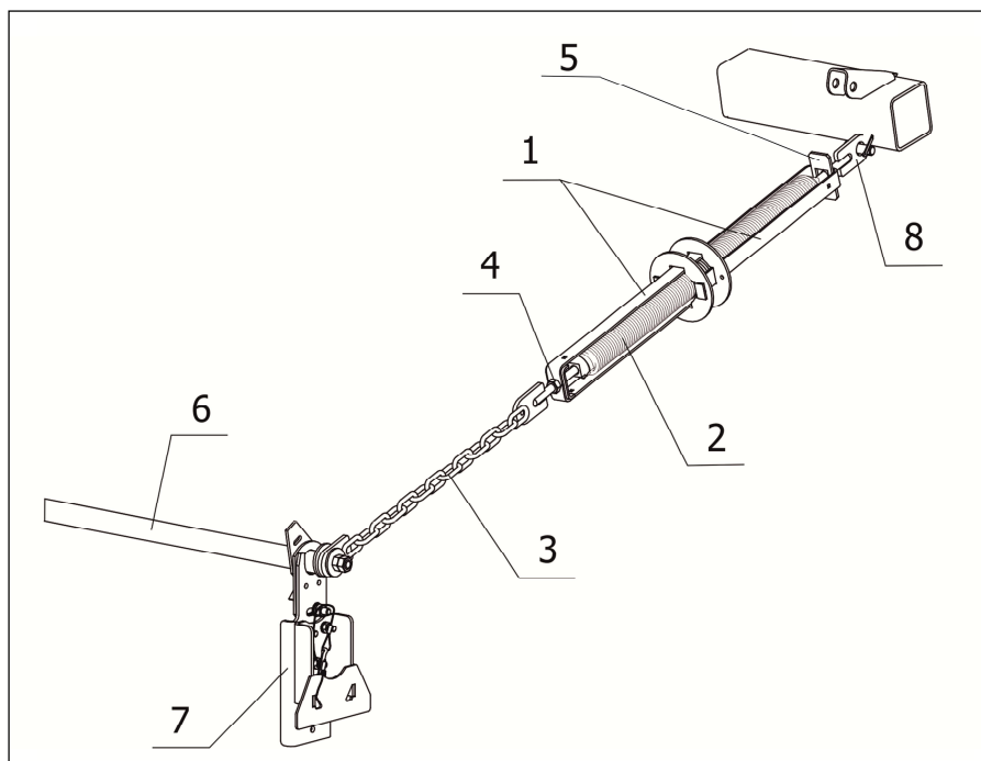
1 – обоймы; 2 – пружина; 3 – тяга; 4 – гайка регулировочная; 5 – фиксатор; 6 – балка нормализатора; 7 – стойка; 8 – растязка
