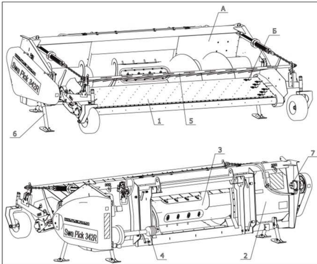
Рисунок 3.1 – Состав платформы-подборщика
