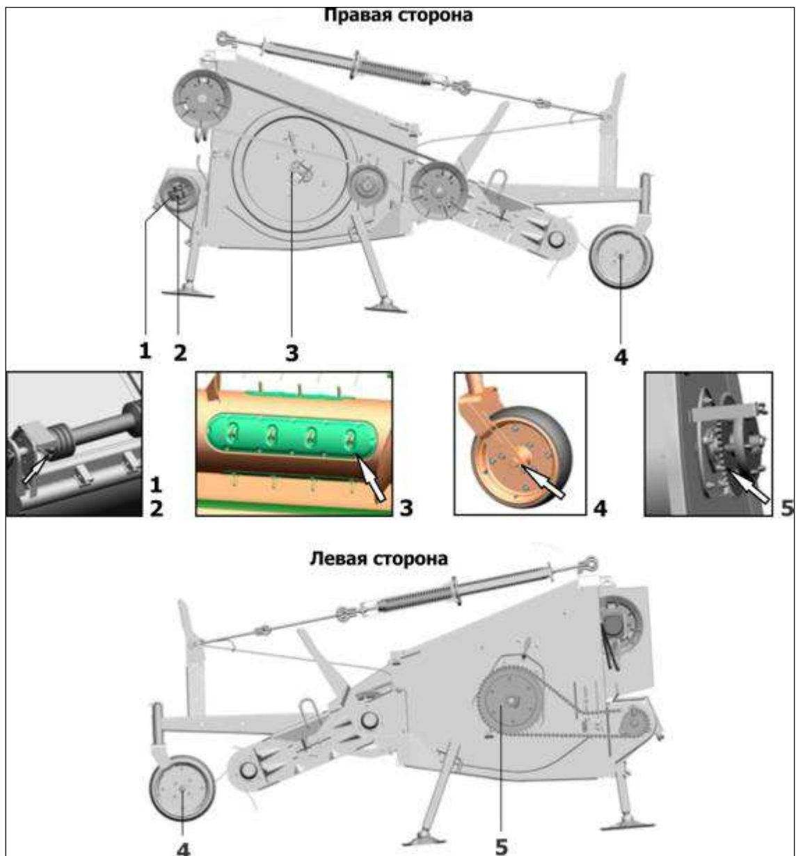
Рисунок 6.1 – Объекты смазки платформы-подборщика
