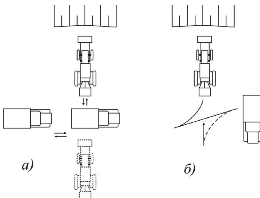
Рис. 9 Схемы взаимодействия погрузчика с транспортным средством
