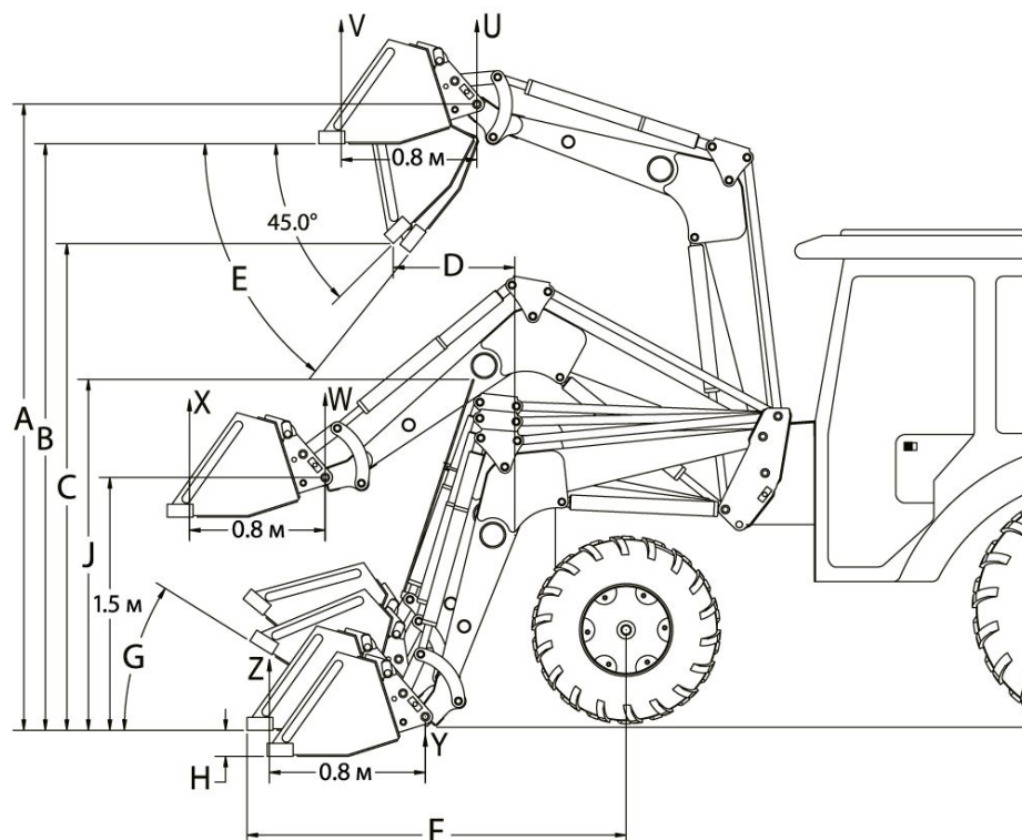
Рис. 2 Технические данные погрузчика
