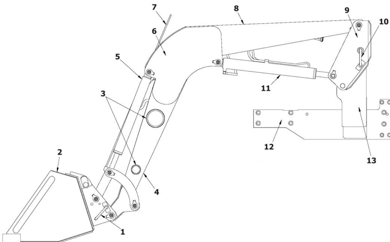
Рис. 1 Погрузчик ПФН-3,0
