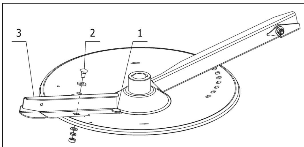
1, 2 – Болт; 3 – Лопатка
