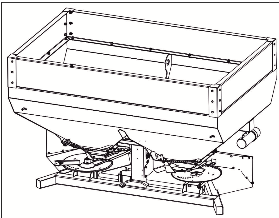
Рисунок 1.1 – Разбрасыватель минеральных удобрений РА-1000 «Grach»
