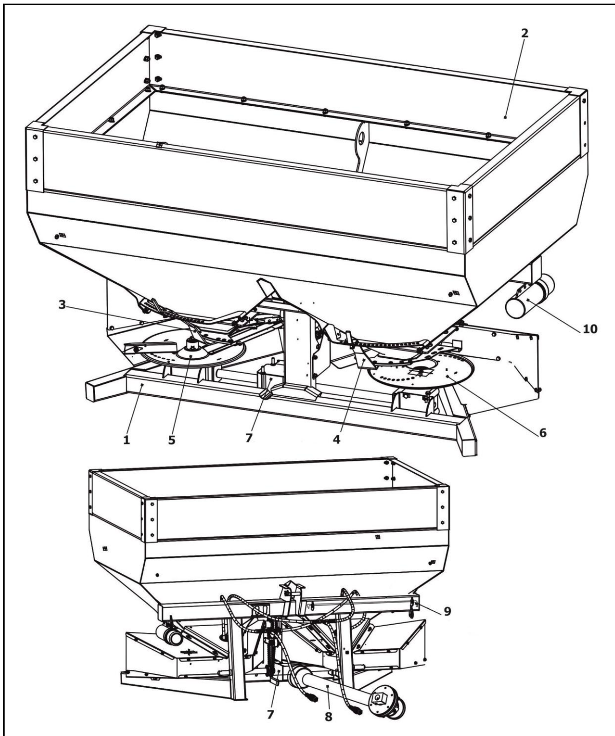
Рисунок 3.1 – Состав разбрасывателя
