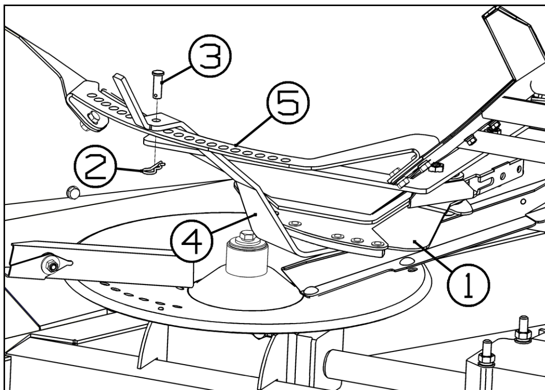
1 – Запорная заслонка; 2 – Шплинт; 3 – Ось; 4 – Регулировочный рычаг дозирующей заслонки; 5 – Шкала (кронштейн) Рисунок 5.8 – Настройка положения дозирующей заслонки с помощью регулировочного рычага
