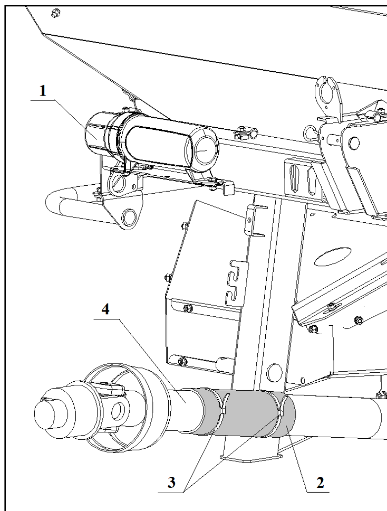
1 – Тубус; 2 – Пакет с документацией; 3 – Кабельные стяжки; 4 – Карданный вал Рисунок 1.2 – Место размещения тубуса с документацией
