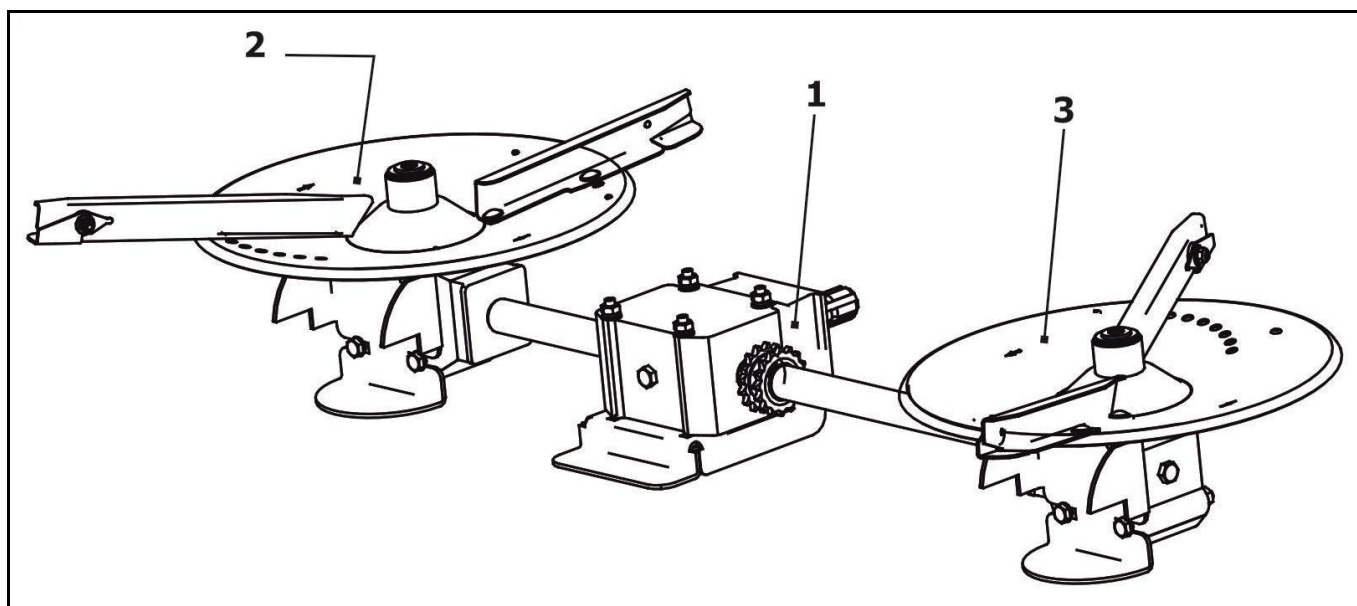
1 – Редуктор; 2, 3 – Разбрасывающие диски Рисунок 3.5 – Распределяющее устройство
