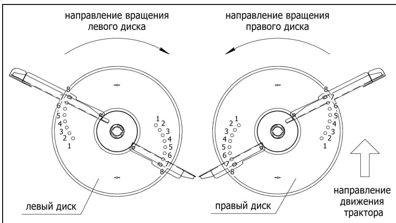
Рисунок 5.1 – Схема установки лопаток
