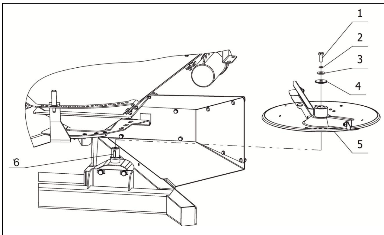
1 – Болт; 2 – Гайка; 3, 4 – Шайба; 5 – Разбрасывающий диск; 6 – Шпонка
