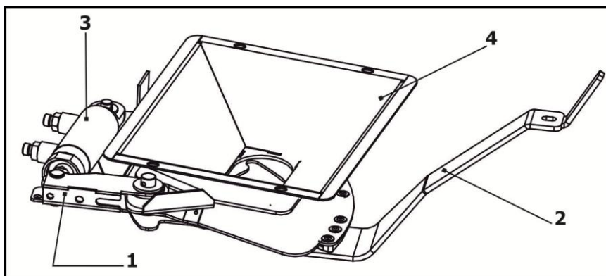
1 – Заслонка запорная; 2 – Заслонка дозирующая; 3 – Гидроцилиндр; 4 – Проставка
