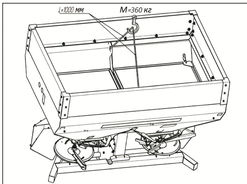
Рисунок 7.1 – Схема строповки
