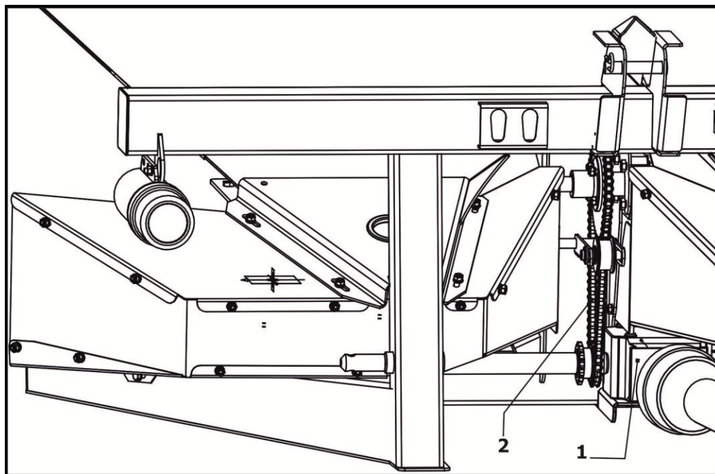
1 – Редуктор; 2 – Цепная передача
