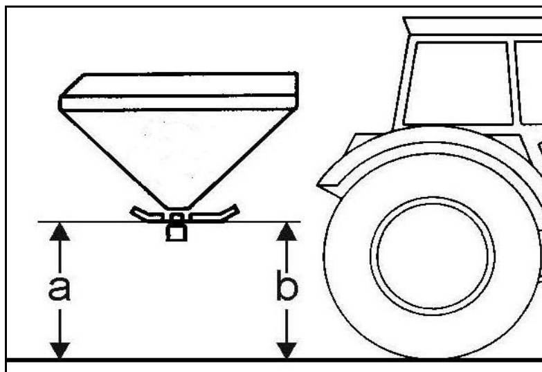
Рисунок 5.4 – Высота над поверхностью поля при стандартном удобрении
