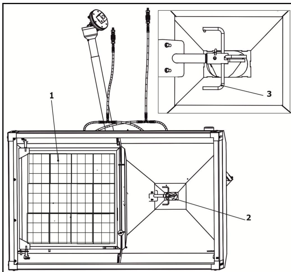
1 – Решетка; 2 – Ворошилка; 3 – Лопасть Рисунок 3.2 – Бункер. Вид сверху
