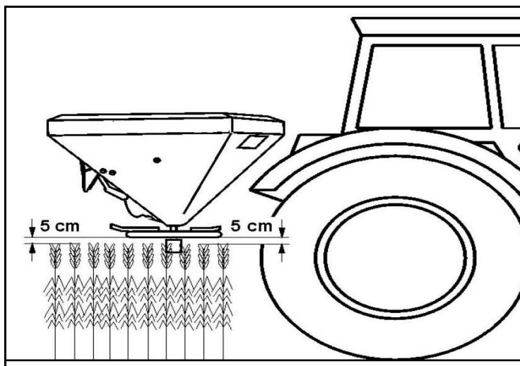
Рисунок 5.5 – Высота над поверхностью поля при позднем внесении удобрения
