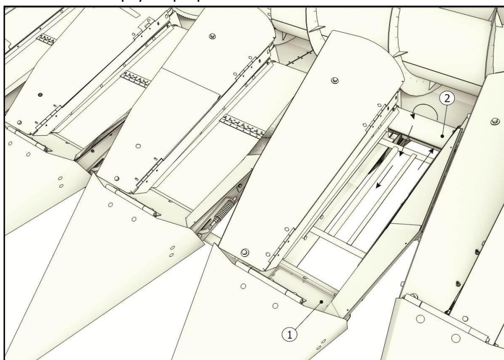
1 – Валик ведомый ПСХ 01.500; 2 – Валик ведущий ПСХ 01.480 Рисунок 6.14
