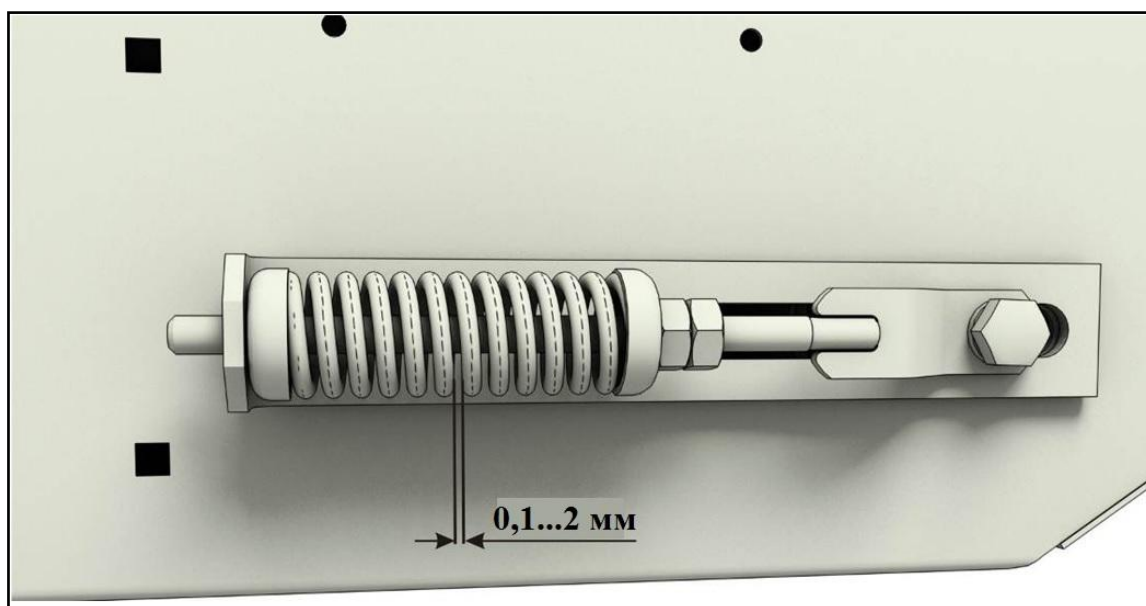
Рисунок 2.15 – Контроль натяжения лент транспортеров семян
