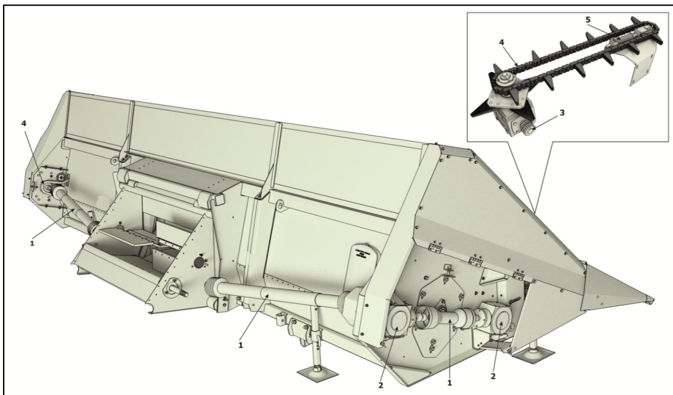
Рисунок 8.1 – Места смазки приспособления
