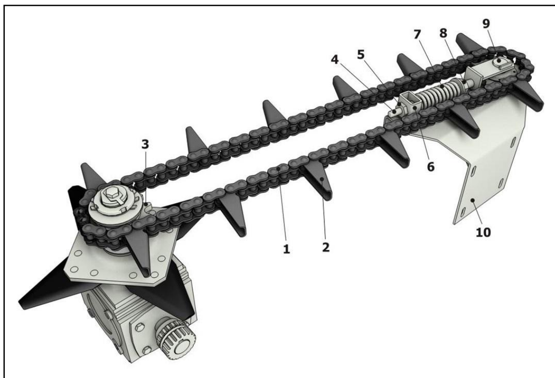
Рисунок 2.11 – Транспортер стеблей
