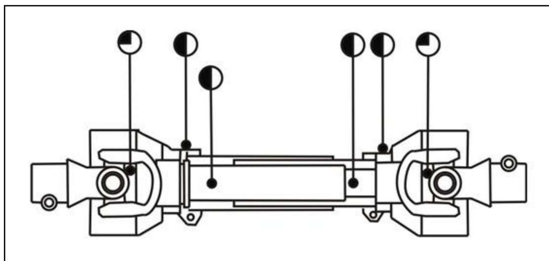
Рисунок 8.2 – Места и периодичность смазки карданного вала
