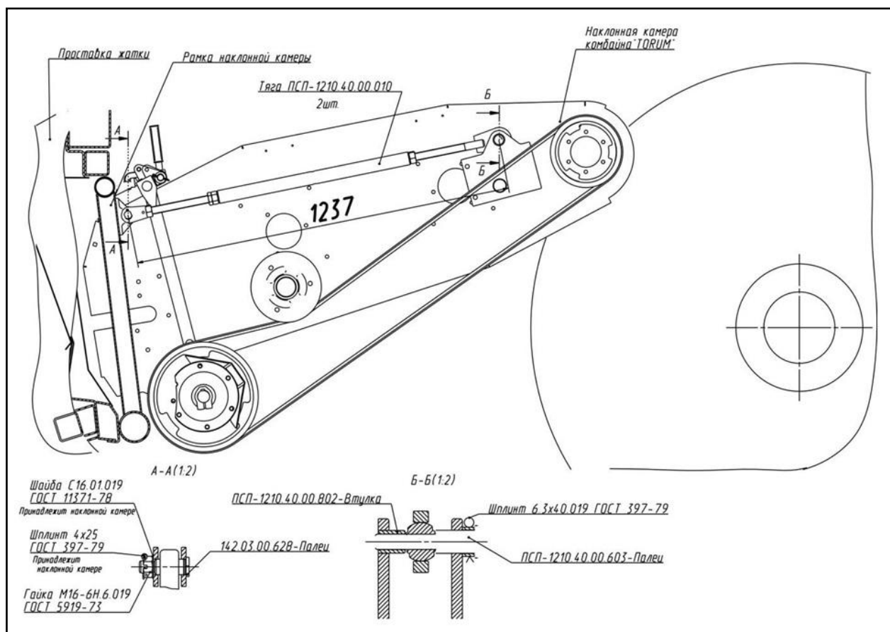
Рисунок 6.8 – Установка тяг на наклонную камеру комбайна «TORUM»
