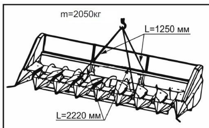
Рисунок 9.1 – Схема строповки
