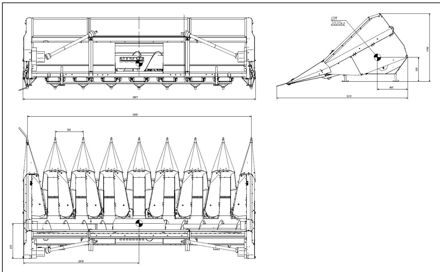
Рисунок Г.1 – Габаритные размеры приспособления и расположение центра масс
