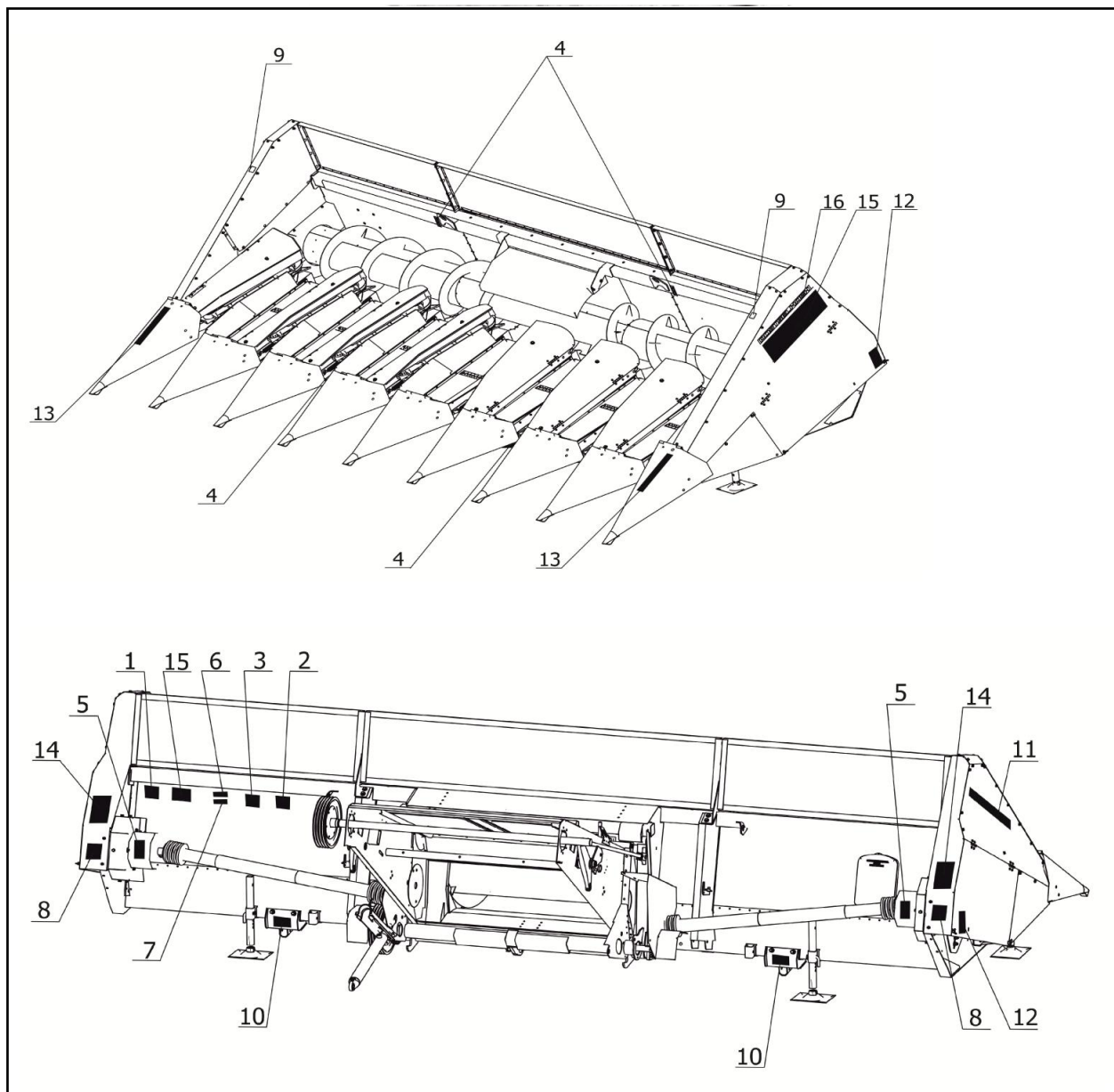
Рисунок 4.1 – Месторасположение табличек и аппликаций
