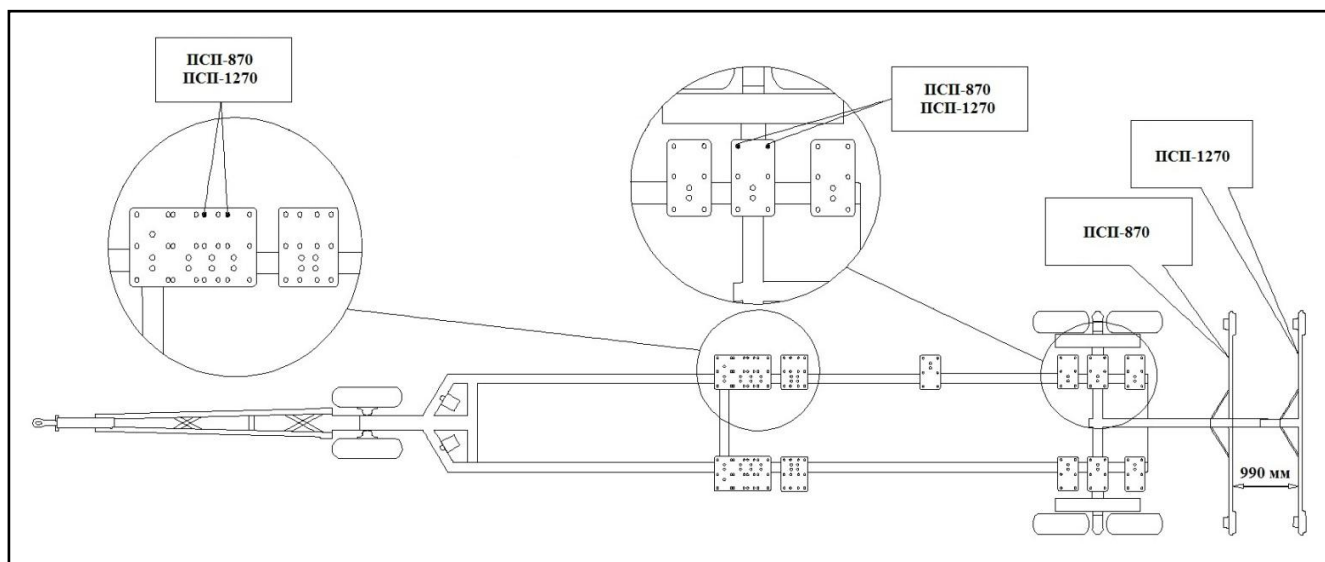
Рисунок 9.3 – Установка опор приспособления ПСП-870
