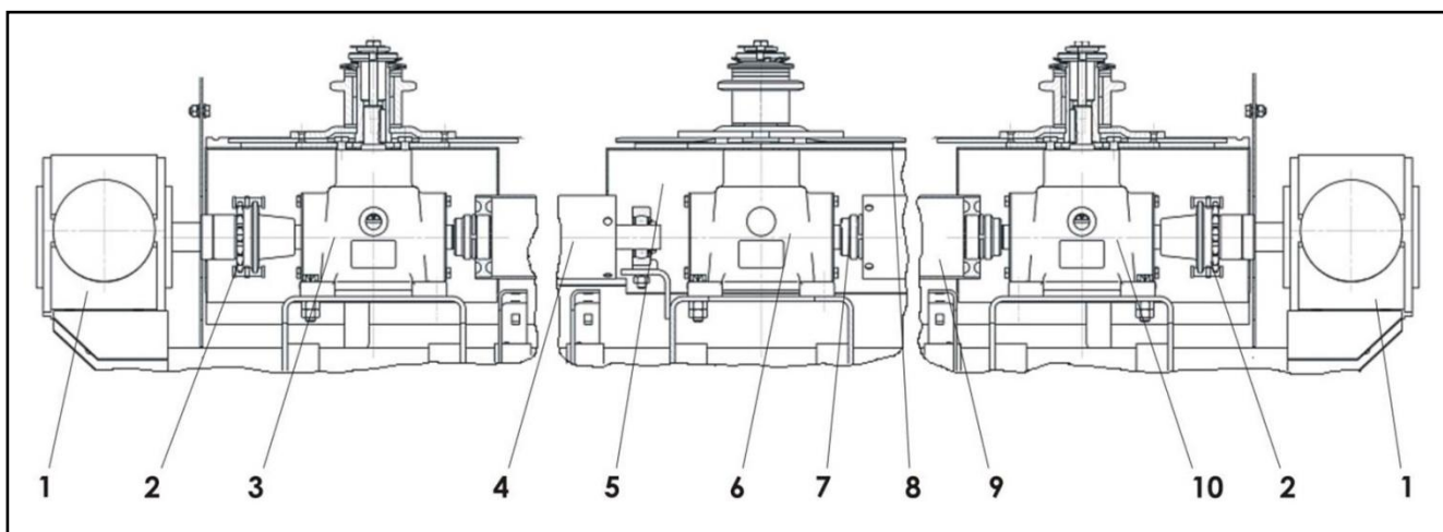
Рисунок 2.16 – Привод конических редукторов
