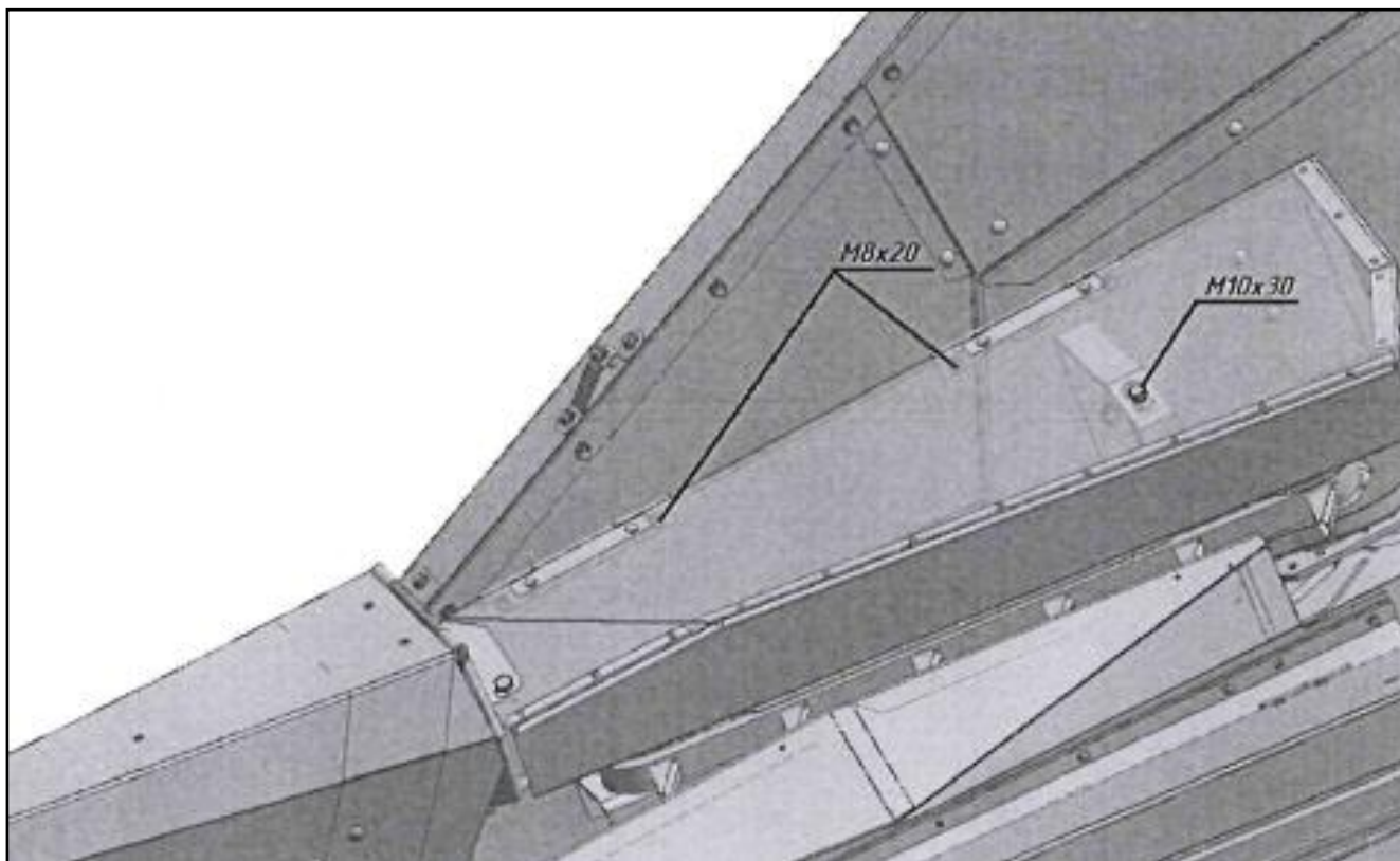
Рисунок 2.7 – Демонтаж скатов
