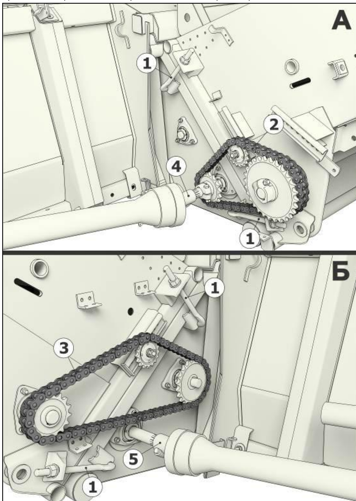
Рисунок 6.5 – Навешивание ПСП-870-03/-39 на комбайн
