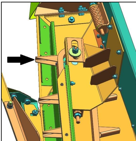
Рисунок 2.3 – Транспортер стеблей
