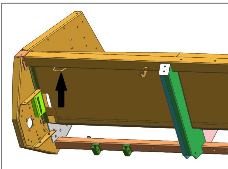
Рисунок 2.2 – Хомут
