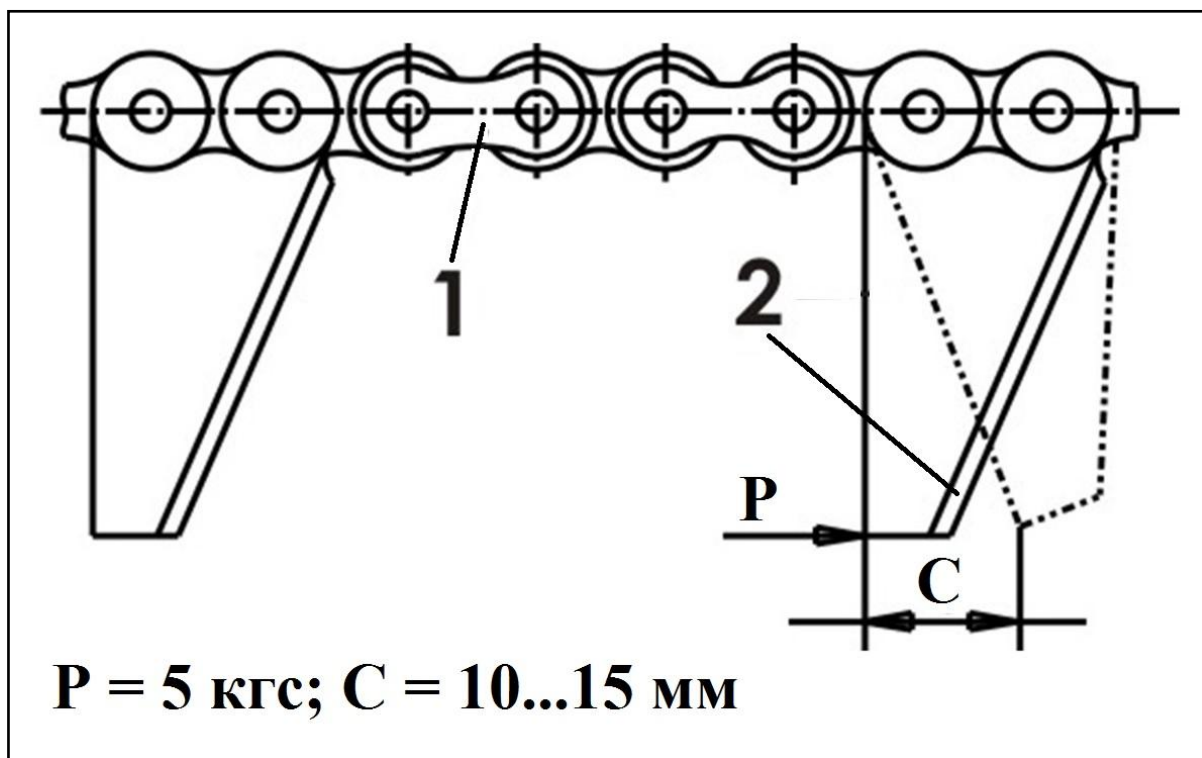
Рисунок 2.13 – Контроль натяжения транспортеров стеблей
