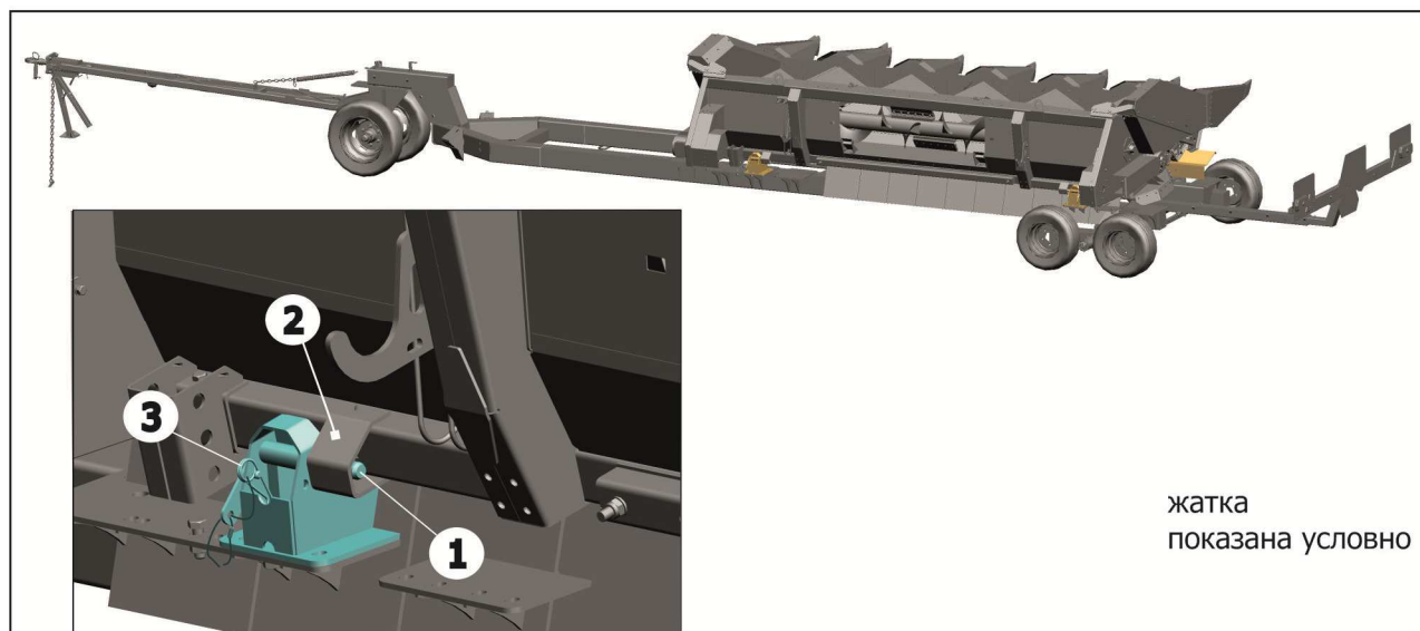
1 - Фиксатор опор; 2 – Опора жатки; 3 - Шплинт Рисунок 9.3
