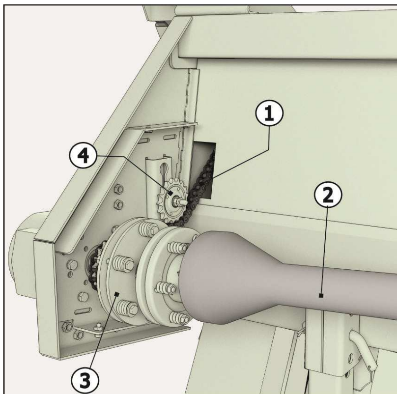
1 – Цепная передача; 2 – Карданный вал; 3 - Предохранительная фрикционная муфта; 4 - Натяжная звездочка; Рисунок 2.7 – Привод шнека
