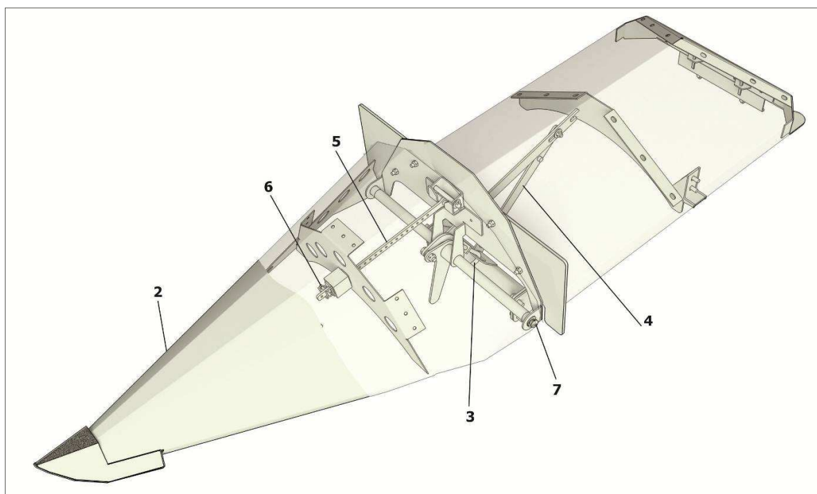
1 – Капот; 2 - Делитель; 3 - Зацеп; 4 – Опора; 5 - Фиксатор; 5 - Шплинт; 7 - Шарнир
