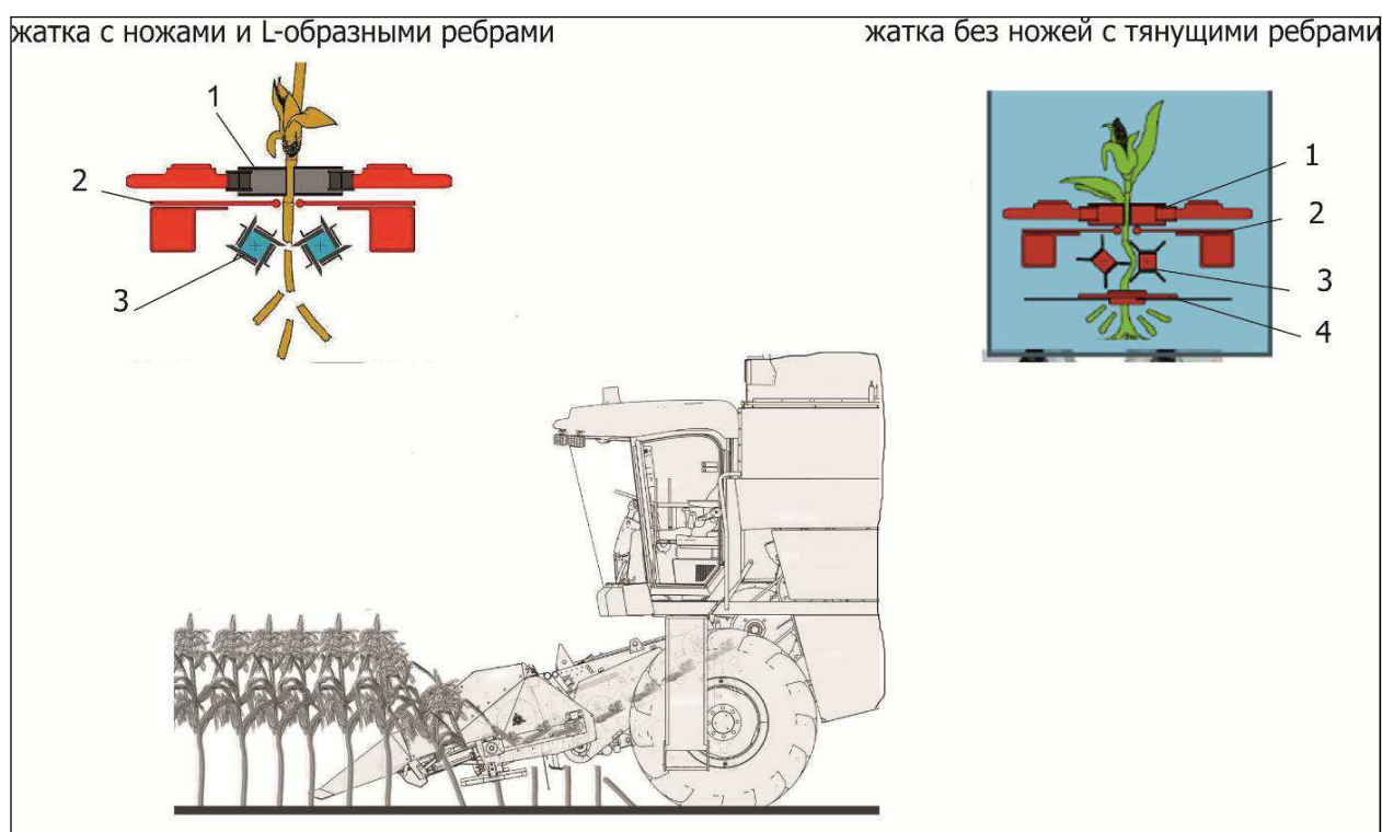
1 - Подающая цепь; 2 - Отрывная пластина; 3 - Протягивающий валец; 4 - Измельчающий аппарат Рисунок 2.13 – Технологическая схема работы приспособления
