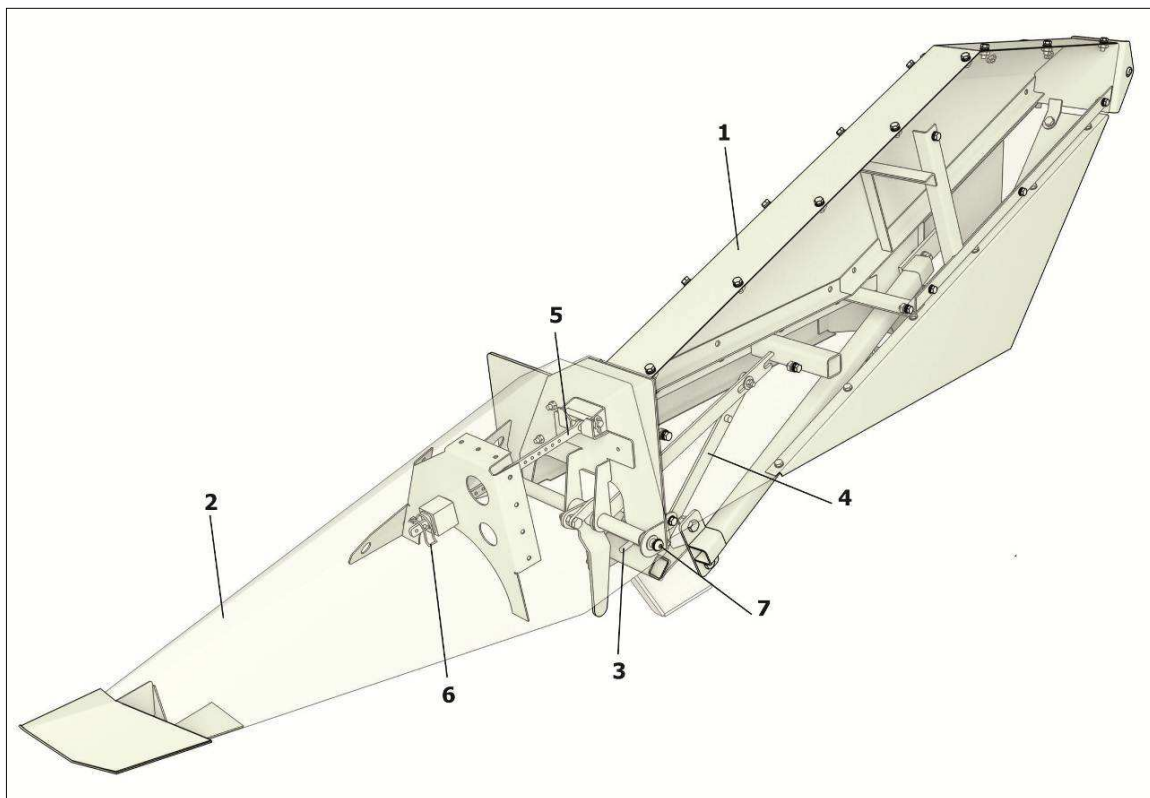
1 – Капот; 2 - Делитель; 3 - Зацеп; 4 – Опора; 5 - Фиксатор; 5 - Шплинт; 7 - Шарнир
