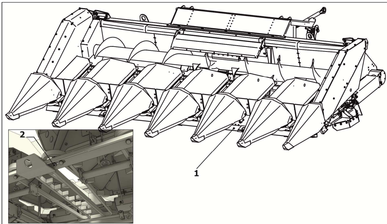
1 – Траверса; 2 - Болтокрепеж
