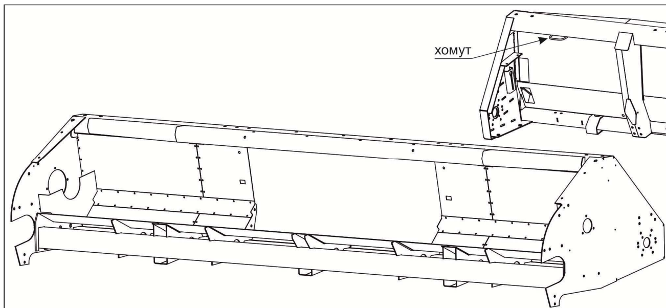
Рисунок 2.2 – Каркас жатки
