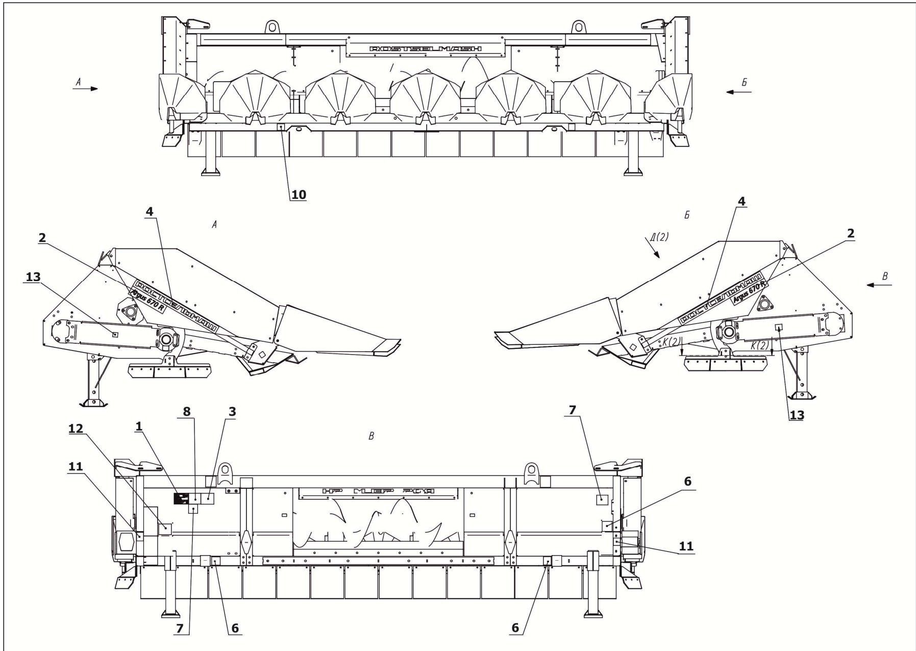
Рисунок 4.1 – Схема расположения табличек и аппликаций на приспособлении
