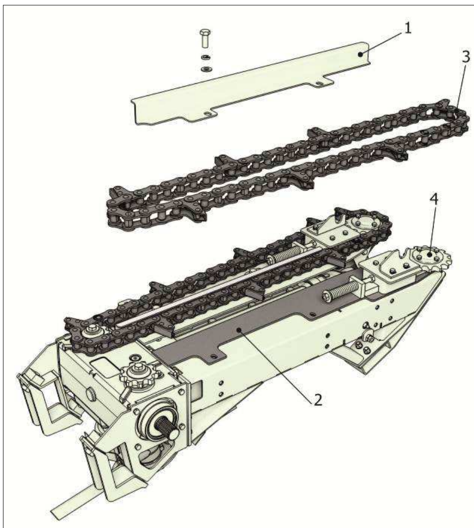
1 - Успокоитель ППК-870.01.06.431-01; 2 - Неподвижная пластина ППК-870.01.06.422; 3 – Цепь; 4 - Натяжник
