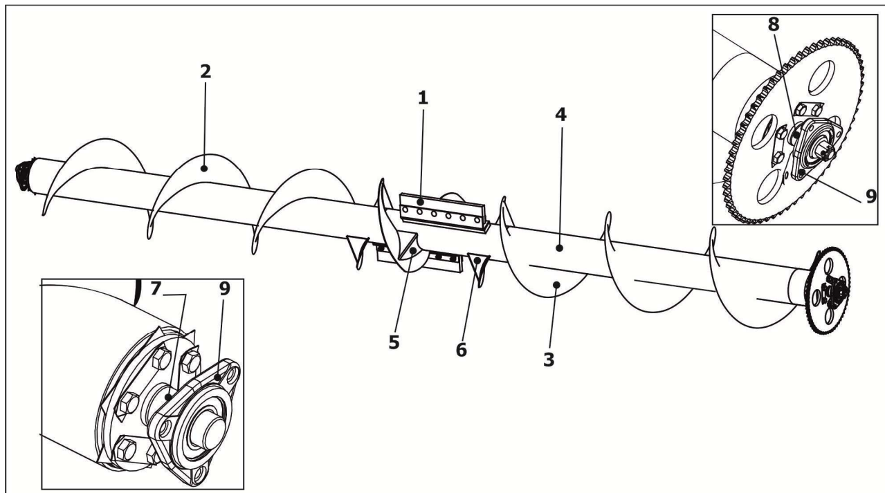
1 - Лопасть; 2 - Спираль правая; 3 - Спираль левая; 4 - Труба шнека; 5 - Виток правый; 6 - Виток левый; 7 - Цапфа с фланцем; 9 - Цапфа со звездочкой; 10 - Подшипниковая опора Рисунок 2.6 – Шнек
