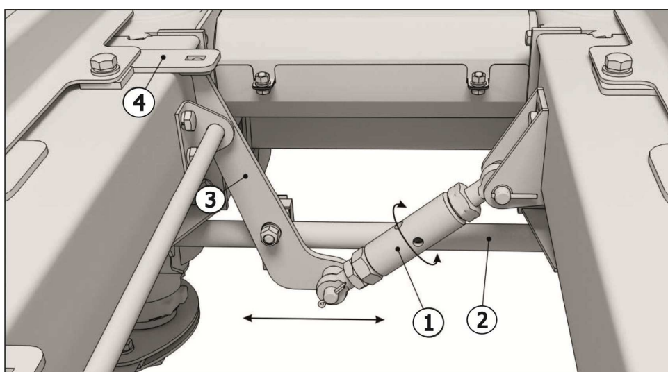
1 - Тяга; 2 - Штанга; 3 - Поводок; 4 - Отрывная пластина Рисунок 7.3 - Механическая регулировка отрывных пластин русла
