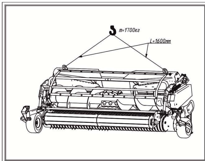
Рисунок 8.1 – Схема строповки
