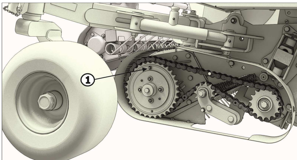
1 – Срезной болт
