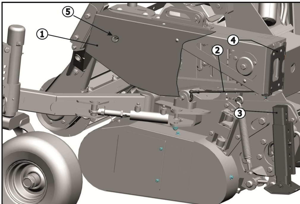
1 – Щиток; 2 – Тяга; 3 – Опора; 4 – Петли; 5 – Замок Рисунок 6.17
