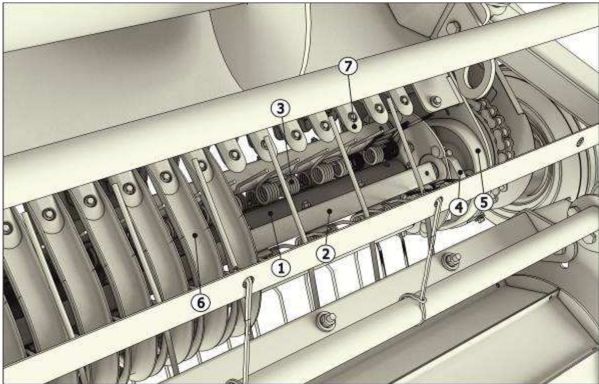
1 – Вал; 2 – Держатель; 3 – Палец подбирающий; 4 – Эксцентрик; 5 – Дорожка беговая; 6 – Скот; 7 – Каркас
