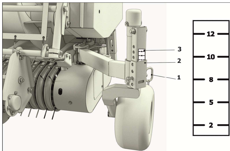
1 – Фиксатор; 2 – Кронштейн; 3 – Табличка «Высота подбора» Рисунок 6.6
