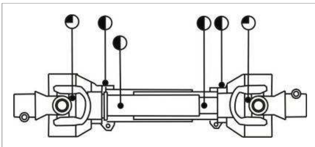
Рисунок 7.1 – Места смазки карданного вала
