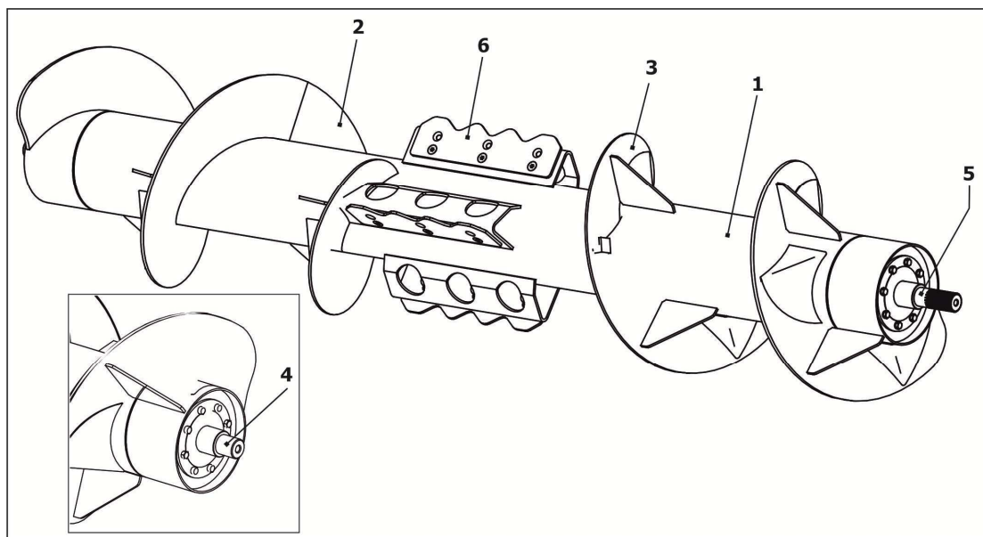
1 – Труба шнека; 2 – Правая лента; 3 – Левая лента; 4, 5 – Цапфа; 6 – Лопатка Рисунок 2.5 – Шнек
