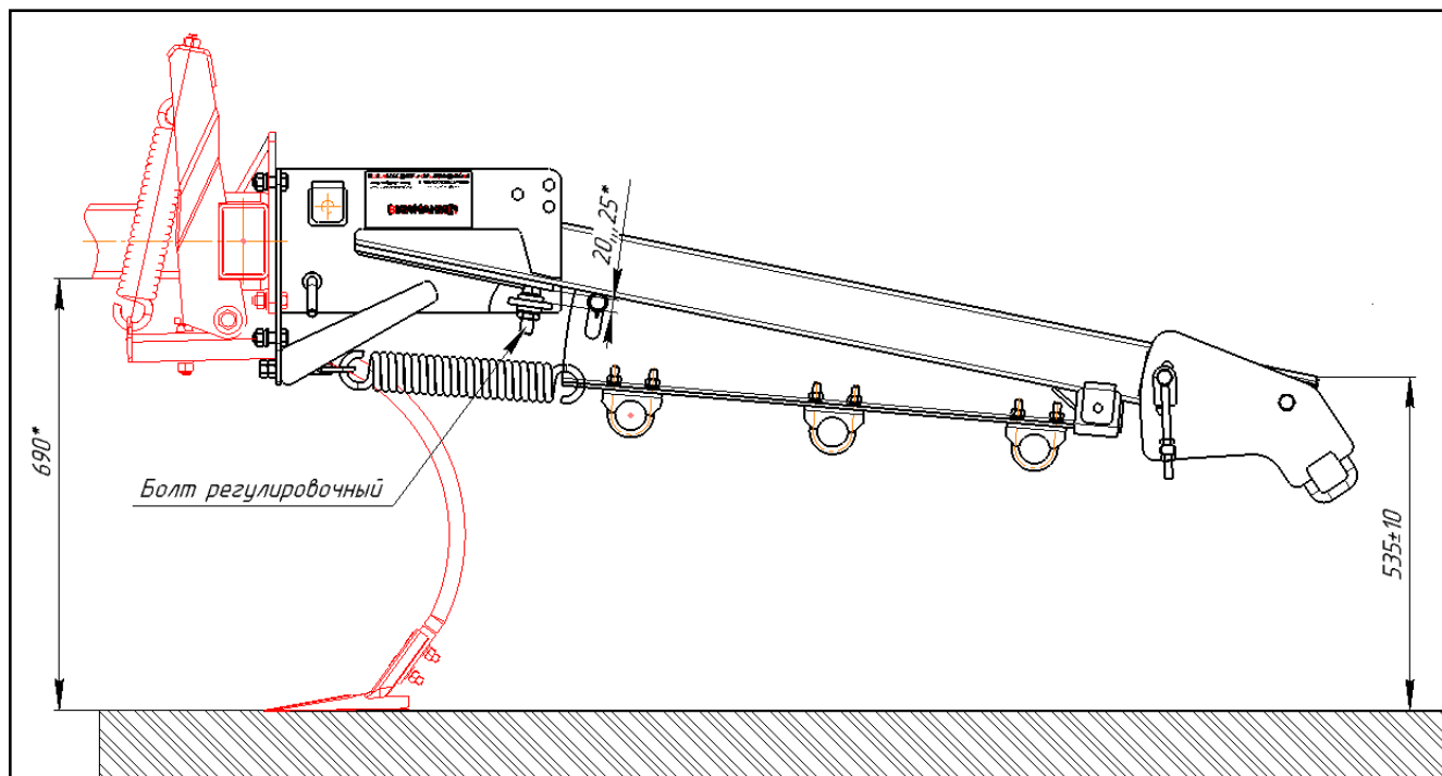
Рисунок 20.1 – Установка подвесок комбинированного шлейфа
