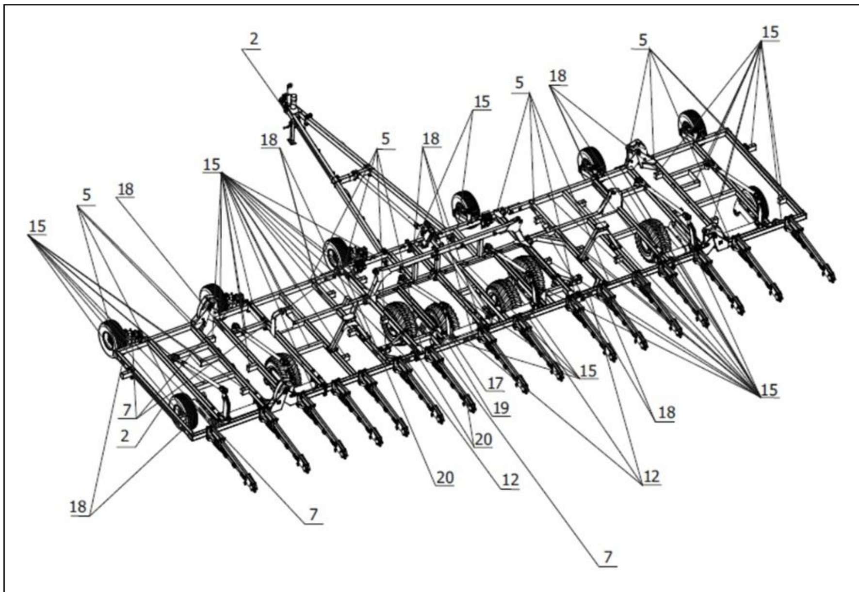
Рисунок 19.2 – Месторасположение табличек на культиваторах К-14800 и К-14800-01. Вид сзади слева
