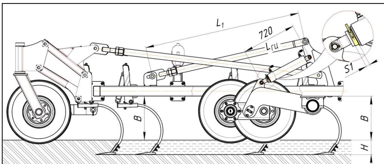
Рисунок 20.3 – Первичная регулировка глубины обработки
