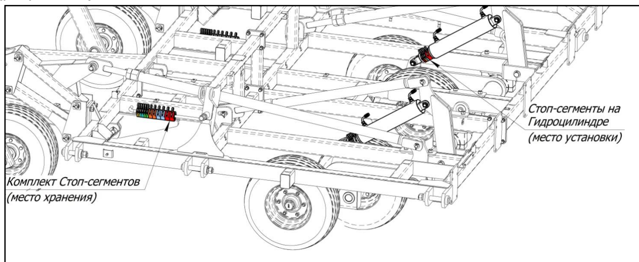
Рисунок 7.2 – Места хранения и установки стоп-сегментов
