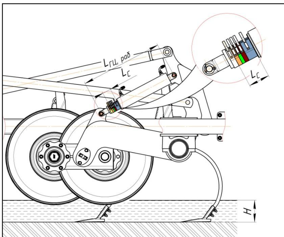
Рисунок 20.5 – Регулировка глубины обработки
