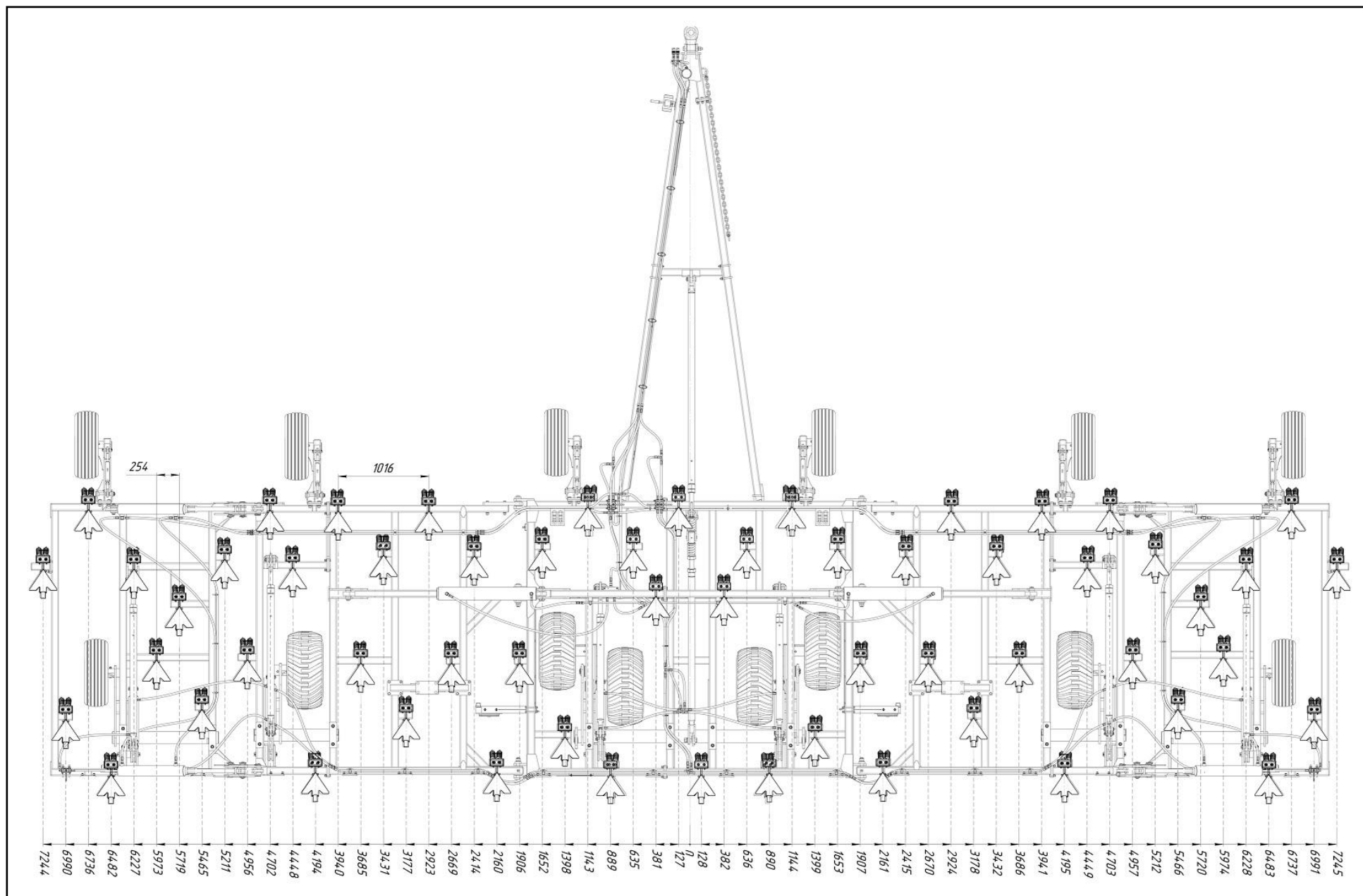
Рисунок Б.2 – Схема расстановки рабочих органов культиватора К-14800 и К-14800-01
