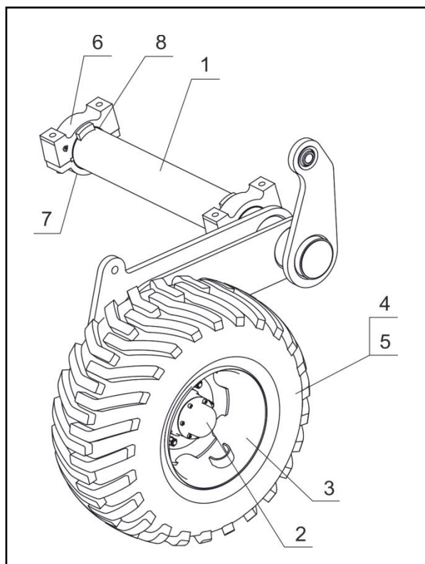
Рисунок 10 – Шасси крыла
