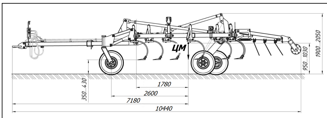
Рисунок Ж.1 – Схема расположения центра масс культиваторов в транспортном положении
