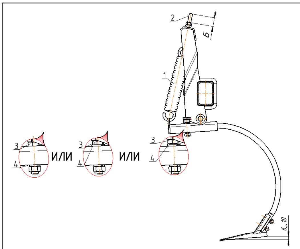
1 – Пружина; 2 – Натяжитель; 3 – Болт М16×70; 4 – Шайба 16 Рисунок 23.1 – Регулировка степени натяжения пружин
