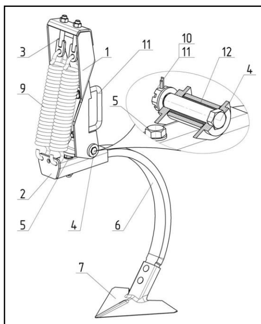
Рисунок 14 – Рабочий орган
