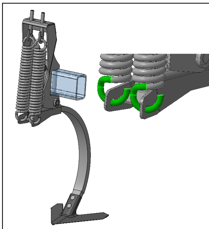
Рисунок 23.2 – Установка пружин и натяжителей подвески рабочего органа
