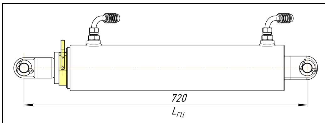
Рисунок 7.3 – Гидроцилиндр MC100/50x400-20.404A.OAOA.720.01.G(052) в сложенном положении.
