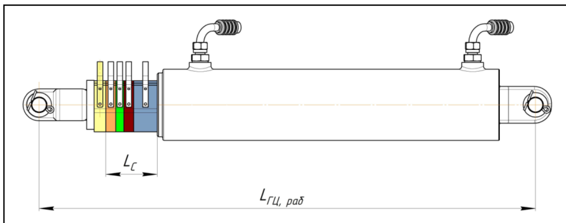
Рисунок 20.4 – Установка стоп-сегментов на шток гидроцилиндра шасси
